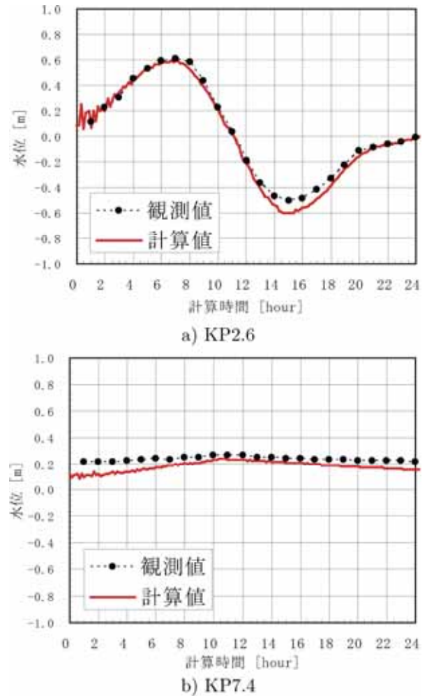
図 - 27 水位の観測地と計算値
