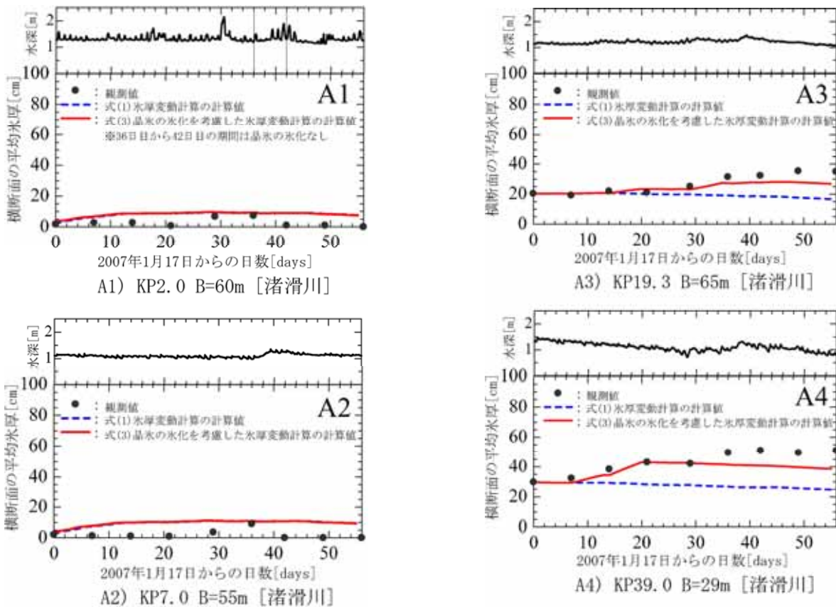
図 - 47 渚滑川における氷厚の観測値と計算値
