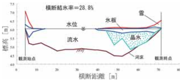
図 - 37 横断測量の一例(2007/2/27、中湧別観測所B1)
