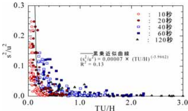
図 - 12 各測定時間と平均流速の関係図(天塩川・結氷時)
