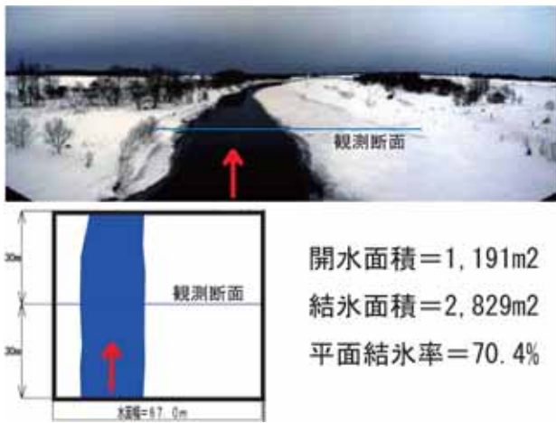
図 - 36 平面結氷率の算出の一例(2007/2/27、中湧別観測所 B1)
