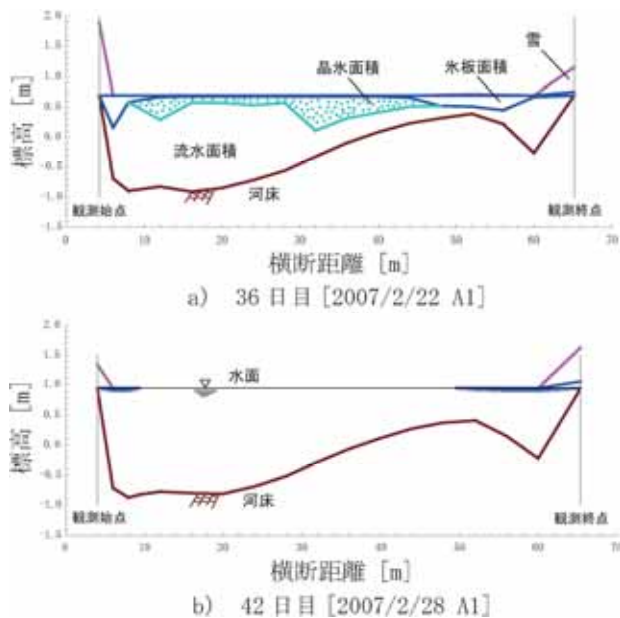
図 - 48 横断測量図A1渚滑橋観測所
