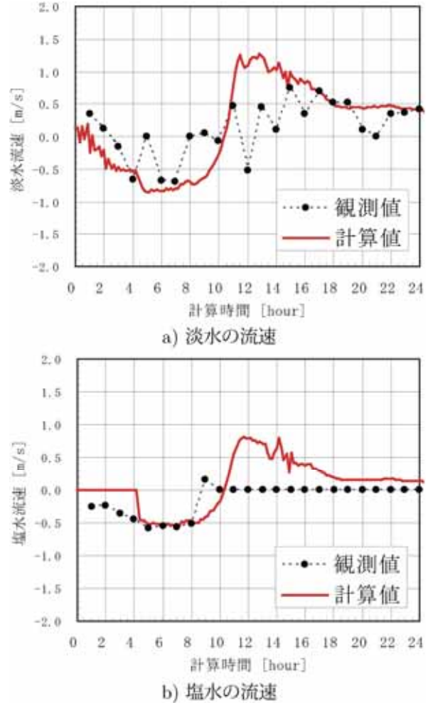
図 - 28 淡水流速と塩水流速の観測値と計算値(KP2.0)
