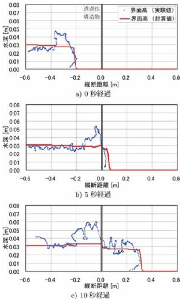
図 - 25 界面の実験値と計算値(構造物あり)
