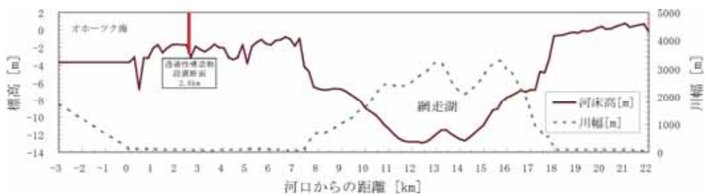
図 - 26 数値計算の河道条件[河床高、川幅]
