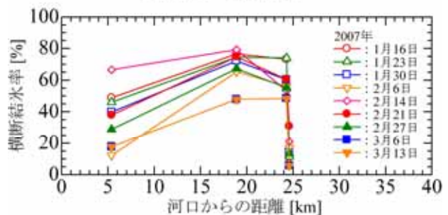
図 - 38 河川縦断方向の結氷率
