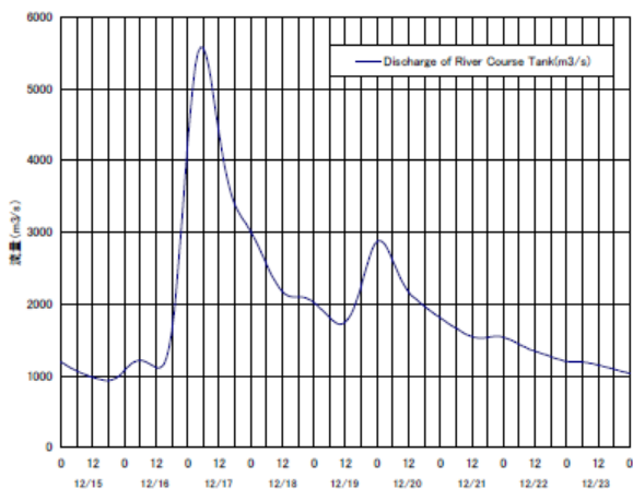
図3 2007.12 洪水波形図 (IFAS による計算値)
