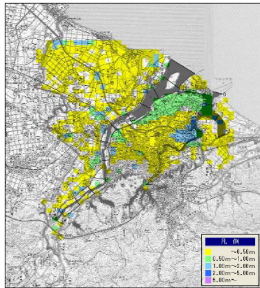
図 10 水理公式集例題プログラムによる計算
