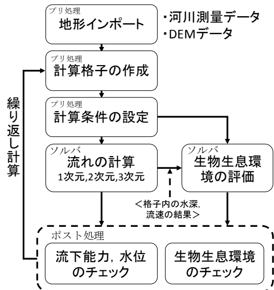
図-2 評価ツールの概略
