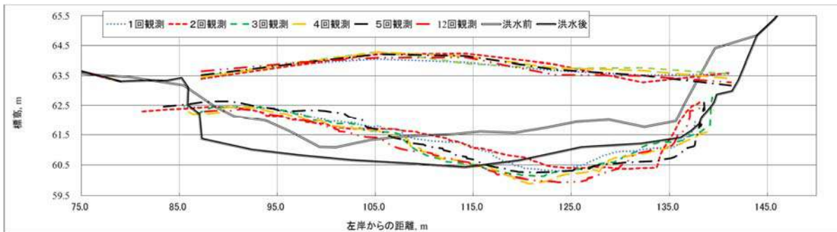
平成25年10月16日洪水の洪水中の河床高変化
