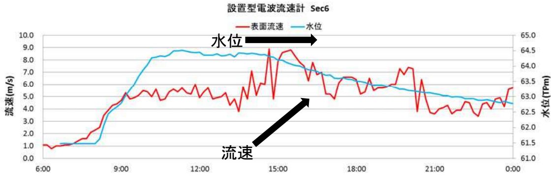
平成25年9月16日洪水の表面流速及び水位(観測)
