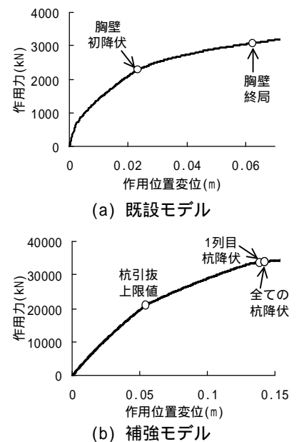
図-2 衝突位置の水平力-変位関係
