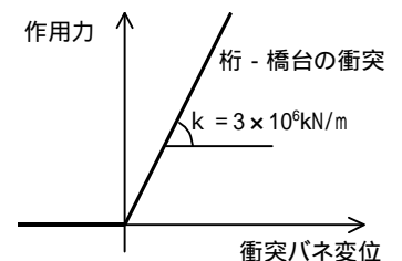
図-3 衝突バネ
