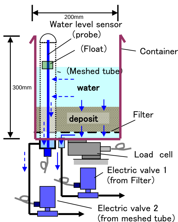
自動降灰・降雨量計の機器構成
