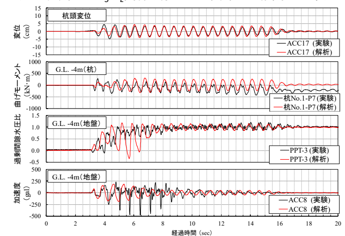
遠心力模型実験の再現解析結果(場所打ち杭の例)
