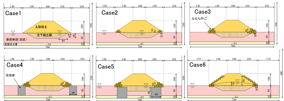
各種対策を施した動的遠心模型実験断面
