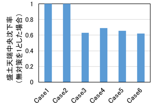
法尻へ集中的なふとんかご工(4段以上)を施すことで盛土沈下量を抑制可能
