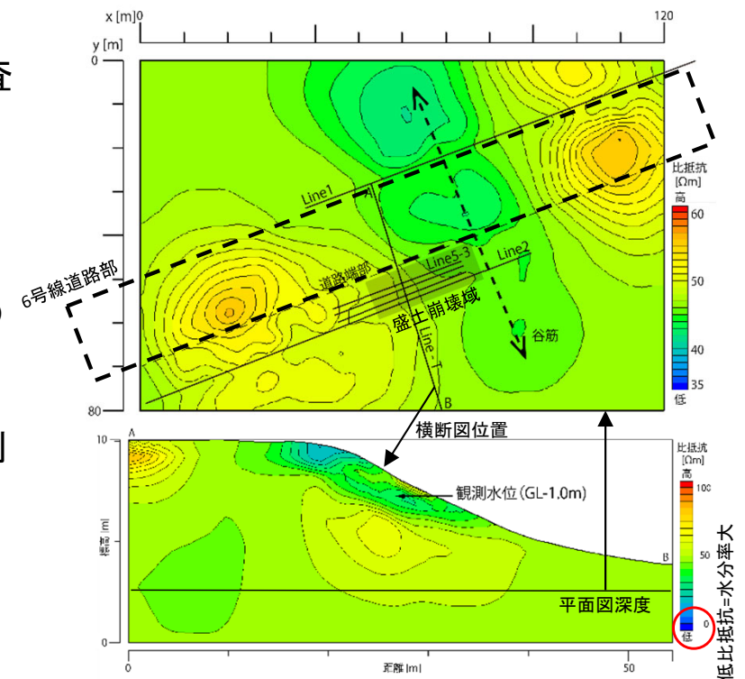
崩壊被災盛土における3次元電気比抵抗分布の 平面分布(上)と垂直分布(下)
