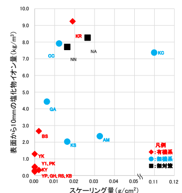
図-6 凍結融解試験後の塩化物イオン量とスケーリング量の関係
