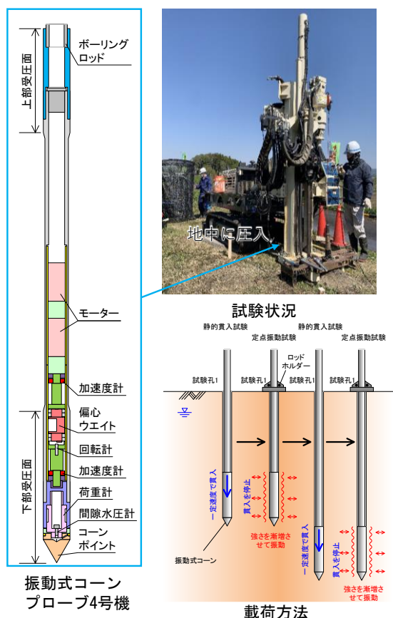
図-1 振動式コーン試験法の概要
