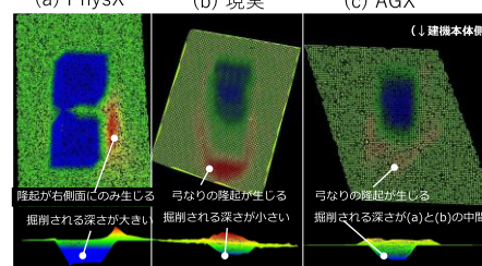
油圧ショベルによる掘削形状のシミュレータ結果と実計測の比較検証
