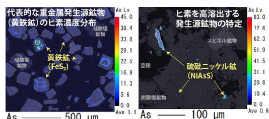
図-4 電子顕微鏡分析による重金属等溶出源鉱物の同定とヒ素含有形態の判別
