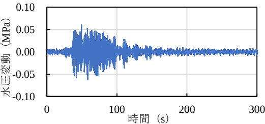
図-5 農業用管水路において観測された地震時動水圧データ
