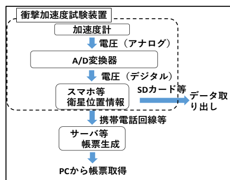
図-3 デジタイゼーションシステム系統概要図
