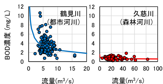
図-3 過去10年間の水文水質DBを用いて作成した都市・森林河川の流量とBOD濃度の関係
