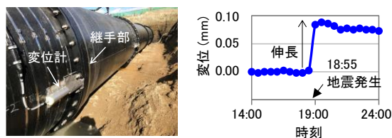
図-4 変位計の設置状況および変位計の観測データ
