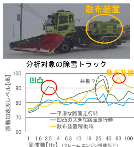
図-2 除雪トラックの周波数分析
