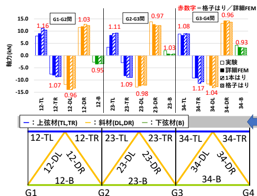
図-4 対傾構の軸力比較
