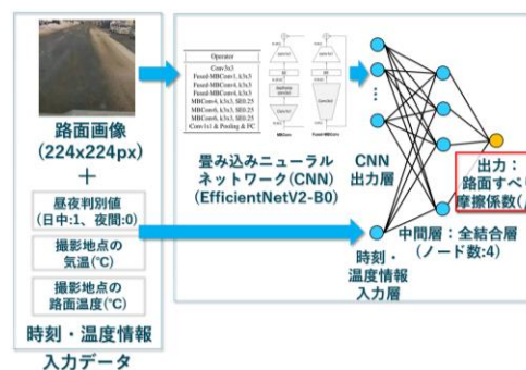
図-1 マルチモーダル AI による路面すべり摩擦係数推定方法の概要
