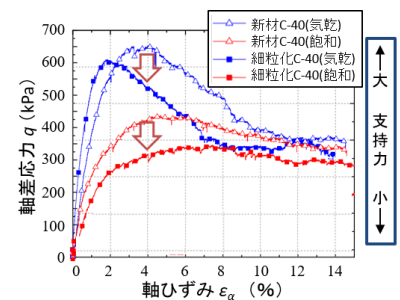
図-4 支持力試験の結果
