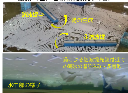
図-7 大型平面水槽を用いた海水をとまなう津波(孤立波)の模型実験
