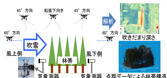
図-6 LiDAR UAVや気象測器を活用した林帯観測(左)と解析結果例(右)
