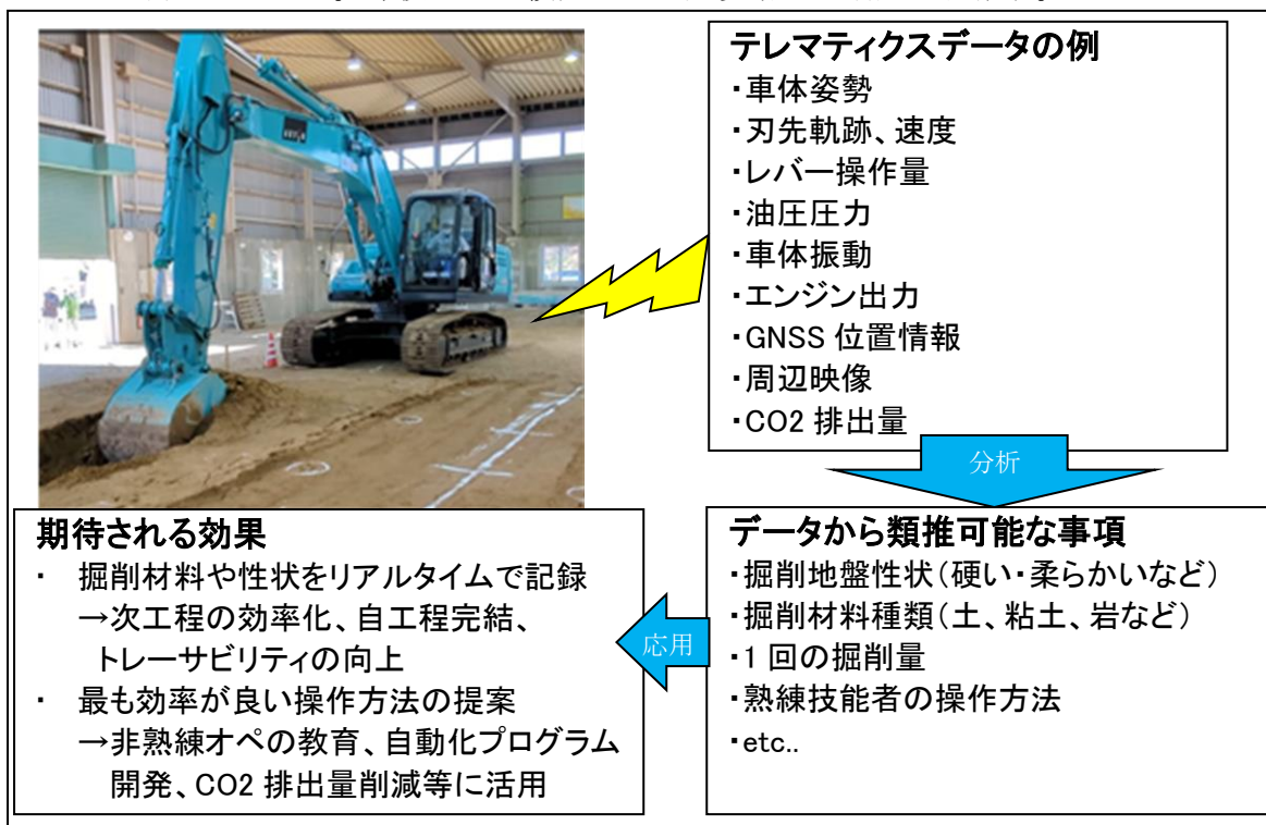
図-1 油圧ショベルのデータ収集システムの活用と期待される効果
