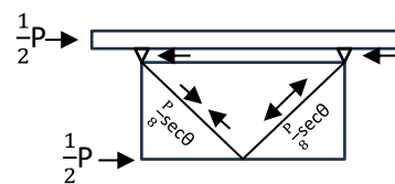
図-2 現行設計のイメージ (対傾構)
