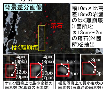
図-3 落石発生の危険がある道路斜面における背景差分画像例と 変状抽出時の画素数例
