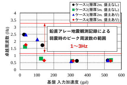
図-5 泥炭地盤基盤の入力加速度と卓越周波数の関係
