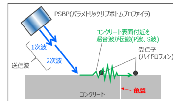
コンクリート水中部亀裂調査技術概要
