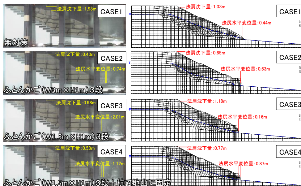
図-1 「ふとんかご」によるのり尻補強対策を行った実験と数値計算結果
