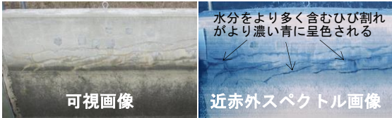
図-4 補修後の開水路における可視画像と近赤外スペクトル画像の比較
