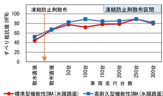
図-5 路面すべり摩擦抵抗の比較
