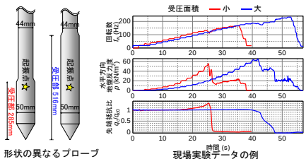
図-8 原位置液状化試験法に用いる試験装置の改良効果の検証
