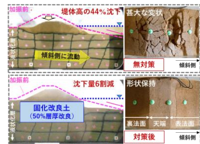
図-7 低コスト液状化対策技術に関する遠心模型実験(左:側面図、右:上面図)
