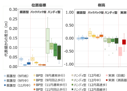
図-2 LiDAR 機器による街路樹の計測精度の比較
