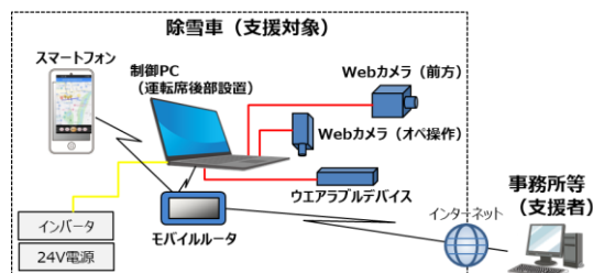
図-2 除雪等機械オペレータ支援システム(システム構成図)
