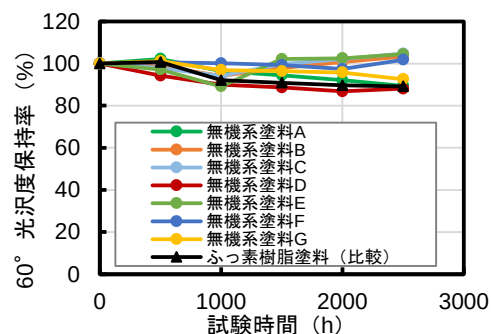
図-6 促進耐候性試験(キセノンランプ法)における無機系塗料の光沢度保持率の経時変化
