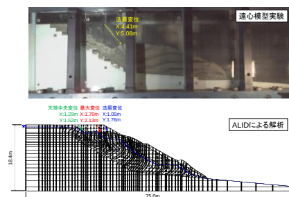
図-4 細粒分を含む谷埋め高盛土の自重変形解析
