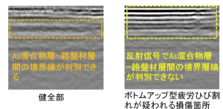
図-6 舗装体の損傷による内部画像の差異
