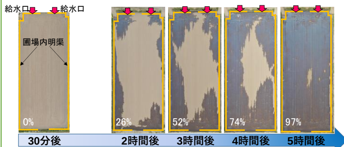
図-4 圃場内明渠を用いた灌漑時の水足進行
