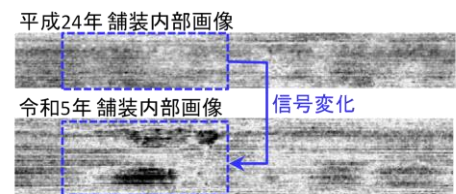
図-5 電磁波レーダ画像の経年変化
