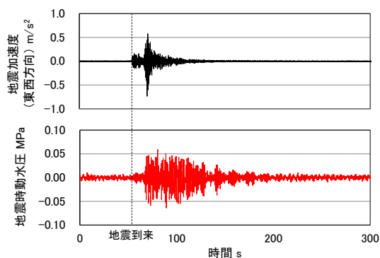
図-3 地震加速度と地震時動水圧の観測データ
