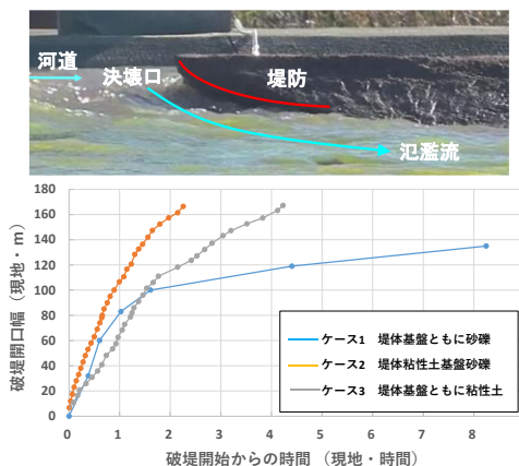
図-6 堤防決壊の縮尺模型実験の状況(上)及び実験ケースごとの破堤口拡幅の進行速度(下)
