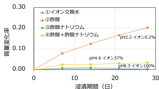
同一mol濃度における質量変化率
