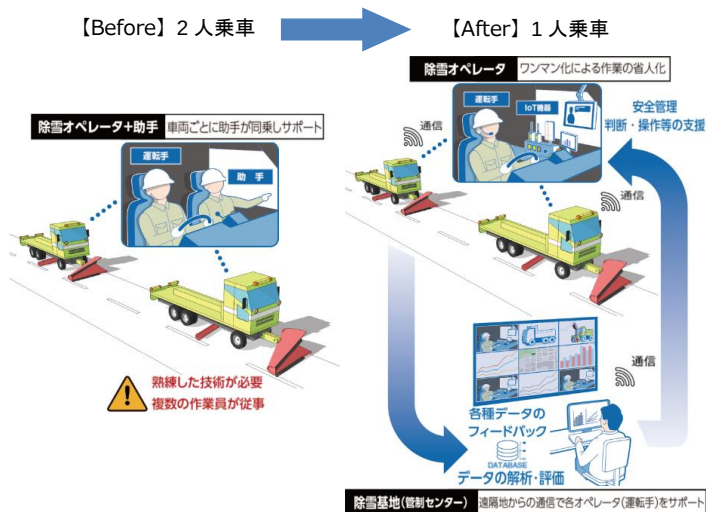
図-1 除雪機械オペレータ作業・安全運転支援システム設計
