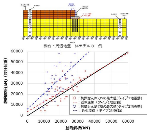
図-2 地震時に橋台に作用する力のうち杭頭せん断力の例
