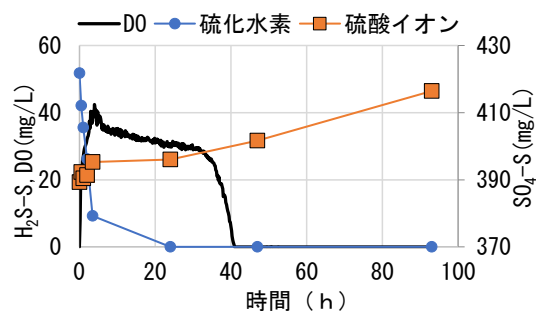
図-6 硫化水素含有水の酸素供給後の硫黄の形態別追跡結果
