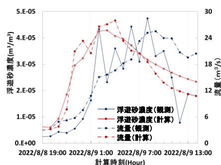
図-4 流量、浮遊砂濃度について、観測と解析結果の比較(安平川)
