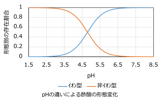
pHの違いによる酢酸の形態変化
