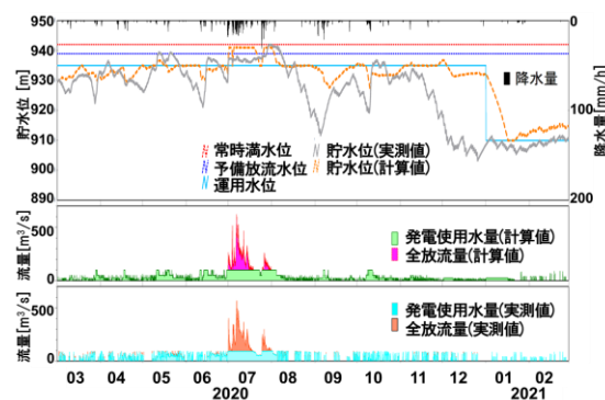
図-3 年間を通したダム操作ミュレーション事例(水位、使用水量、放流量)
