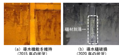
図-5 トンネル覆工の漏水対策工不具合事例
