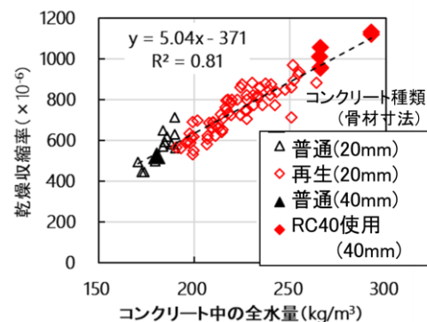
図-3 コンクリートの乾燥収縮(骨材種類によらずコンクリート中の全水量と対応)
