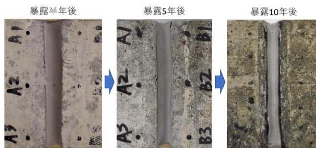
図-2 有機系充填材の劣化進行の一例（増毛暴露場） (紫外線劣化等で亀裂が発生→徐々に剥離が拡大)
