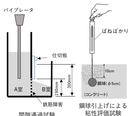
図-1 高流動性コンクリートの特性を評価する試験例
