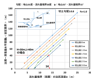
図-4 地山条件に応じたチャート図の例(安定確保可能な流れ盤条件)
