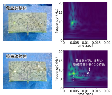
打音波形の時間周波数解析結果の例 (左:試験体の損傷状態、右:解析結果)
