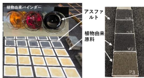
図-1 植物由来の舗装用代替材料の屋外暴露例
