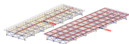
(a) 一本梁モデル (b) 格子梁モデル
