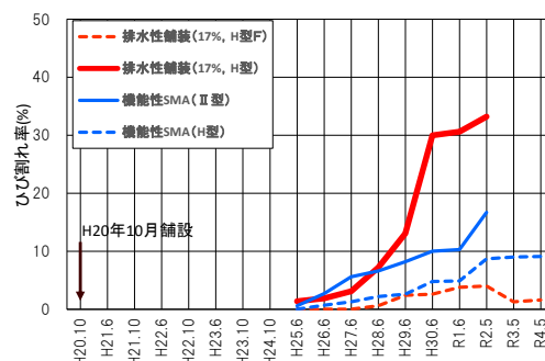
図-4 ひび割れ率の測定結果の比較試験
