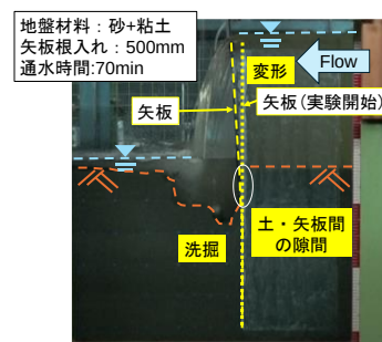
図-5 堤防強化工法の水理模型実験の状況
