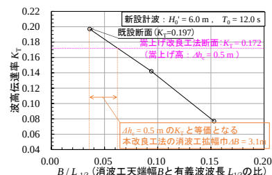
B/L_{1/3} と波高伝達率 K_T の関係
