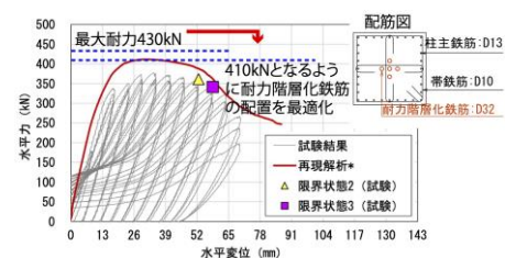
図-3 荷重変位（橋脚天端）関係
