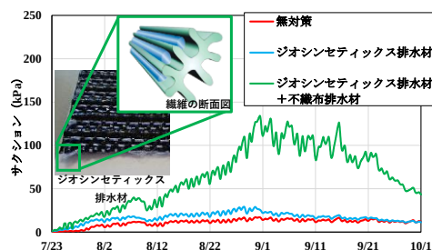
図-7 排水材の排水能力
