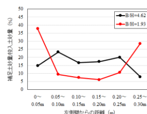
図-5 横断方向の通過土砂分布
