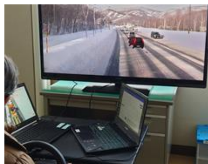
写真-1 除雪機械シミュレータの試作品
