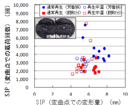
図-2 再生中温化アスファルト混合物の剥離抵抗性
