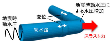
図-2 曲管部におけるスラスト力の発生と管体変位の模式
