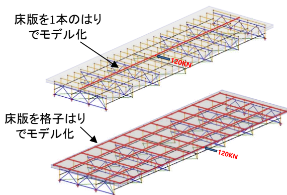
図-3 提案する立体骨組モデル
