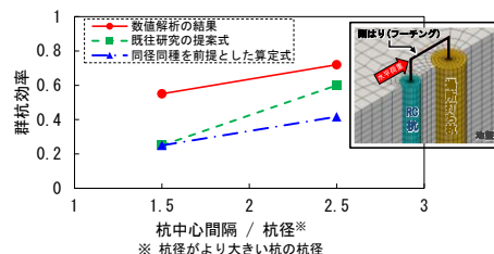
図-1 各種の群杭効率の比較
