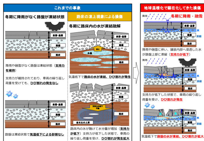
図-3 冬期間の舗装損傷において顕在化してきた事象
