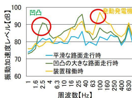
図-3 外乱、装置毎の周波数特性例
