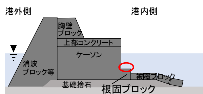
図-1 防波堤の根固ブロック上の試験体設置位置
