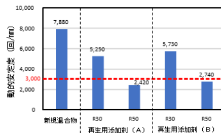
図-1 再生アスファルト混合物の塑性変形抵抗性
