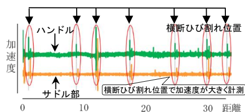
図-5 加速度計測データの一例
