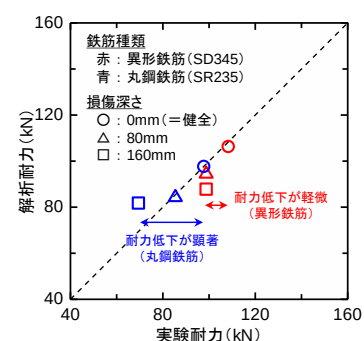
図-1 耐力低下の評価結果
