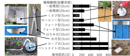
図-6 電極の種類および設置深度と接地抵抗の関係
