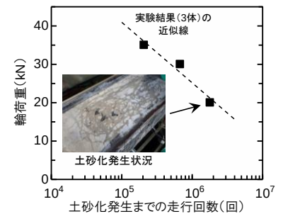
図-3 土砂化実験の結果
