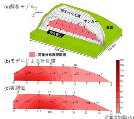
地すべり斜面の3次元モデルによるアンカー荷重増加量の再現結果
