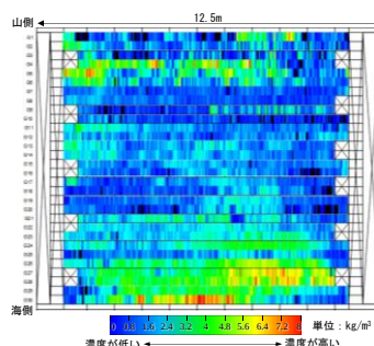
図-2 主桁下面の塩化物イオン濃度の可視化
