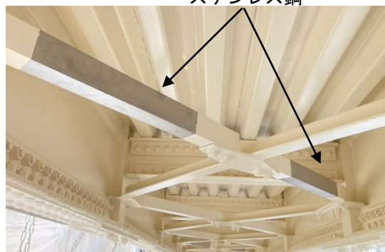
写真-3 側道橋の部材更新状況（左：施工前、右：施工後）
