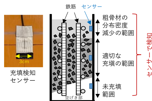
図-4 コンクリートの充填状況を確認できる技術の例
