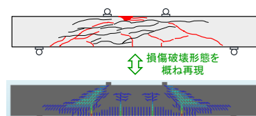
図-2 損傷破壊形態の比較例 （上：実験、下：解析）
