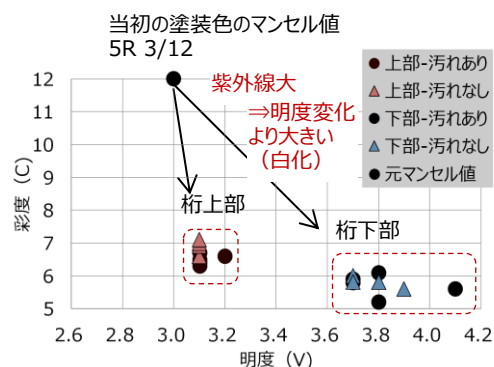
明度彩度の変化（赤系／30 年経過）
