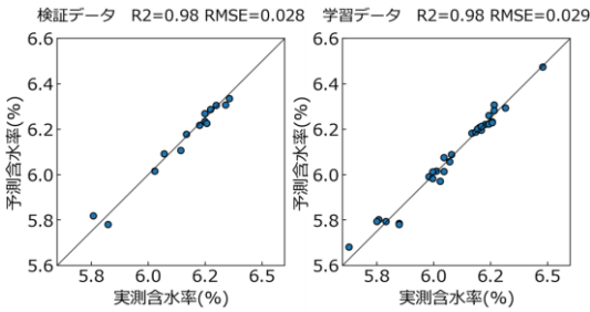
図-3 室内試験により作成したコンクリートの含水率予測モデルの予測値-実測値プロット
