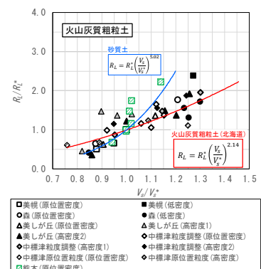
図-9 火山灰質土の V_s - R_L 関係
