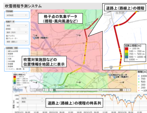
図-1 暴風雪時の判断支援システムにおける視程情報提供画面（モックアップ）
