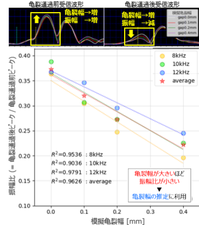
模擬亀裂幅と波形ピークの振幅比
