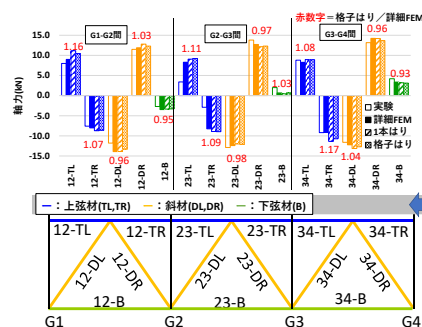
図-3 端対傾構の軸力の比較
