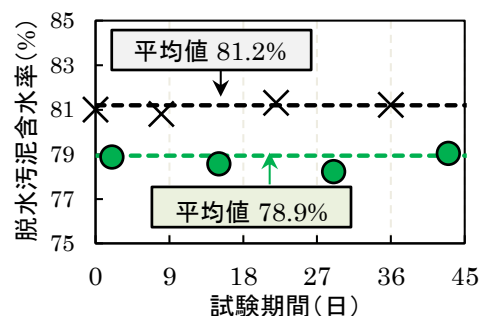
図-5 刈草混合脱水による含水率の変化(×汚泥のみ、●刈草混合)
