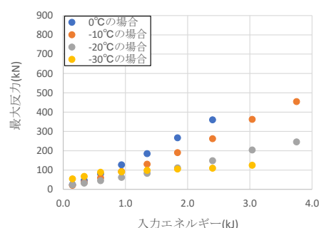
最大反力と入力エネルギーの関係 (緩衝材厚さ 50mm、硬度 55 度)
