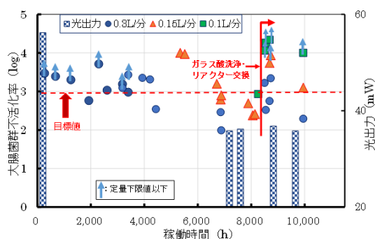
図-5 UV-LED消毒装置の稼働時間・光出力と通水条件ごとの大腸菌群不活化率
