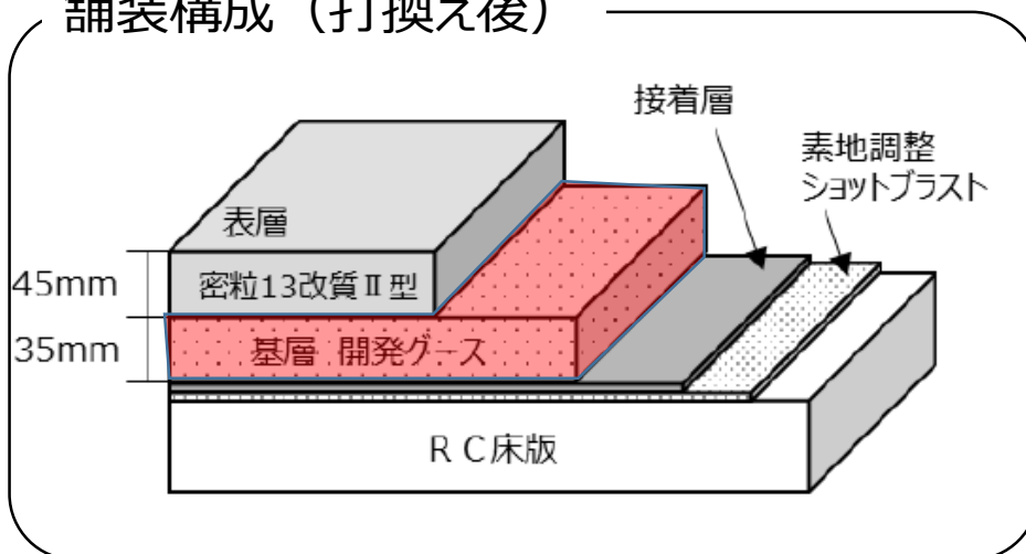
舗装構成（打換え後）
