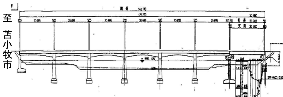
側面図
