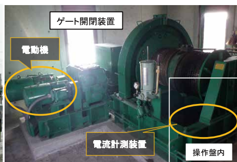
電動機操作盤内の動力線から電流を計測し、設備状態を診断
