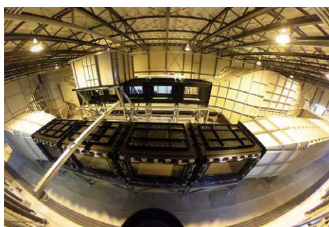
吹雪室内実験装置（石狩実験場内）
