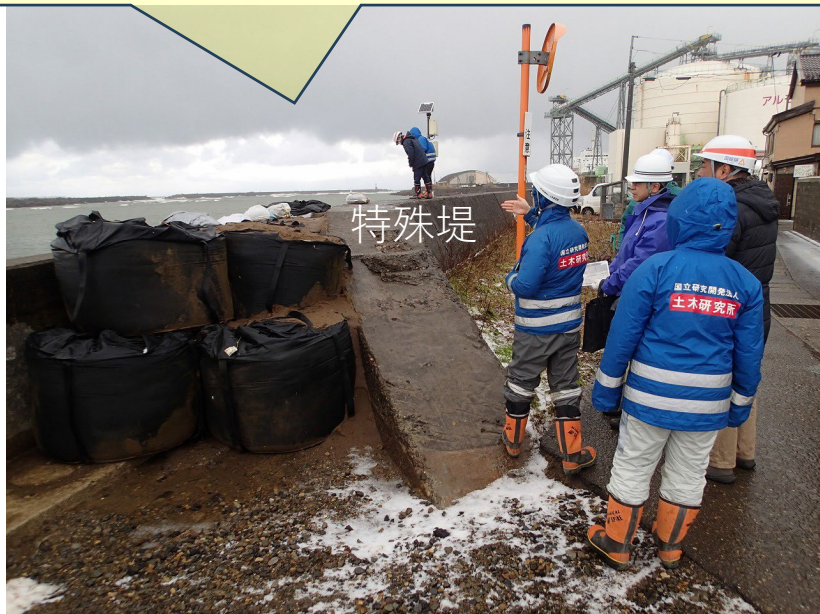
写真1 関川特殊堤の損傷に関する調査
