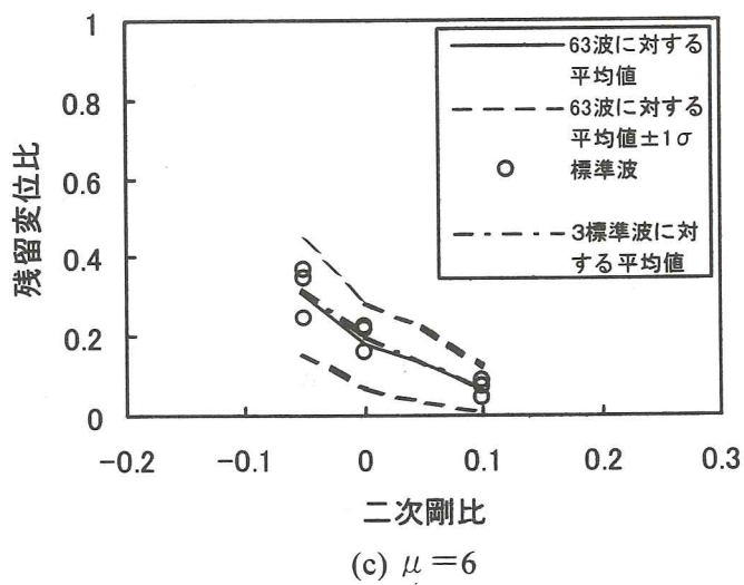
図-9.44 タイプⅡの地震動（Ⅱ種地盤）の3標準波形に対する残留変位比の平均値と63波の強震記録に対する平均値の比較
