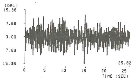
(14) 岩手県沖地震開北橋記録 ( M=7.2 , \Delta=190.9\text{km} , I種地盤)
