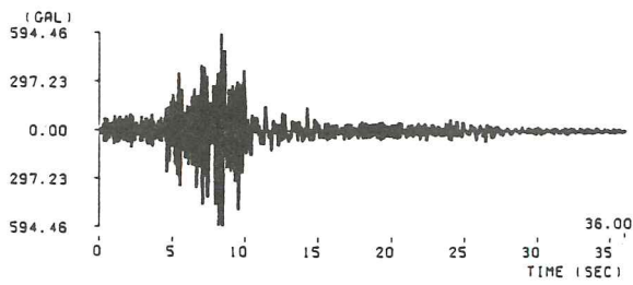
(16) 愛媛県西部沿岸地震板島橋記録 ( M=6.6 , \Delta=10.0\text{km} , II種地盤)
