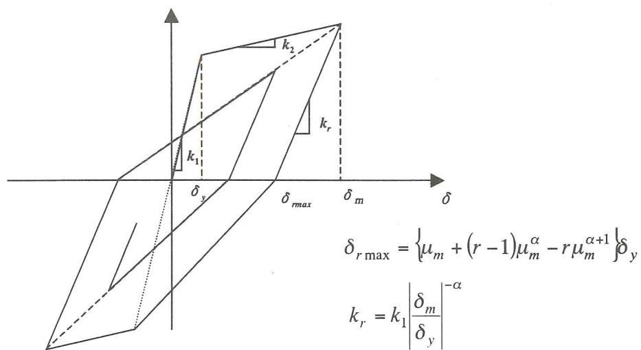
図-2.2 武田モデルにおける可能最大残留変位
