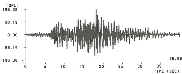
(3) 日向灘地震板島橋記録 ( M=7.5 , \Delta=103.3\text{km} , II種地盤)
