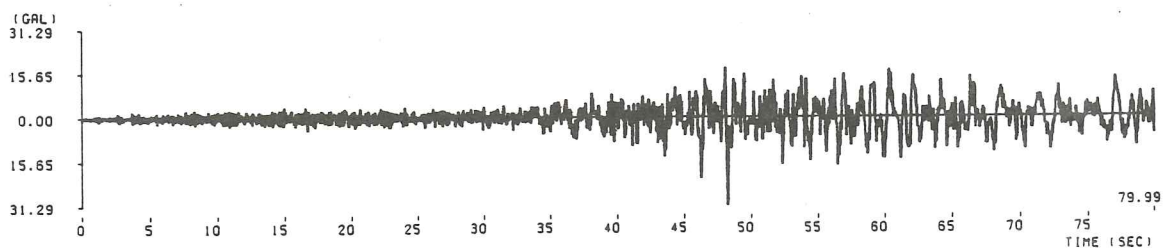
(45) 根室半島沖地震苫小牧港記録 ( M=7.4 , \Delta=357.3\text{km} , II種地盤)
