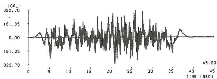
(3) I - I - 3 波形
