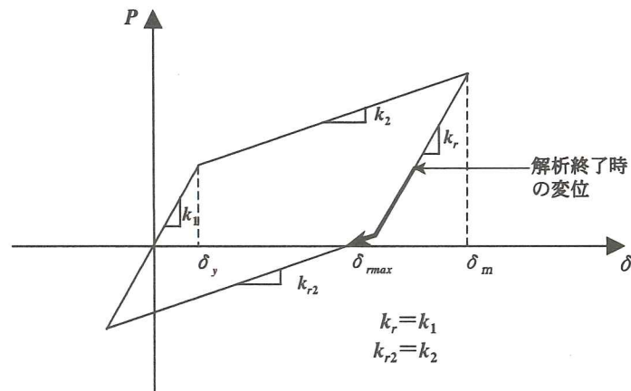
図-2.1 バイリニア型モデルにおける可能最大残留変位
