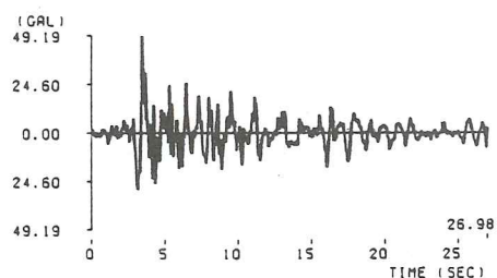
(50) 伊豆半島南部沿岸近海地震東京湾（富津岬）記録 ( M=6.9 , \Delta=123.2\text{km} , II種地盤)
