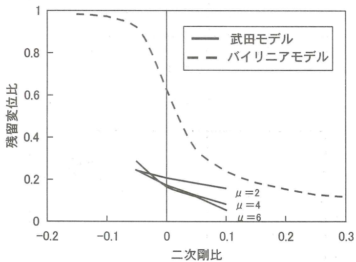
図-7.3 履歴復元力特性が残留変位比に及ぼす影響
