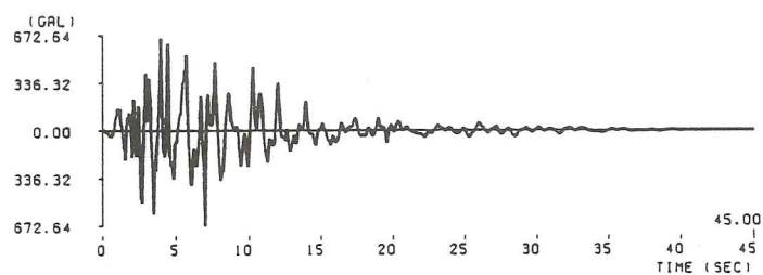
(14) II - II - 2 波形
