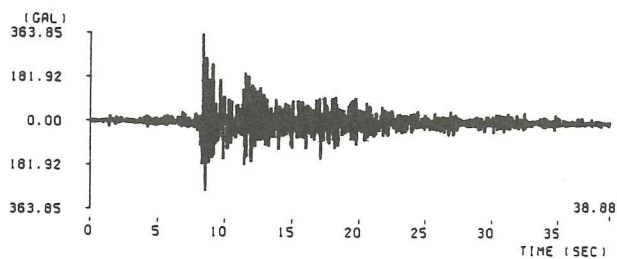
(59) 宮城県沖地震開北橋記録 ( M=7.4 , \Delta=81.4\text{km} , Ⅰ種地盤)
