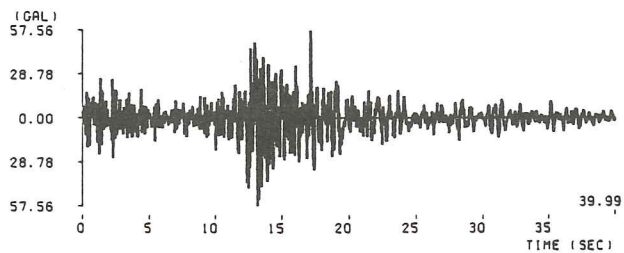
(23) 岐阜県中部地震衣浦港記録 ( M=6.6 , \Delta=97.3\text{km} , III種地盤)
