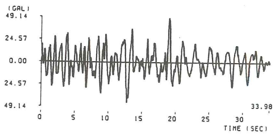
(6) 日向灘地震有明海堤防記録 ( M=7.5 , \Delta=233.7\text{km} , Ⅲ種地盤)
