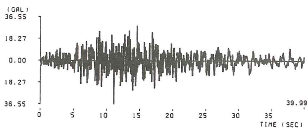
(48) 伊豆半島南部沿岸近海地震田子ノ浦記録 ( M=6.9 , \Delta=63.9\text{km} , III種地盤)
