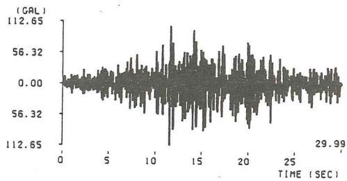
(8) 東北東方沖地震幌満橋記録 ( M=7.9 , \Delta=155.1\text{km} , I種地盤)
