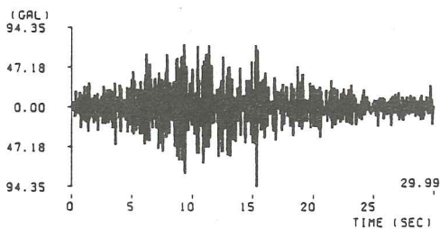
(10) 青森県東方沖地震幌満橋記録 ( M=7.5 , \Delta=74.0\text{km} , I種地盤)
