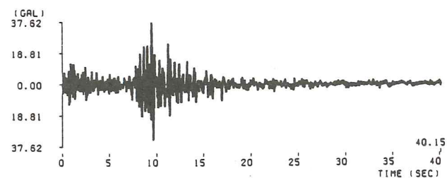
(63) 伊豆半島付近地震東名・富士川記録 ( M=6.7 , \Delta=61.3\text{km} , II種地盤)
