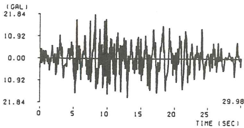
(40) 八丈島東方沖地震平井大橋記録（ M=7.2 , \Delta=301.0\text{km} , II種地盤）
