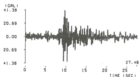
(49) 伊豆半島南部沿岸近海地震東京湾（観音崎）記録 ( M=6.9 , \Delta=115.0\text{km} , I種地盤)
