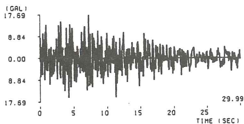
(35) 八丈島東方沖地震久里浜港記録 ( M=7.2 , \Delta=257.6\text{km} , III種地盤)
