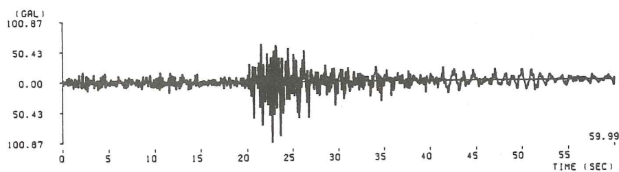
(33) 襟裳岬沖地震釧路港記録 ( M=7.0 , \Delta=201.7\text{km} , II種地盤)
