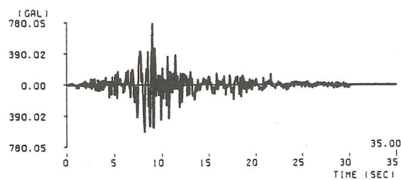
(12) II - I - 3 波形
