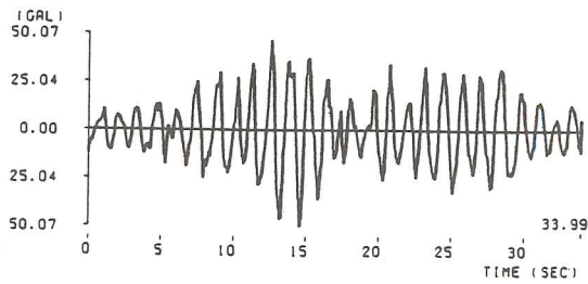
(7) 日向灘地震妙見橋記録 ( M=7.5 , \Delta=341.3\text{km} , Ⅲ種地盤)
