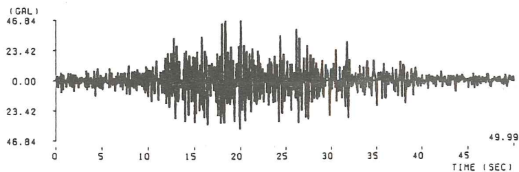
(28) 北海道南部地方地震室蘭港記録 ( M=6.7 , \Delta=177.2\text{km} , II種地盤)
