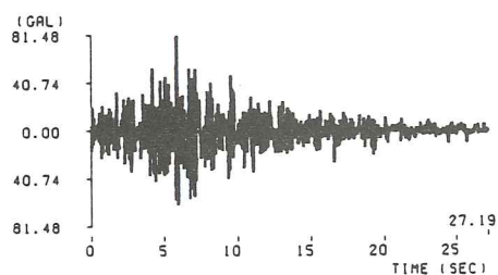
(53) 大島近海地震白堀変電所記録 ( M=7.0 , \Delta=44.7\text{km} , I種地盤)
