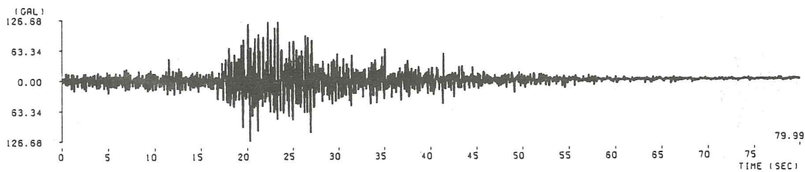
(11) 青森県東方沖地震室蘭港記録 ( M=7.5 , \Delta=184.0\text{km} , II種地盤)
