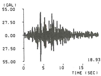
(21) 岐阜県中部地震四徳大橋記録 ( M=6.6 , \Delta=85.5\text{km} , II種地盤)
