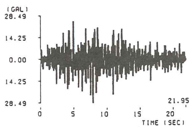
(43) 八丈島東方沖地震伊達橋記録 ( M=7.2 , \Delta=517.2\text{km} , I種地盤)
