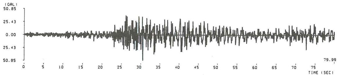
(20) 北海道東部地震釧路港記録 ( M=7.8 , \Delta=265.1\text{km} , II種地盤)
