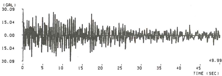
(39) 八丈島東方沖地震東京湾（品川）記録（ M=7.2 , \Delta=293.2\text{km} , II種地盤）
