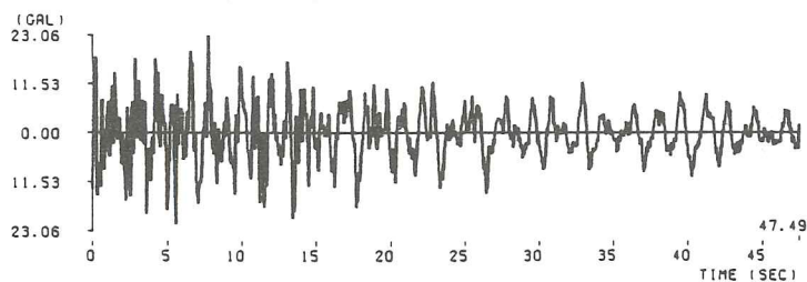
(15) 岩手県沖地震青森港記録 ( M=7.2 , \Delta=254.0\text{km} , III種地盤)
