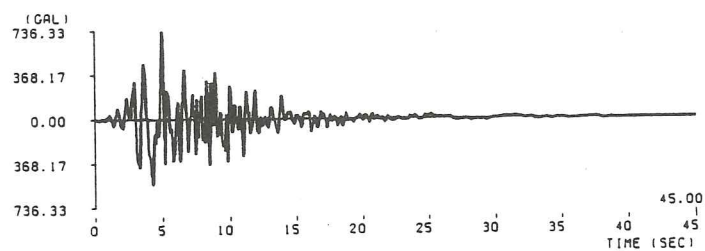
(15) II - II - 3 波形
