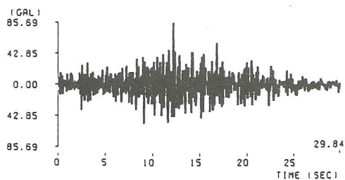
(55) 大島近海地震東京湾(観音崎)記録 ( M=7.0 , \Delta=70.3\text{km} , I種地盤)
