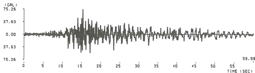
(47) 根室半島沖地震釧路港記録 ( M=7.1 , \Delta=192.4\text{km} , II種地盤)
