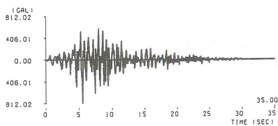
(10) II - I - 1 波形
