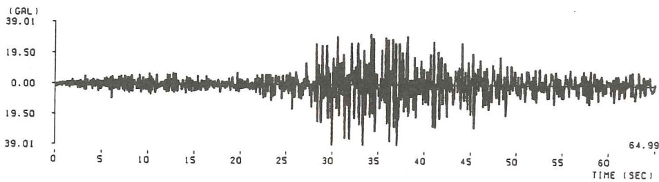
(38) 八丈島東方沖地震横浜港（京浜）記録（ M=7.2 , \Delta=282.7\text{km} , II種地盤）
