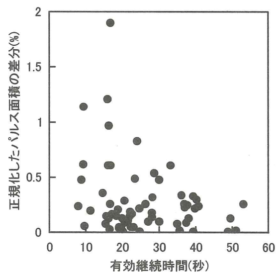
(b)パルス面積の差分との関係
