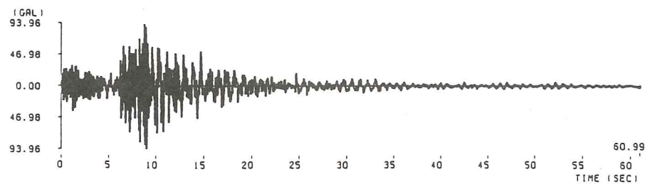
(19) 日向灘地震細島港記録 ( M=6.5 , \Delta=51.4\text{km} , II種地盤)
