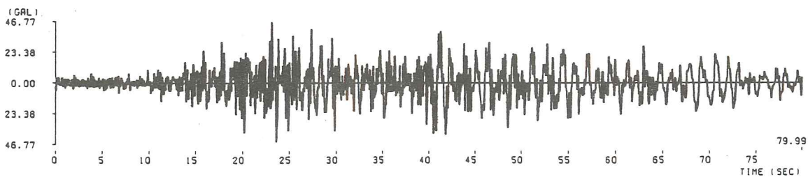
(9) 東北東方沖地震釧路港記録 ( M=7.9 , \Delta=257.9\text{km} , Ⅱ種地盤)
