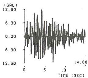
(24) 岐阜県中部地震豊浜大橋記録 ( M=6.6 , \Delta=145.9\text{km} , II種地盤)
