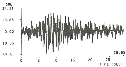
(61) 宮城県沖地震雄平橋記録 ( M=7.4 , \Delta=188.1\text{km} , II種地盤)
