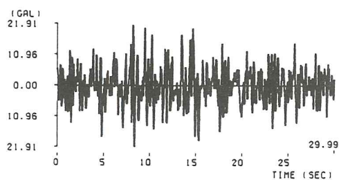
(46) 根室半島沖地震室蘭港記録 ( M=7.4 , \Delta=412.8\text{km} , II種地盤)
