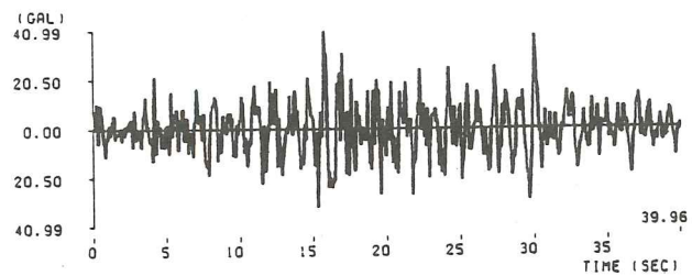
(62) 宮城県沖地震新利根川橋記録 ( M=7.4 , \Delta=312.2\text{km} , II種地盤)
