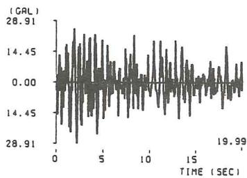
(4) 日向灘地震石瀬戸橋記録 ( M=7.5 , \Delta=136.0\text{km} , II種地盤)
