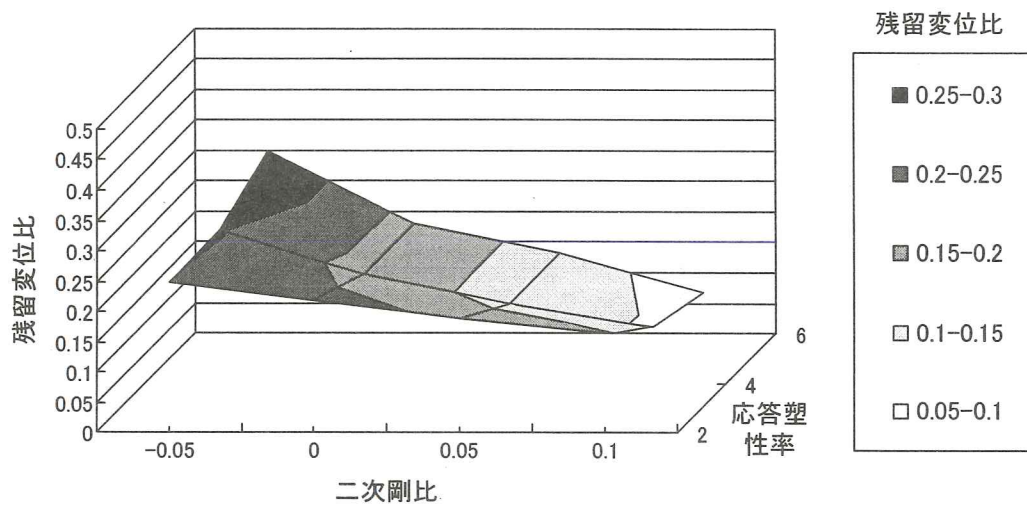
図-7.2 応答塑性率と二次剛比と残留変位比の関係
