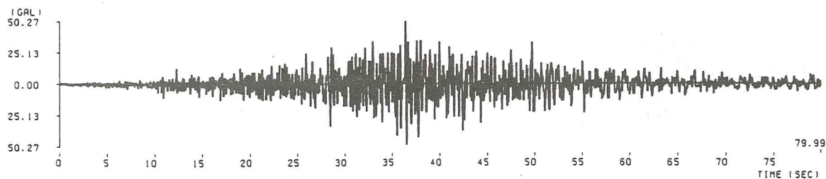
(13) 岩手県沖地震八戸港記録 ( M=7.2 , \Delta=182.7\text{km} , II種地盤)
