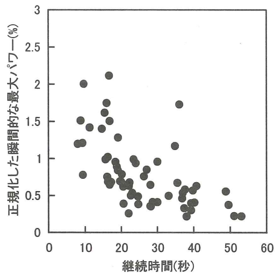
図-3.2 地震動の継続時間と瞬間的な最大パワーの関係
