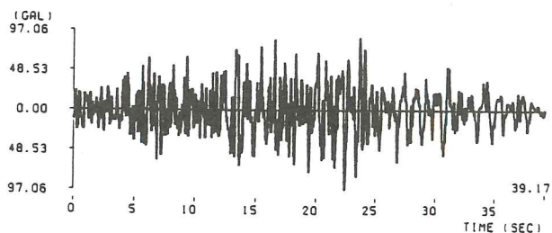
(60) 宮城県沖地震平大橋記録 ( M=7.4 , \Delta=164.6\text{km} , Ⅱ種地盤)
