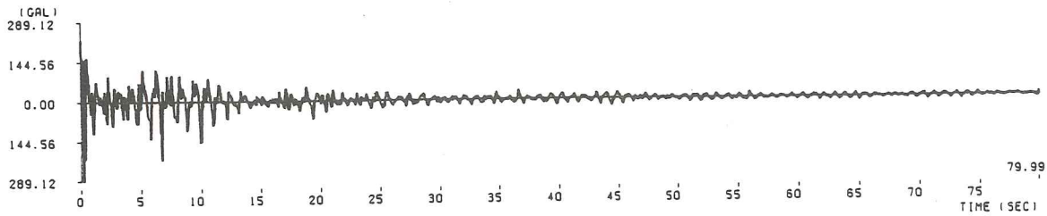
(2) 日向灘地震細島港記録 ( M=7.5 , \Delta=32.2\text{km} , II種地盤)
