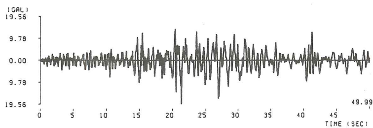
(51) 伊豆半島南部沿岸近海地震横浜港(1)記録 ( M=6.9 , \Delta=124.9\text{km} , Ⅲ種地盤)
