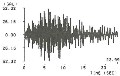
(22) 岐阜県中部地震新八幡橋記録 ( M=6.6 , \Delta=89.1\text{km} , I種地盤)
