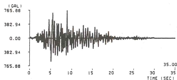
(11) II - I - 2 波形
