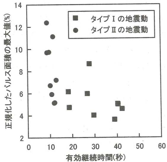
図-9.3 標準波形の地震動の継続時間とパルス面積の最大値との関係
