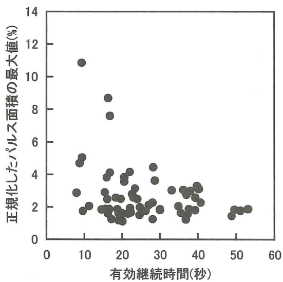
(a)パルス面積の最大値との関係
