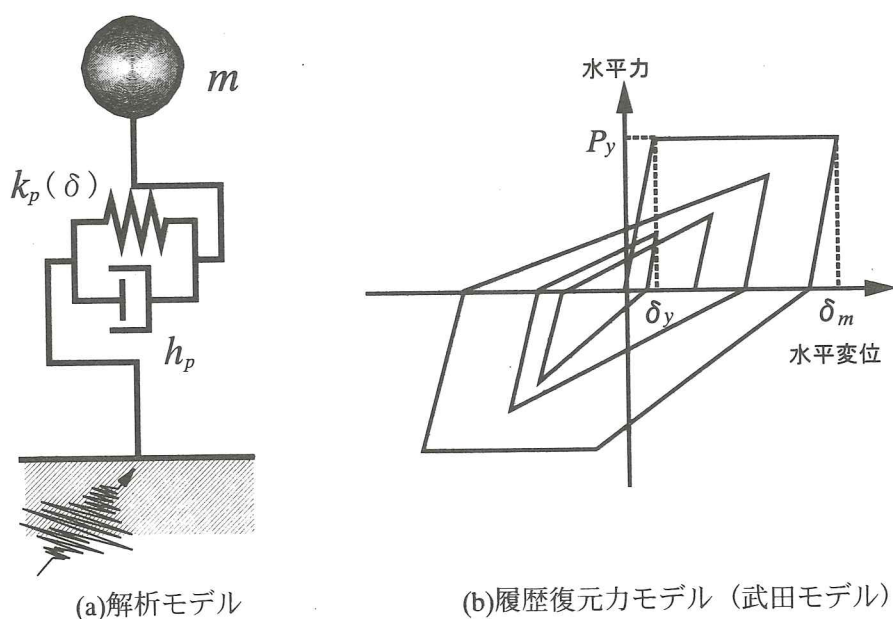
図-3.1 解析モデルの概要
