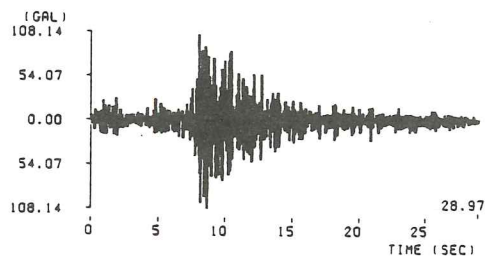
(57) 宮城県沖地震開北橋記録 ( M=6.7 , \Delta=84.2\text{km} , Ⅰ種地盤)
