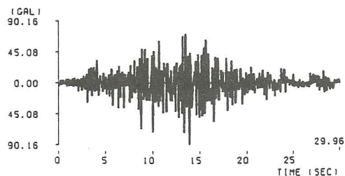
(54) 大島近海地震沼津変電所記録 ( M=7.0 , \Delta=53.7\text{km} , I種地盤)
