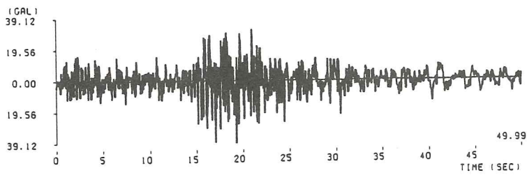
(1) 越前岬沖地震名古屋港記録 ( M=6.9 , \Delta=127\text{km} , II種地盤)
