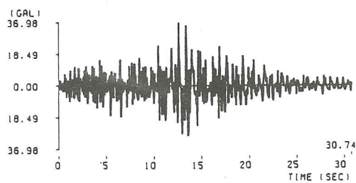
(31) 宮崎県沖地震石瀬戸橋記録 ( M=6.7 , \Delta=84.9\text{km} , II種地盤)
