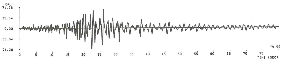
(5) 日向灘地震高知港記録 ( M=7.5 , \Delta=167.4\text{km} , III種地盤)
