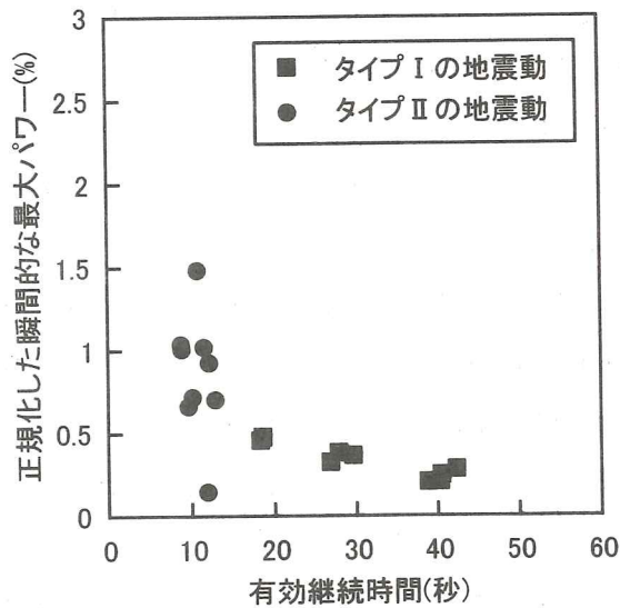
図-9.2 標準波形の地震動の継続時間と瞬間的な最大パワーの関係
