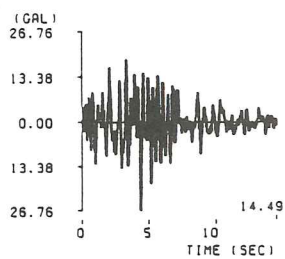
(26) 岐阜県中部地震神戸港記録 ( M=6.6 , \Delta=207.5\text{km} , II種地盤)
