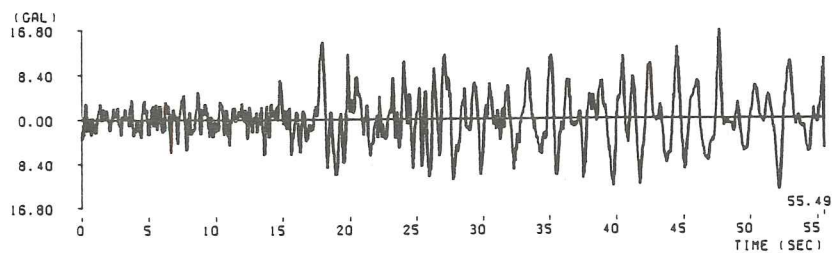
(32) 宮崎県沖地震鹿児島港記録 ( M=6.7 , \Delta=149.6\text{km} , III種地盤)
