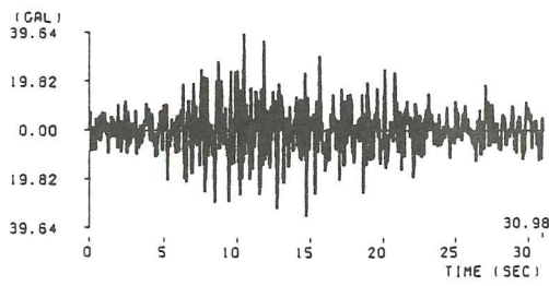
(36) 八丈島東方沖地震東京湾（観音崎）記録（ M=7.2 , \Delta=258.8\text{km} , I種地盤）
