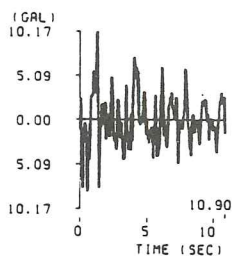
(25) 岐阜県中部地震西横堀高架橋記録 ( M=6.6 , \Delta=188.7\text{km} , II種地盤)
