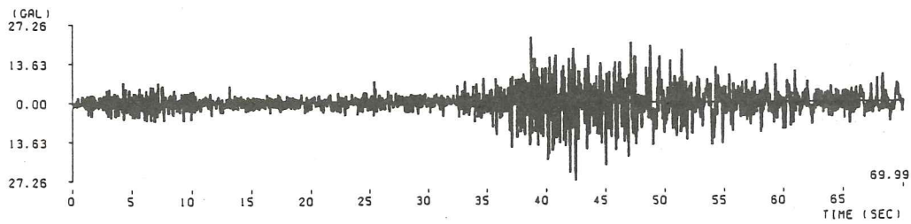
(42) 八丈島東方沖地震小浜名港記録 ( M=7.2 , \Delta=416.5\text{km} , II種地盤)
