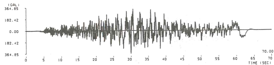
(6) I - II - 3 波形
