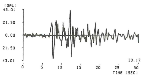
(56) 大島近海地震新岩田変電所記録 ( M=7.0 , \Delta=108.5\text{km} , Ⅲ種地盤)
