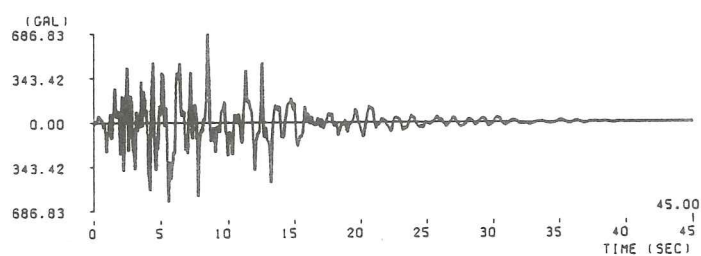
(13) II - II - 1 波形
