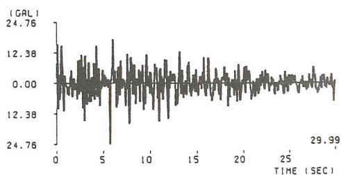
(29) 北海道南部地方地震八戸港記録 ( M=6.7 , \Delta=246.1\text{km} , II種地盤)
