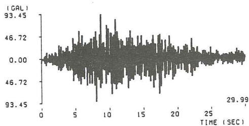
(52) 大島近海地震熱海変電所記録 ( M=7.0 , \Delta=41.2\text{km} , I種地盤)
