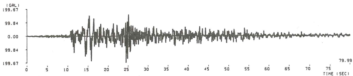
(44) 根室半島沖地震釧路港記録 ( M=7.4 , \Delta=127.3\text{km} , II種地盤)
