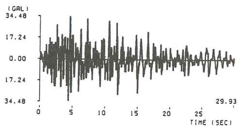
(58) 宮城県沖地震平大橋記録 ( M=6.7 , \Delta=219.9\text{km} , Ⅱ種地盤)
