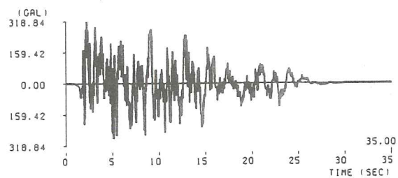
(1) I - I - 1 波形
