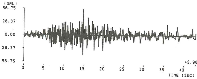
(37) 八丈島東方沖地震東京湾（富津岬）記録（ M=7.2 , \Delta=262.0\text{km} , II種地盤）
