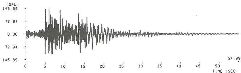
(30) 宮城県沖地震細島港記録 ( M=6.7 , \Delta=51.9\text{km} , II種地盤)
