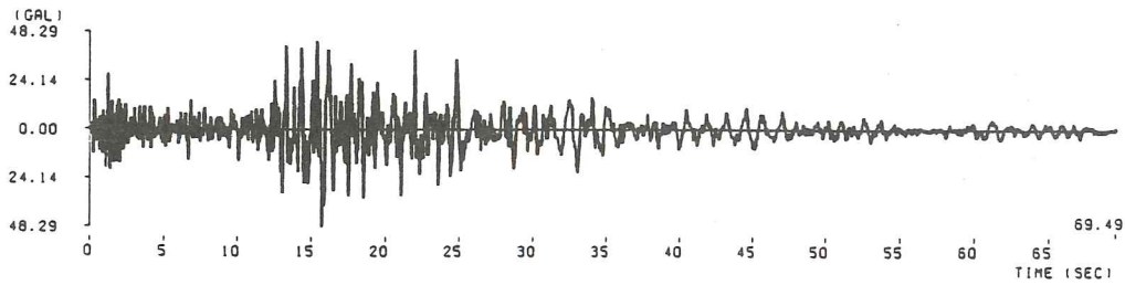
(17) 愛媛県西部沿岸地震高知港記録 ( M=6.6 , \Delta=112.5\text{km} , III種地盤)
