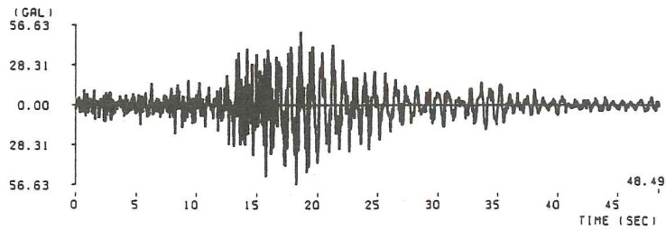
(18) 愛媛県西部沿岸地震細島港記録 ( M=6.6 , \Delta=118.2\text{km} , II種地盤)
