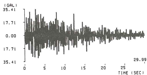
(34) 襟裳岬沖地震室蘭港記録 ( M=7.0 , \Delta=255.4\text{km} , II種地盤)
