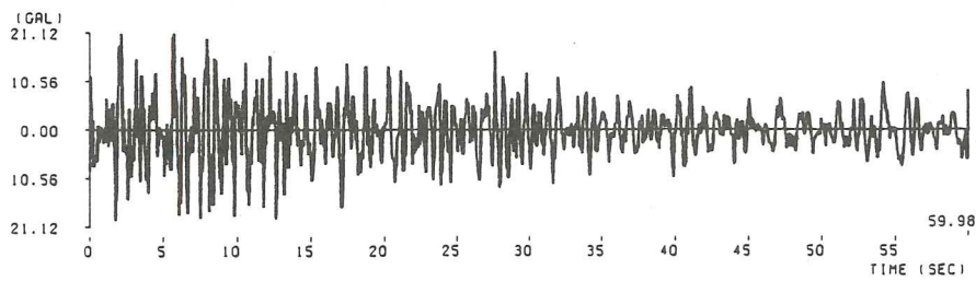
(41) 八丈島東方沖地震草加高架橋記録 ( M=7.2 , \Delta=312.6\text{km} , III種地盤)
