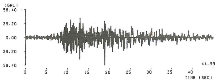
(27) 北海道南部地方地震釧路港記録 ( M=6.7 , \Delta=121.6\text{km} , II種地盤)
