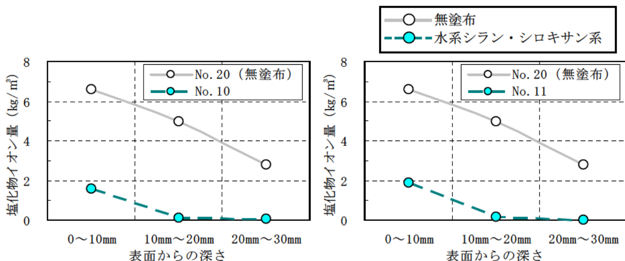
図－Ⅲ. 2. 39 (1) シラン・シロキサン系（水系）の塩化物イオン量
