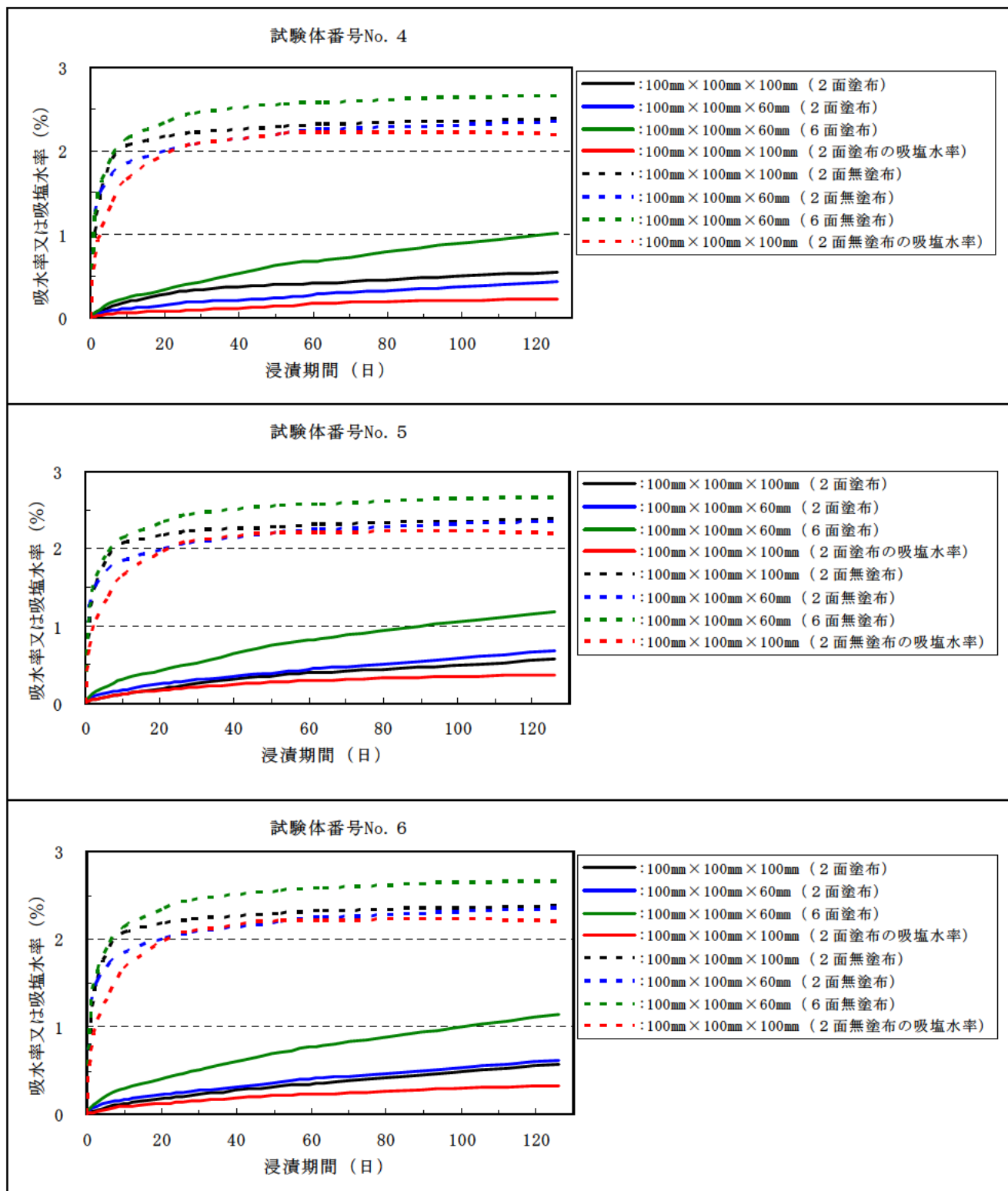
付録図－3.3.1(2) 浸漬 126 日の測定結果（シラン系）
