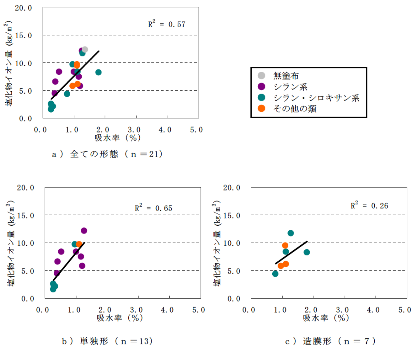
図－Ⅲ.1.141 吸水率 (7日後) と上面の塩化物イオン量
