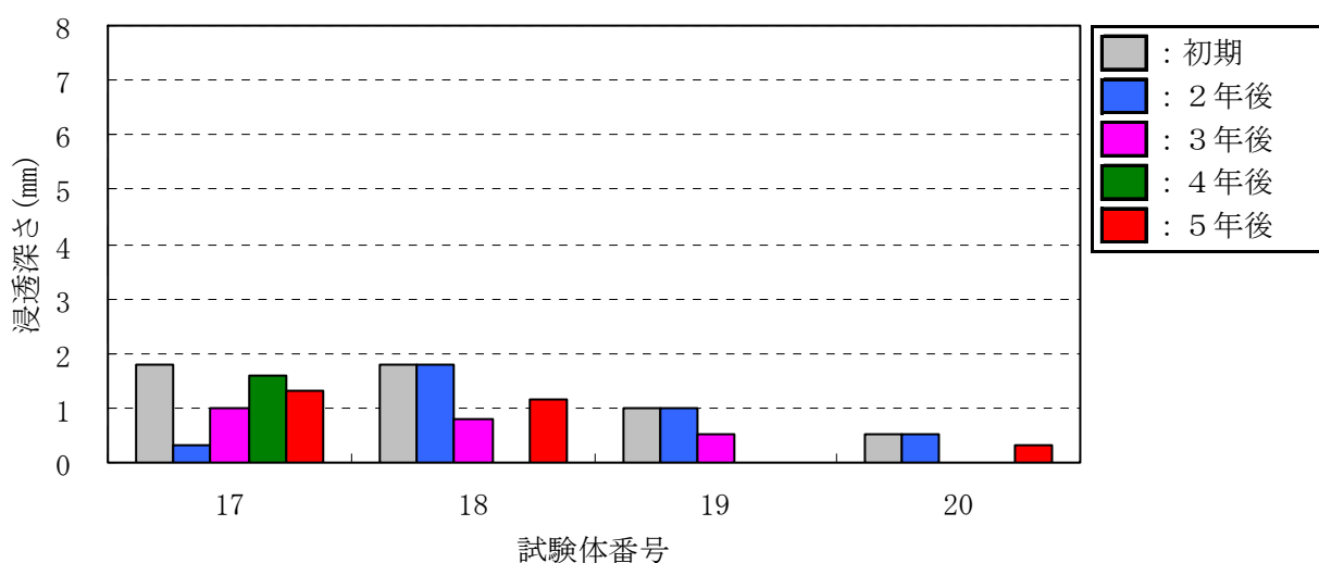
図－Ⅲ.1.64 その他の類の浸透深さ(国道側)
