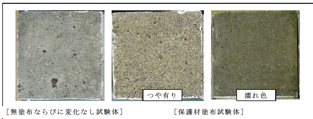
図－Ⅲ.1.3 評価基準の例
