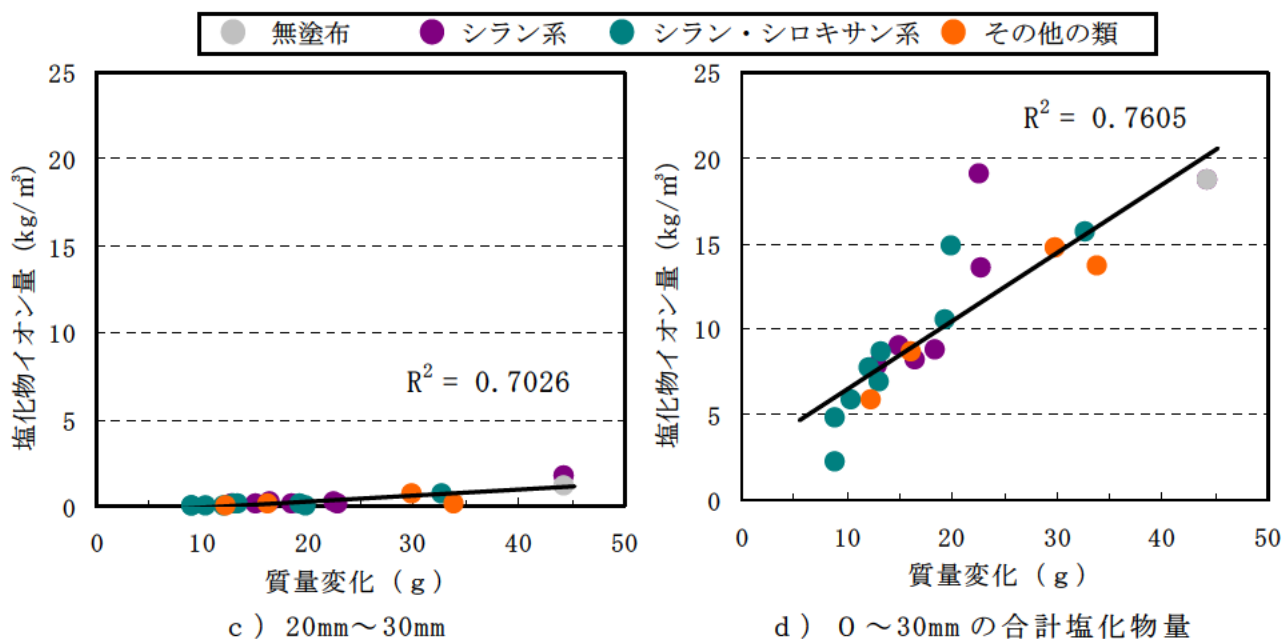
図－Ⅲ.1.43(2) 質量変化と深さ方向の塩化物イオン量との関係 (2) ( n = 21 )
