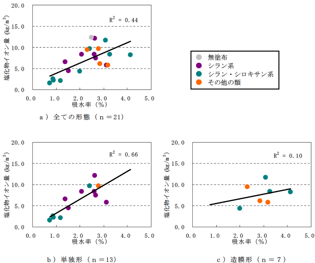
図－Ⅲ.1.142 吸水率 (45 日後) と上面の塩化物イオン量
