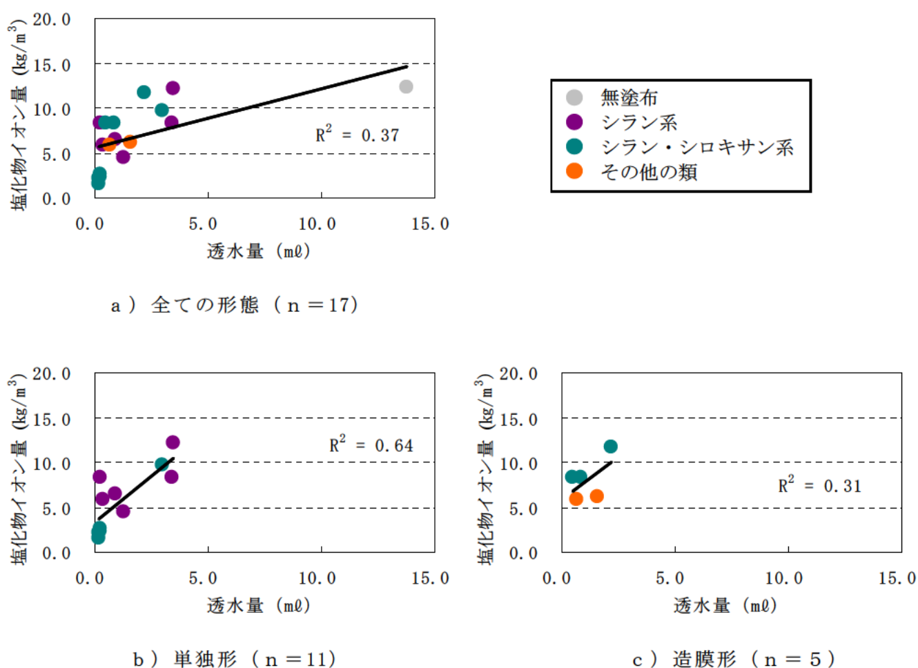
図－Ⅲ.1.145 上面の塩化物イオン量と透水量（室内試験）
