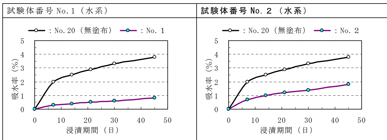
付録図－4.2.1(1) 吸水率測定結果 (シラン系)
