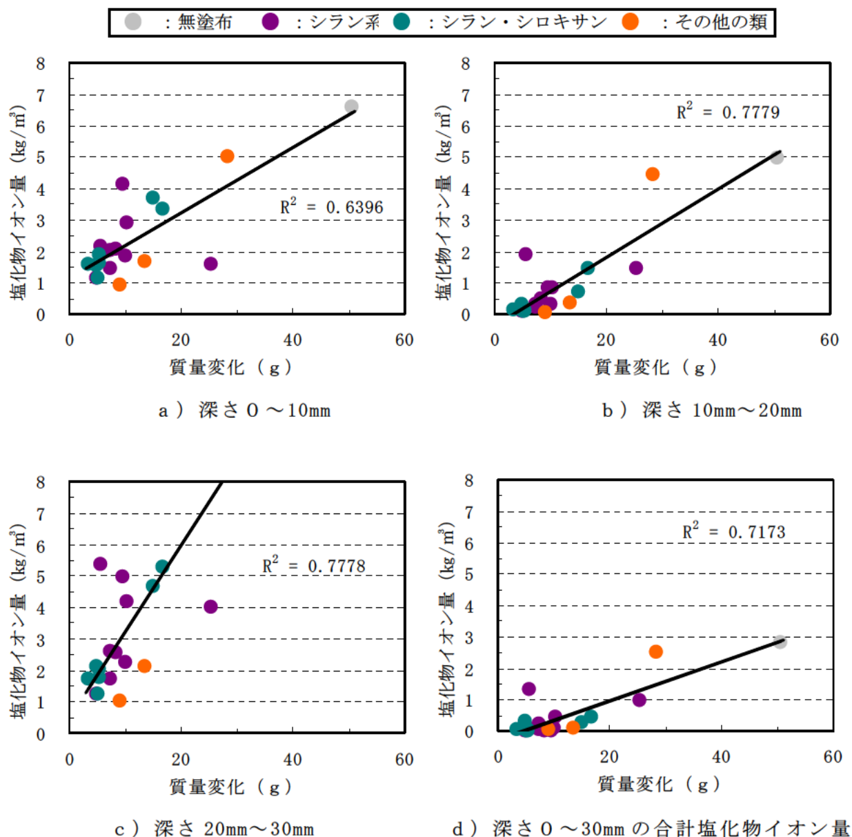
図－Ⅲ. 2. 41 質量変化と深さ方向の塩化物イオン量との関係 ( n = 20 )
