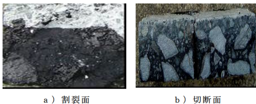
写真－Ⅲ. 1. 11 試験面の状態(割裂面と切断面)による浸透深さ
