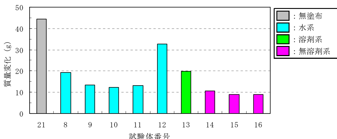
図－Ⅲ.1.29 シラン・シロキサン系の質量変化（浸漬 90 日）
