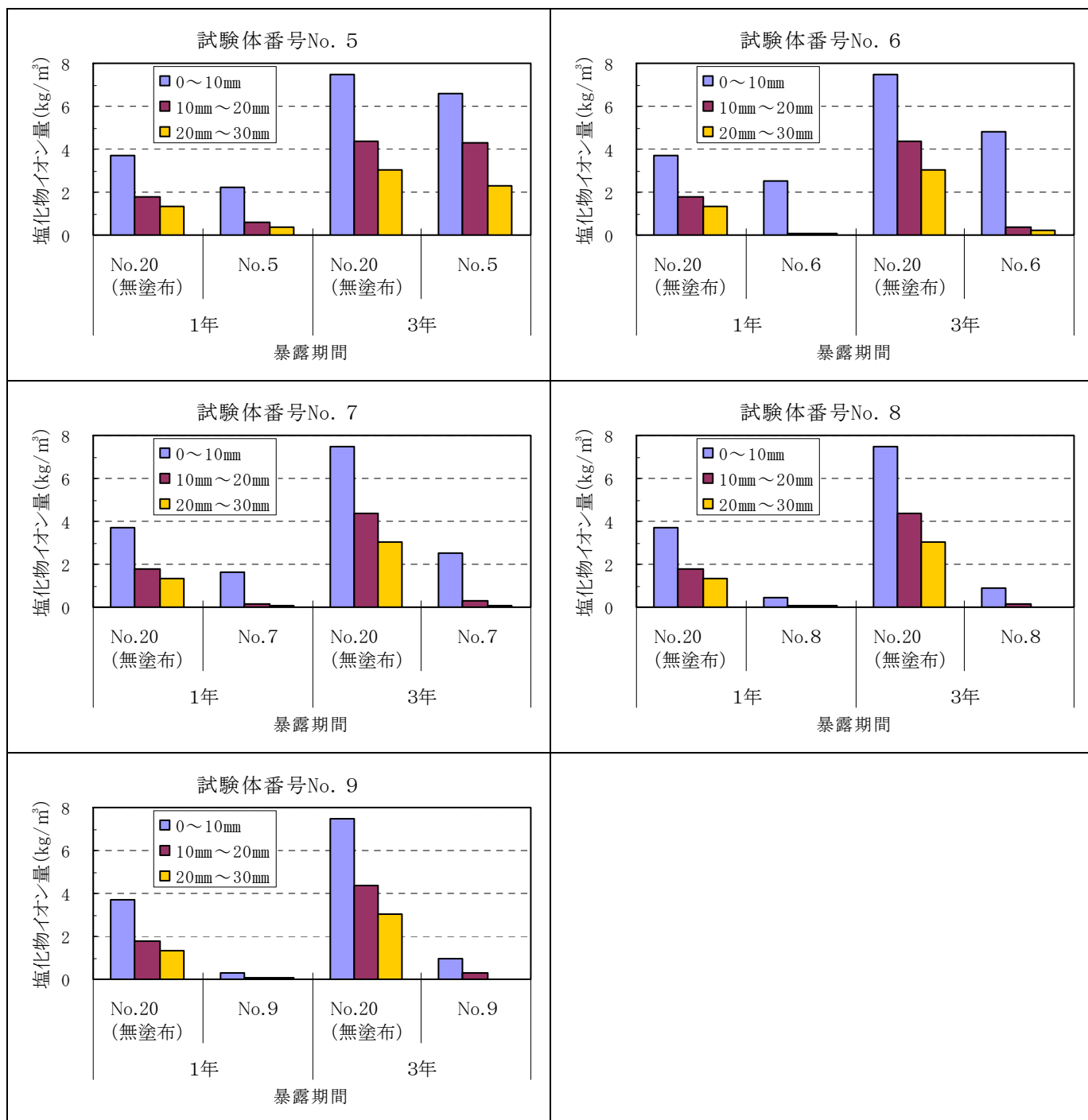
付録図－4.3.1(2) 塩化物イオン量（シラン系）
