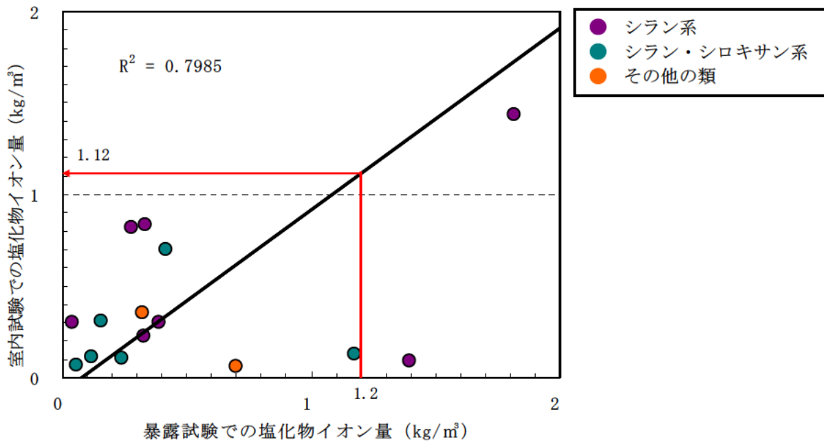
図－V.2.2 鉄筋腐食発生限界値での暴露試験と室内試験との関係（ n = 16 ）
