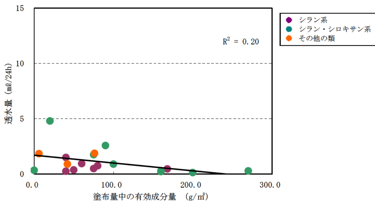
図－Ⅲ．1.84 暴露２年後の透水量と有効成分との関係（ n = 20 ）
