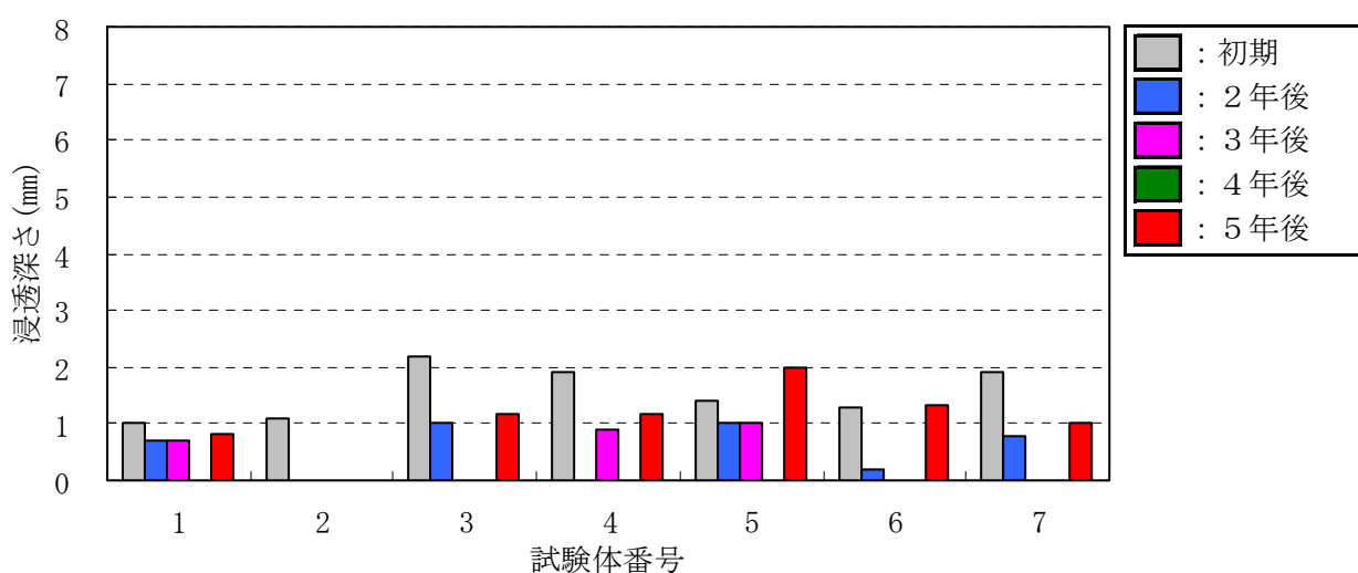
図－Ⅲ．１．６９ シラン系の浸透深さ
