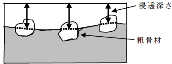
図－Ⅲ. 2. 7 測定箇所粗骨材がある場合の測定方法
