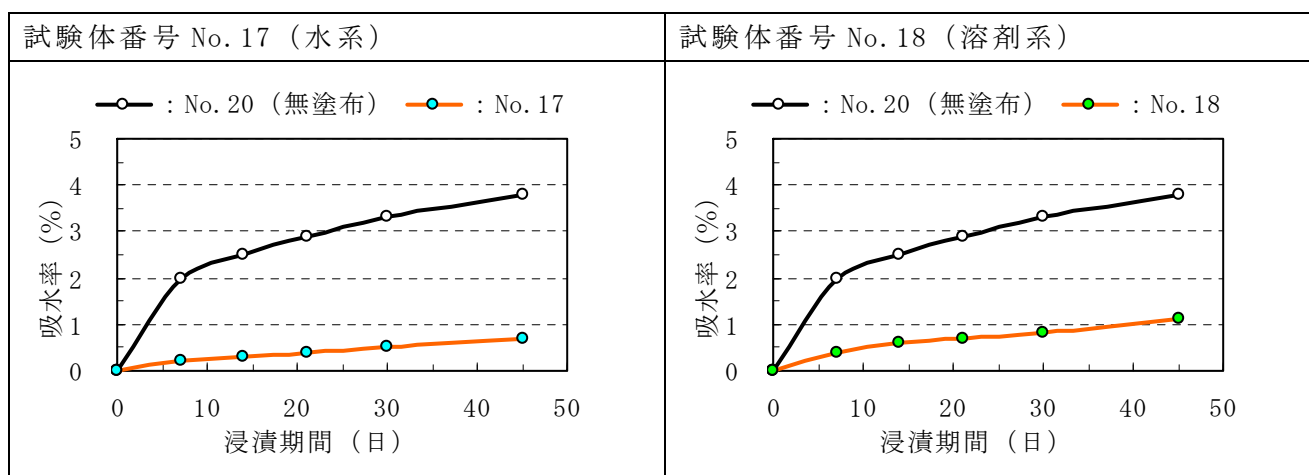
付録図－4. 2. 3(1) 吸水率測定結果 (その他の類)
