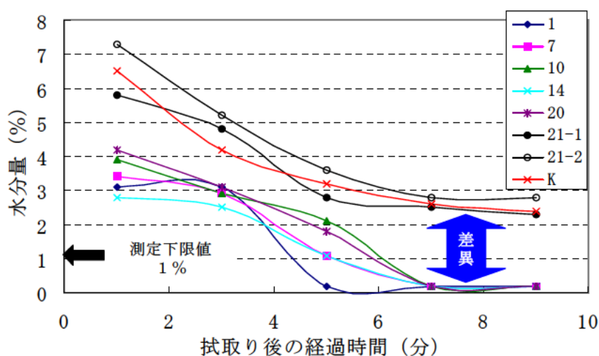
図－Ⅳ.2.8 保護材の種類による拭取り後の水分量
