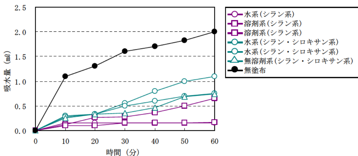
図－Ⅳ.1.1 実構造物での吸水量の測定
