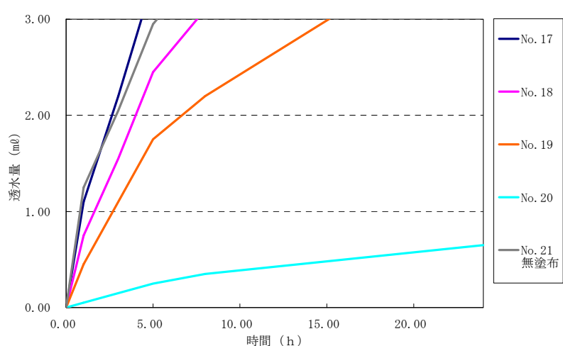
付録図－2.4.3 暴露3年後の透水量測定結果
