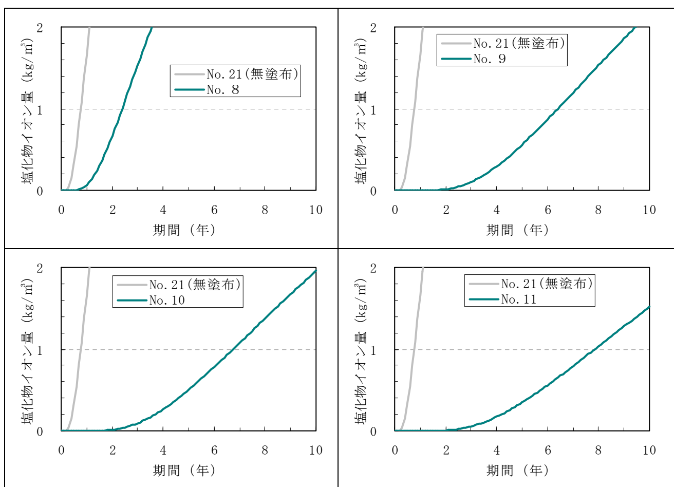
付録図－1.6.5(1) 促進試験での耐久性予測（シラン・シロキサン系）
