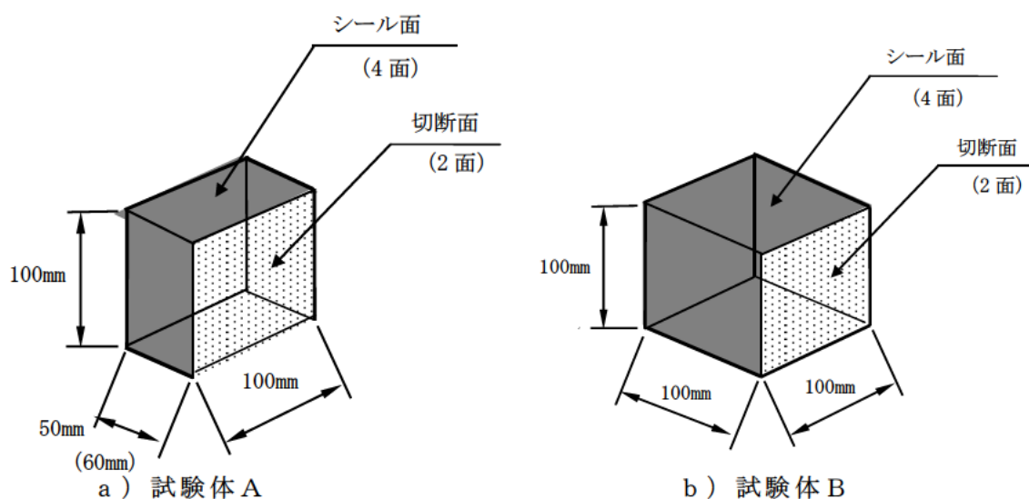
図－Ⅲ.2.4 試験体の形状
