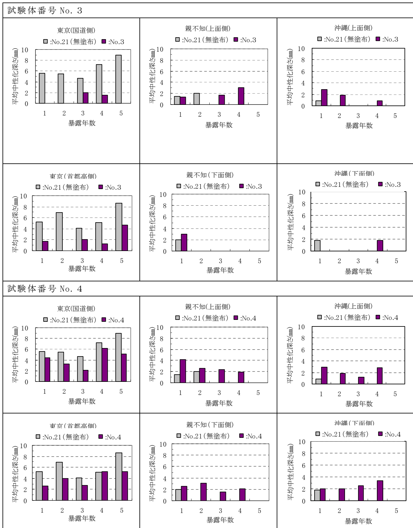
付録図－2.7.1(2) 中性化深さ測定結果（シラン系）
