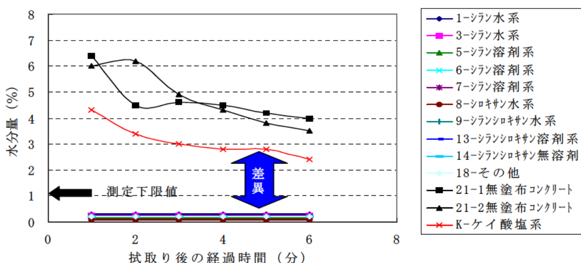
図－Ⅳ.2.25 つくば7年暴露大型試験体の水分量の経時変化
