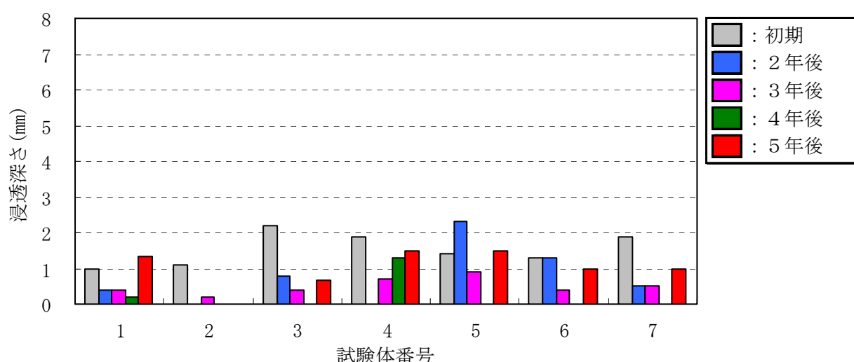
図－Ⅲ. 1. 60 シラン系の浸透深さ(国道側)
