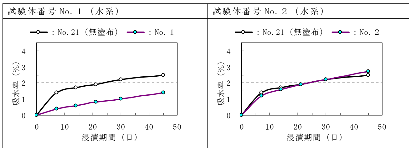
付録図－2.8.1(1) 吸水率測定結果 (シラン系)
