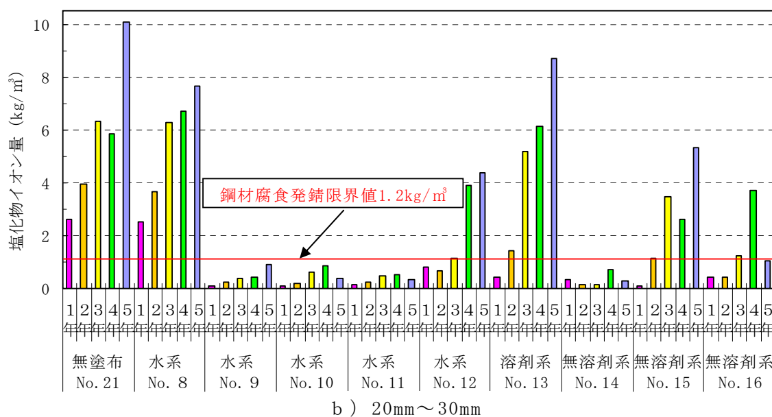
図－Ⅲ.1.108(1) 親不知暴露シラン・シロキサン系の塩化物イオン量
