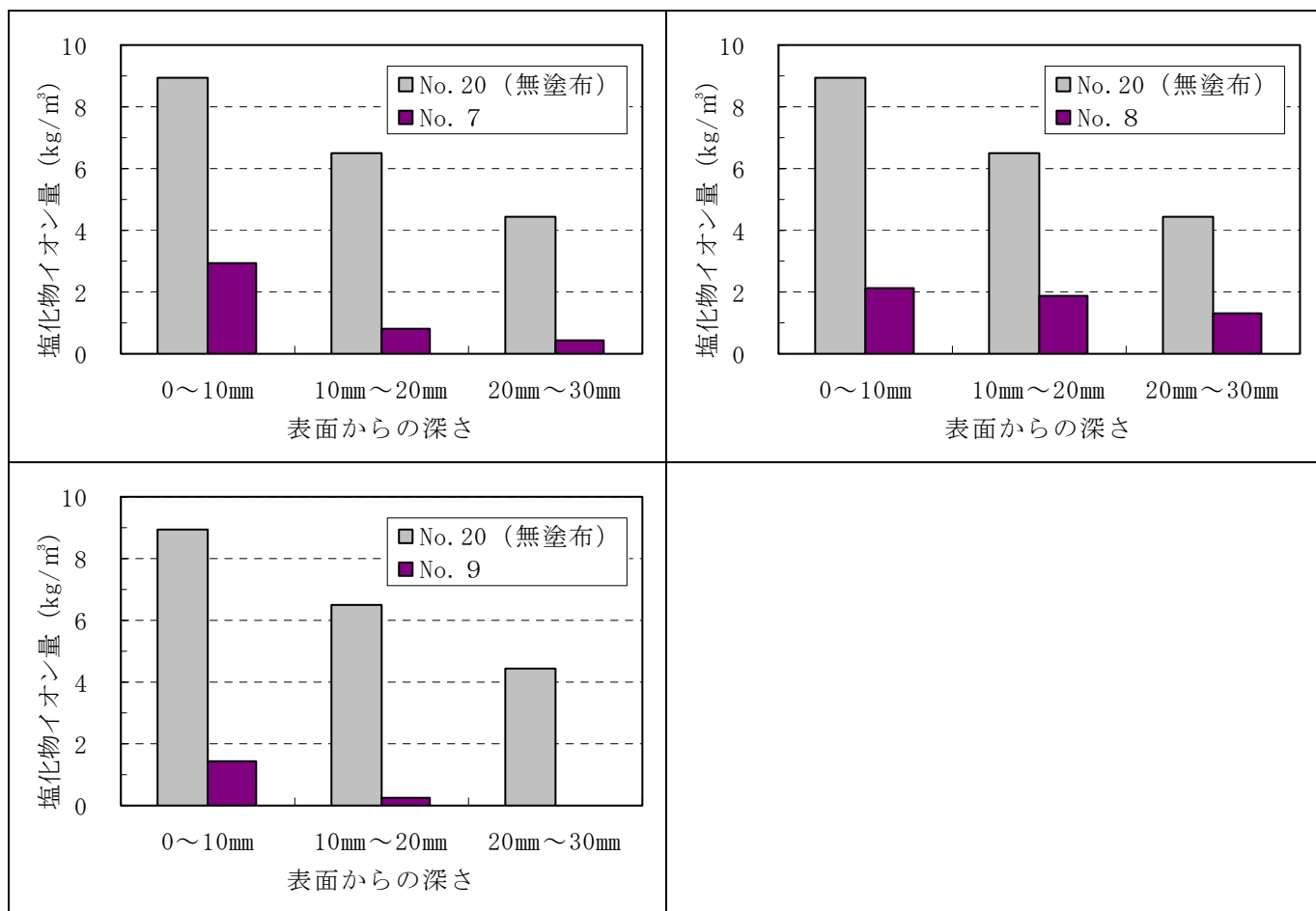
付録図－3.4.1(2) 塩化物イオン量（シラン系）
