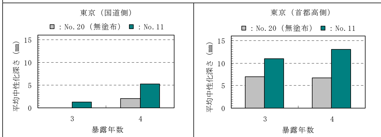
付録図－4.4.2(1) 中性化深さ測定結果（シラン・シロキサン系）
