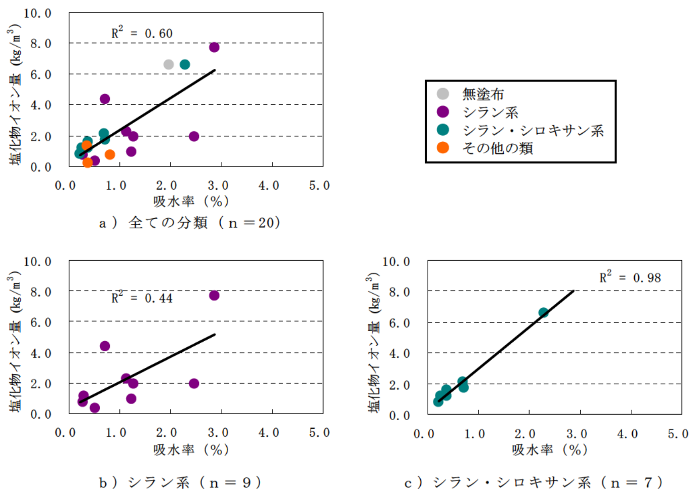
図－Ⅲ.2.55 吸水率（7日後）と塩化物イオン量
