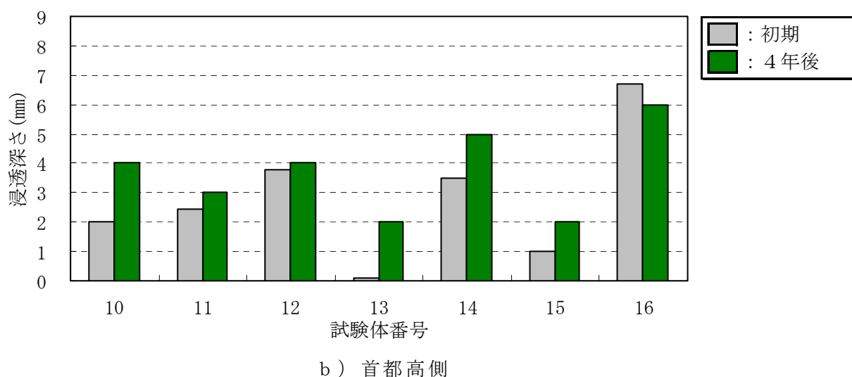
図－Ⅲ. 2. 46 シラン・シロキサン系の浸透深さ
