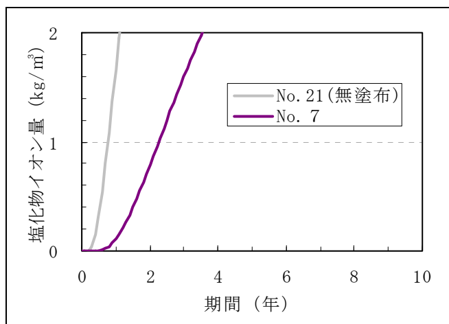
付録図－1.6.4(2) 促進試験での耐久性予測（シラン系）
