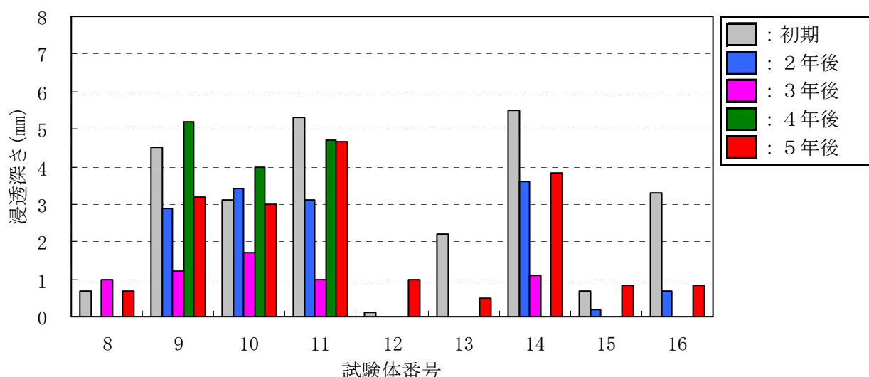
図－Ⅲ. 1. 70 シラン・シロキサン系の浸透深さ
