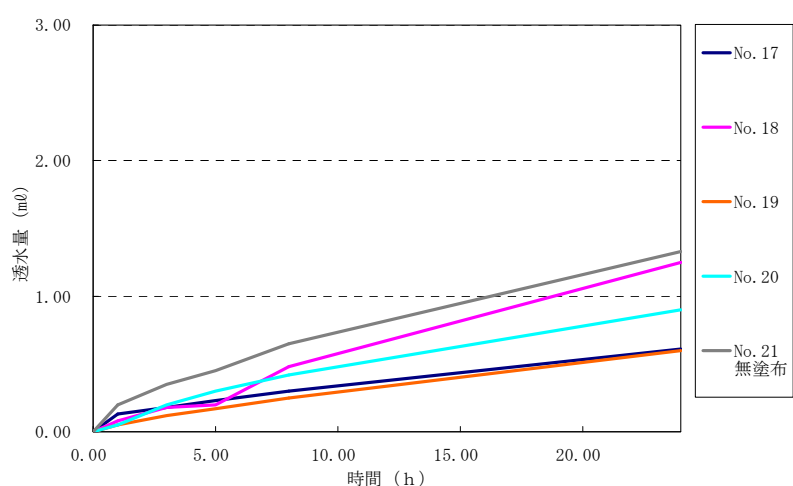
付録図－2.4.2 暴露2年後の透水量測定結果
