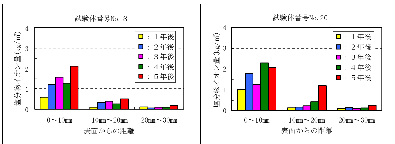
付録図－2.6.3(1) 塩化物イオン量測定結果（シラン・シロキサン系）
