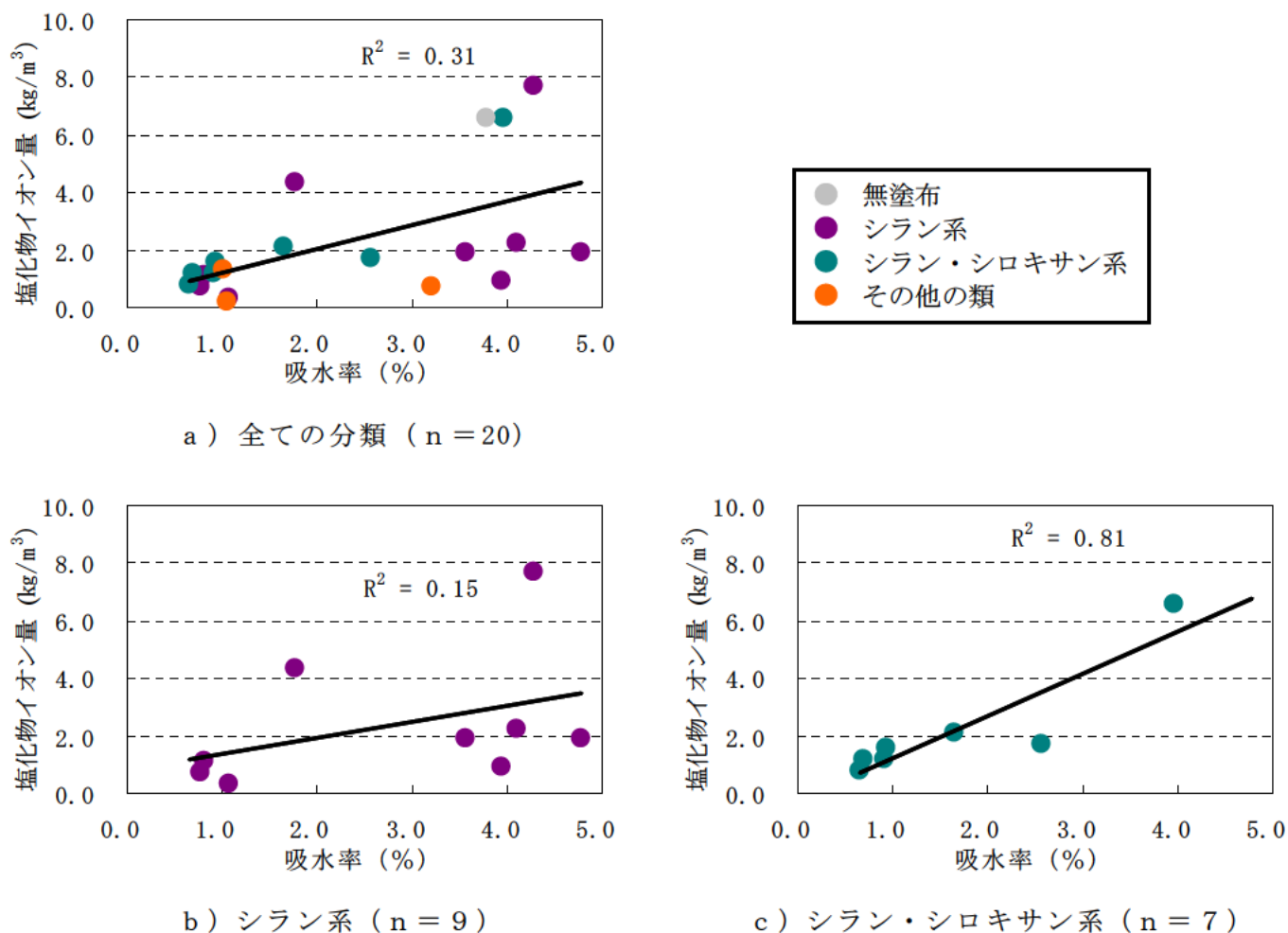
図－Ⅲ.2.56 吸水率 (45 日後) と塩化物イオン量
