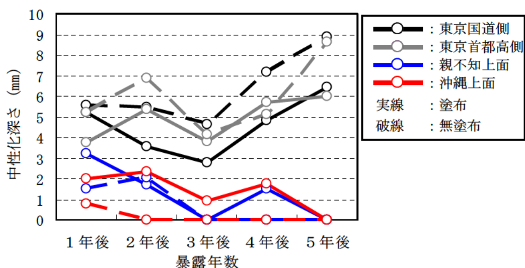
図－Ⅲ. 1. 132 その他の類 単独形の平均中性化
