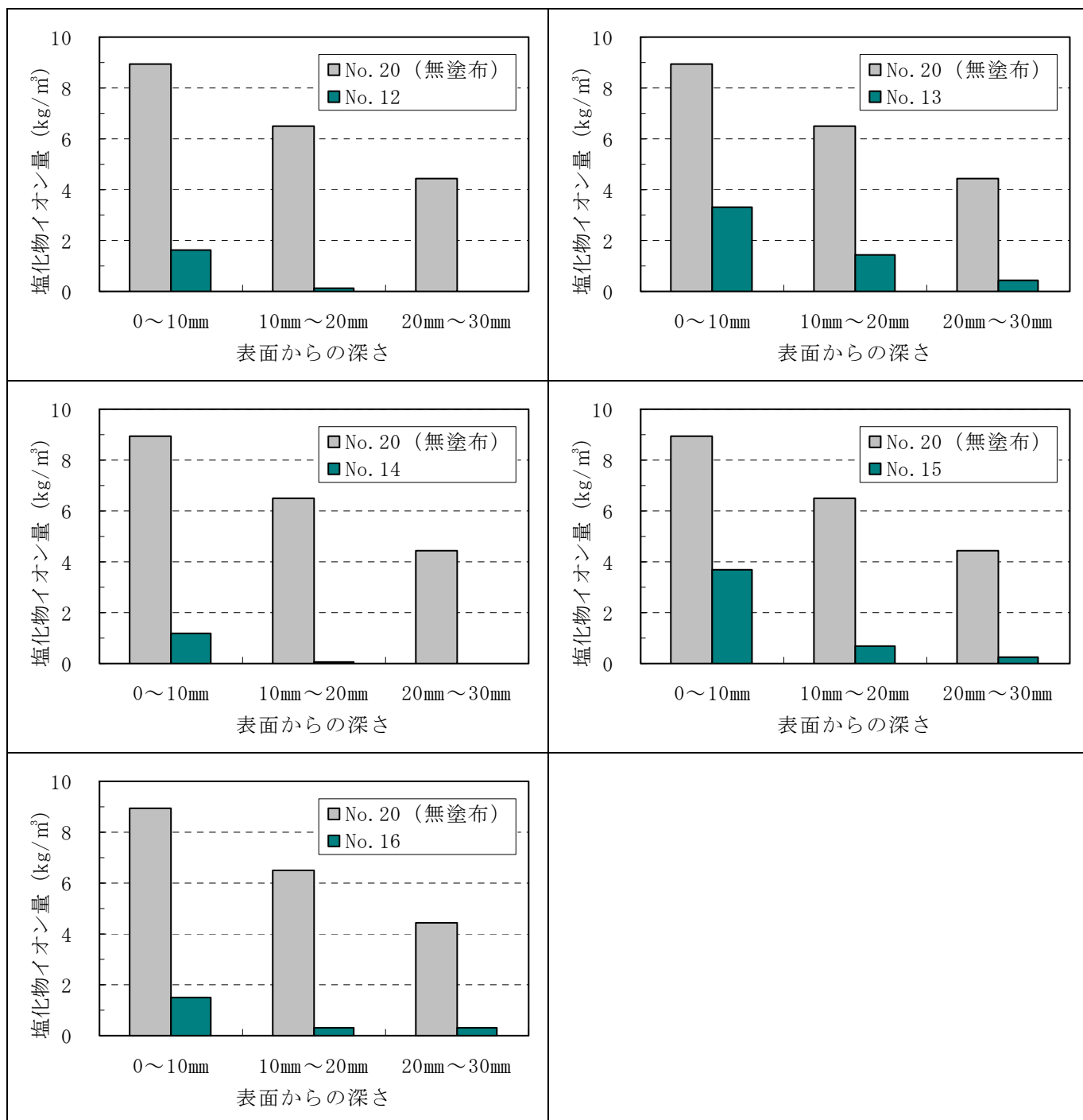
付録図－3.4.2(2) 塩化物イオン量（シラン・シロキサン系）
