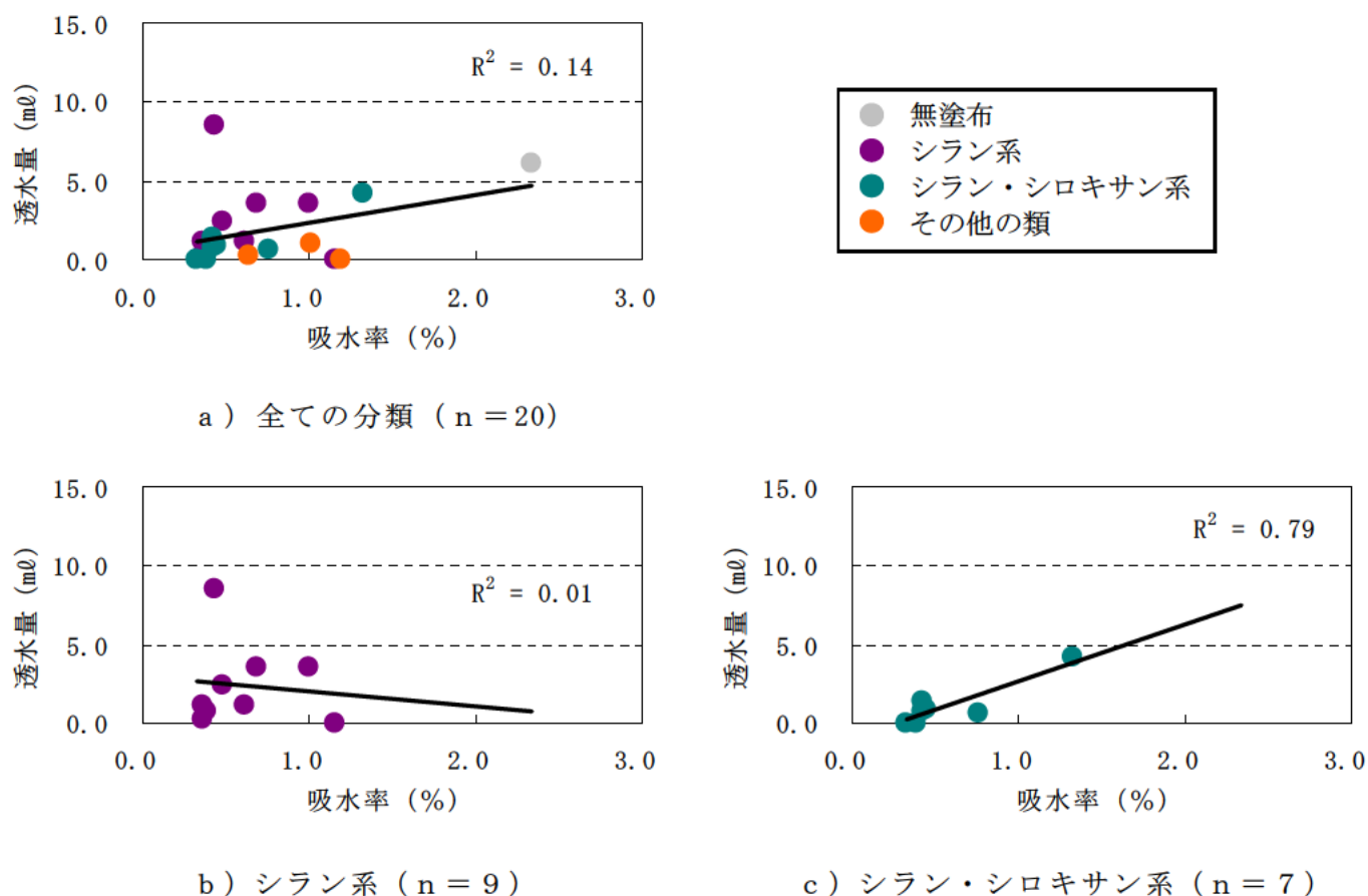
図－Ⅲ.2.30 100 mm×100 mm×60 mm（2面塗布）の吸水率と透水量（室内試験）
