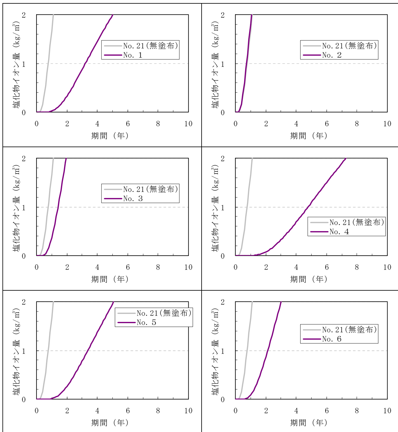
付録図－1.6.4(1) 促進試験での耐久性予測（シラン系）
