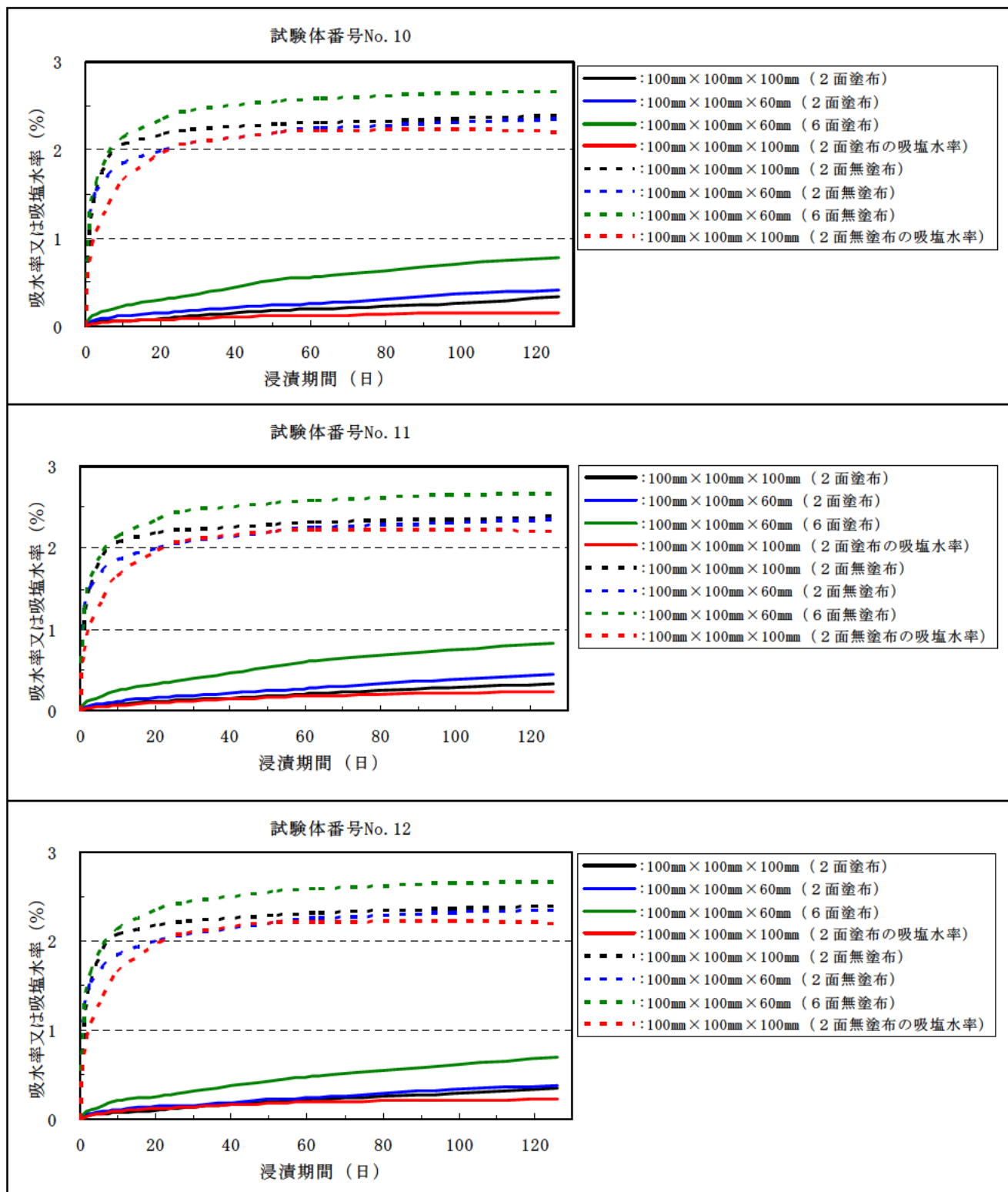
付録図－3.3.2(1) 浸漬 126 日の測定結果 (シラン・シロキサン系)
