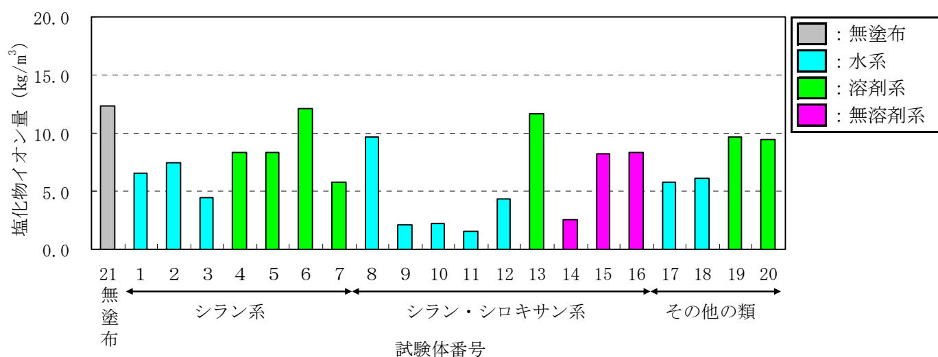
a) 上面の塩化物イオン量
