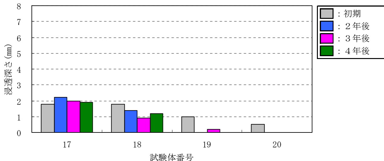
図－Ⅲ．１．６８ その他の類の浸透深さ
