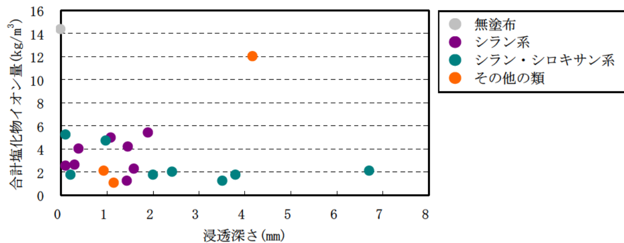
図－Ⅲ.2.16 浸透深さと塩化物イオン量 (n=20)
