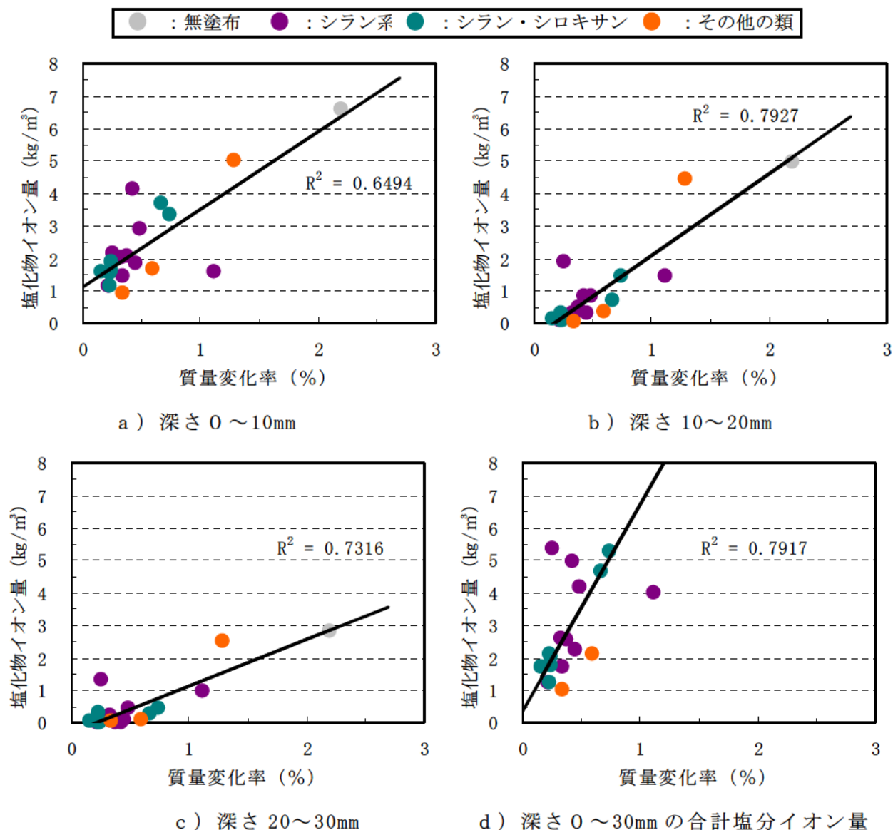
図－Ⅲ. 2. 42 質量変化率と塩化物イオン量との関係 (n = 20)
