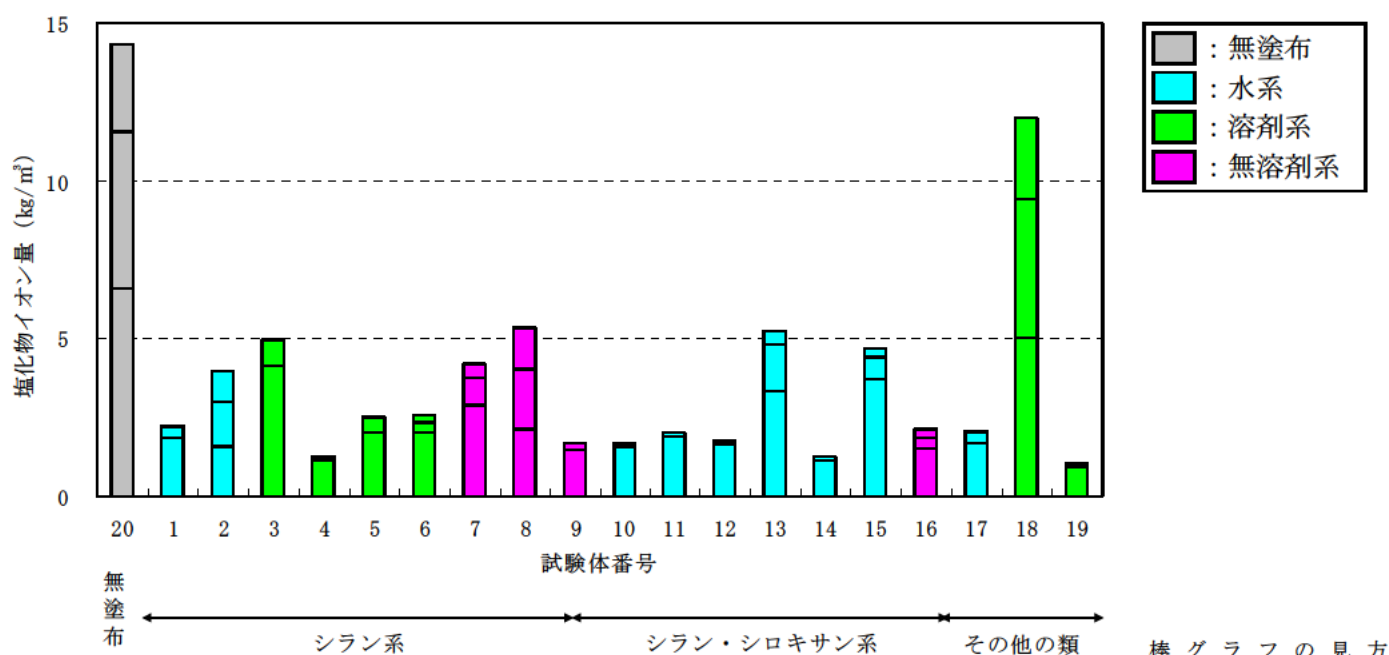
図－Ⅲ. 2. 36 塩化物イオン量 (浸漬 126 日)
