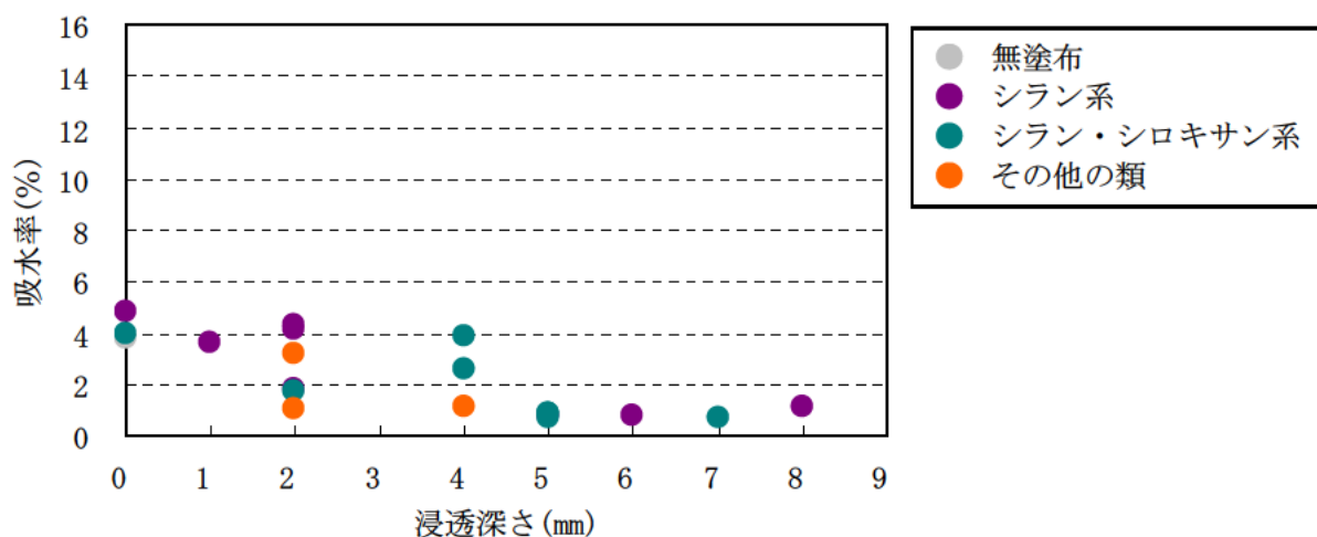
図－Ⅲ. 2. 51 浸透深さと吸水率 ( n = 20 )
