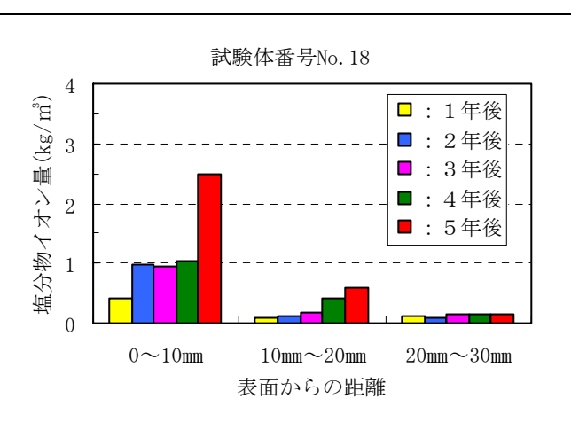
付録図－2.6.3(3) 塩化物イオン量測定結果（シラン・シロキサン系）
