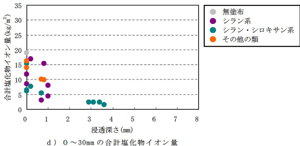
図－Ⅲ.1.72 浸透深さと塩化物イオン量 (n = 21)
