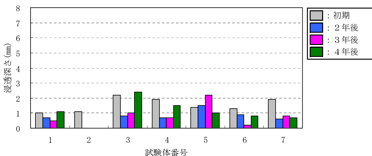
図－Ⅲ．１．６６ シラン系の浸透深さ
