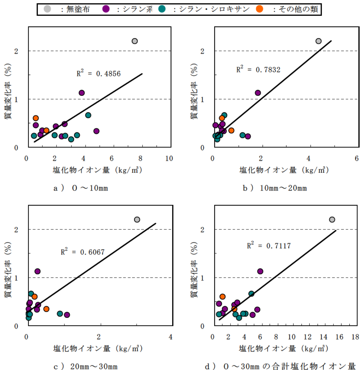
図－Ⅲ.2.77 暴露3年の塩化物イオン量と質量変化率(%)との関係 (n=17)
