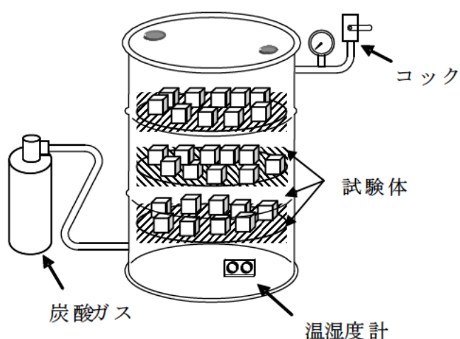
図-Ⅲ.1.11 促進中性化試験装置の概略図
