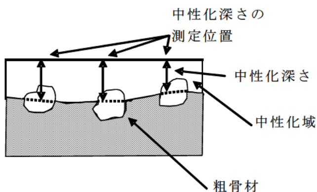
図－Ⅲ.1.13 測定箇所に粗骨材がある場合の測定方法
