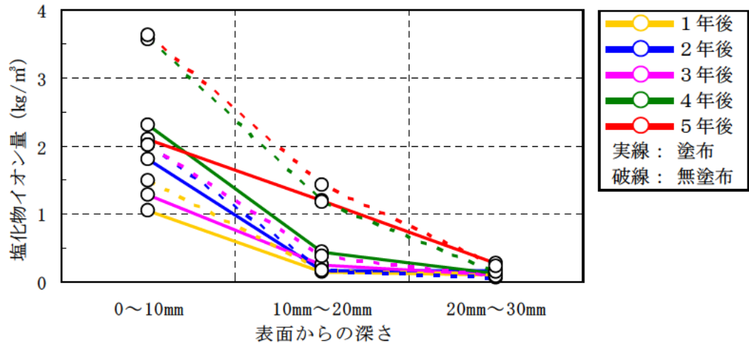
図－Ⅲ.1.101(2) その他の類（溶剤系）の塩化物イオン量測定結果
