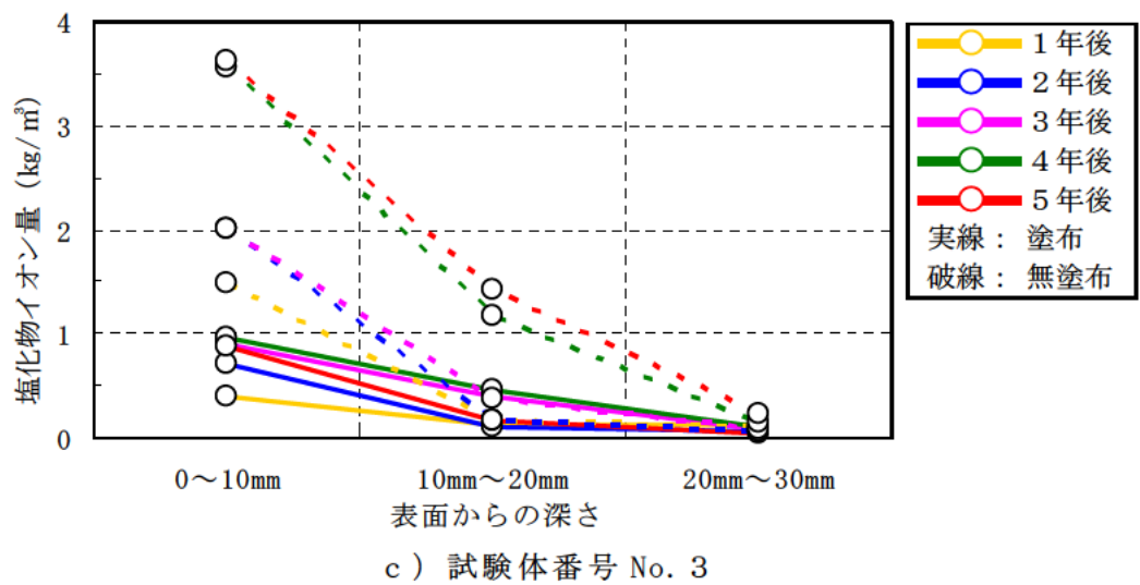
図－Ⅲ.1.99(1) シラン系（水系）の塩化物イオン量測定結果
