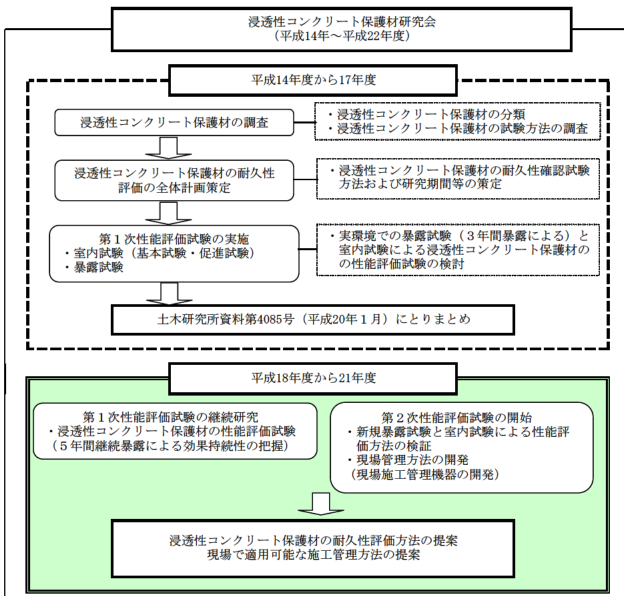
図－Ⅱ.1.1 浸透性コンクリート保護材の全体研究フロー
