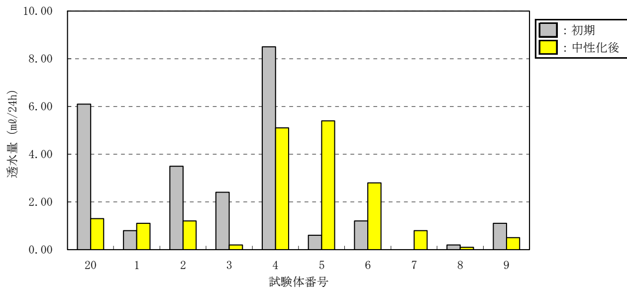
図－Ⅲ．2.17 シラン系の透水量
