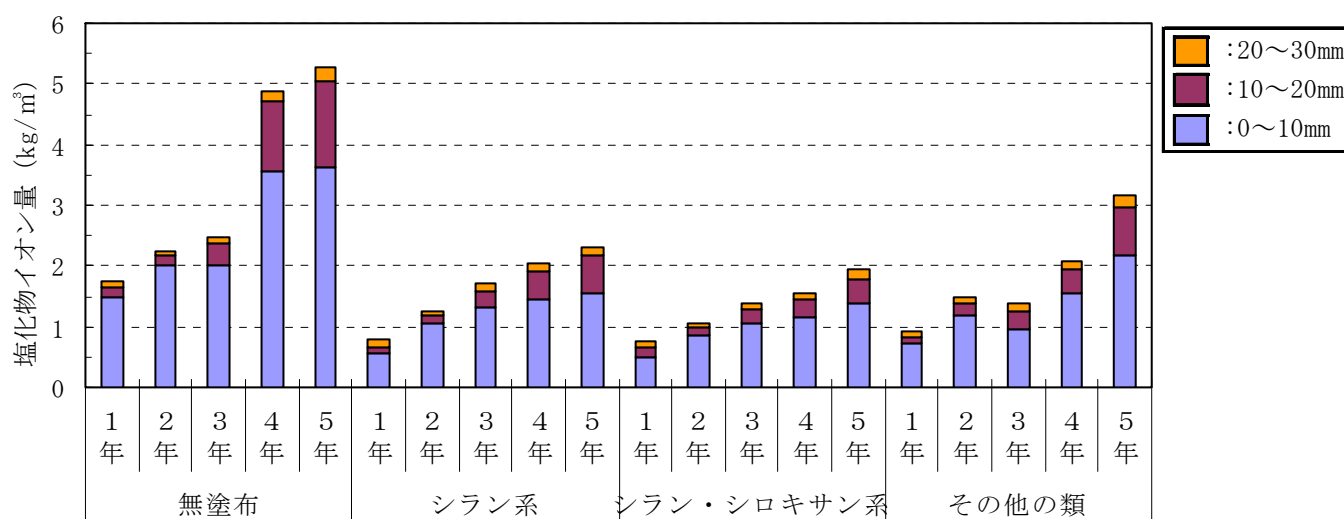
図-Ⅲ.1.98 分類別の各種保護材の平均塩化物イオン量
