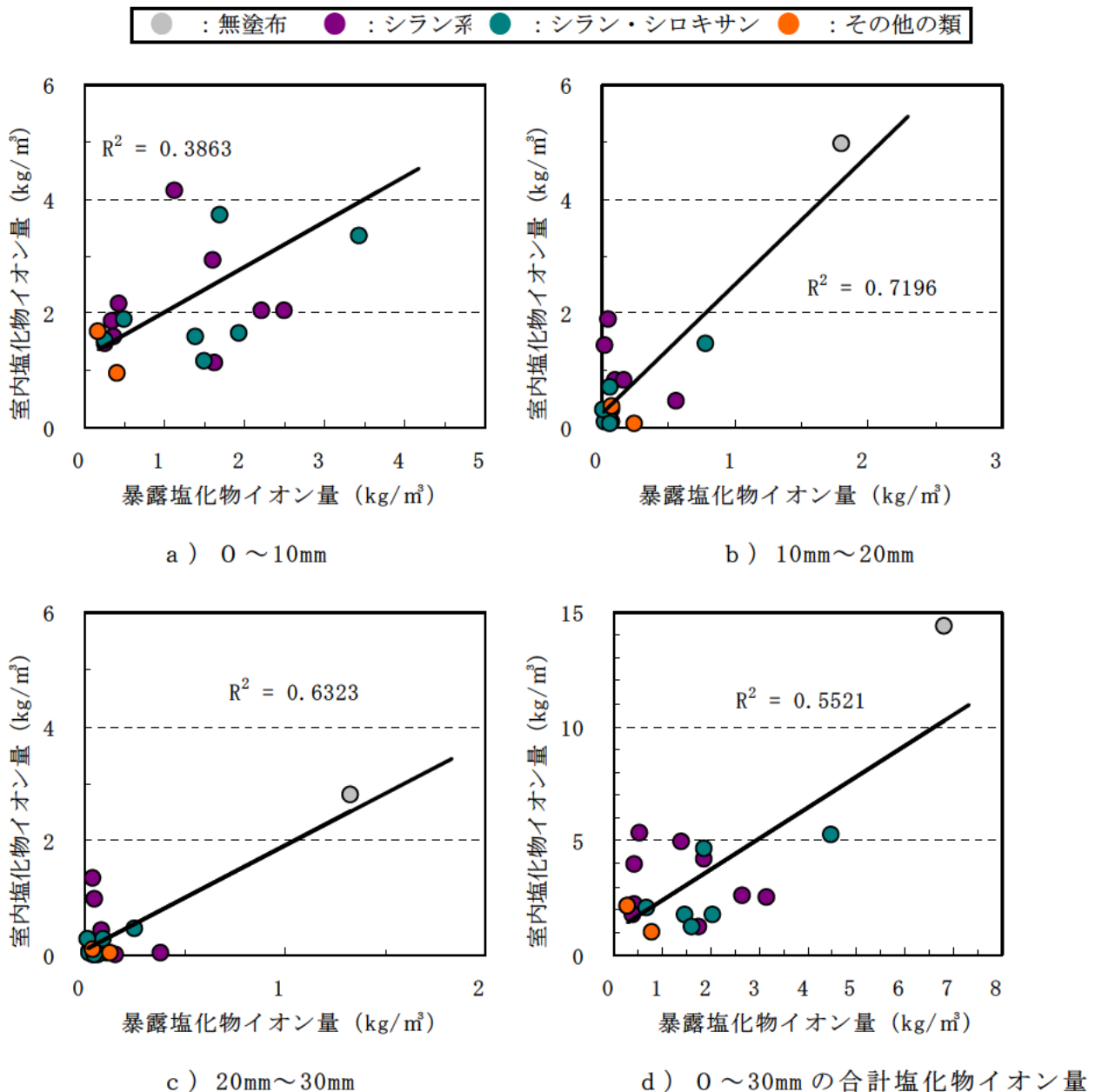
図－Ⅲ. 2. 72 暴露 1 年と室内塩化物イオン量との関係 ( n = 19 )
