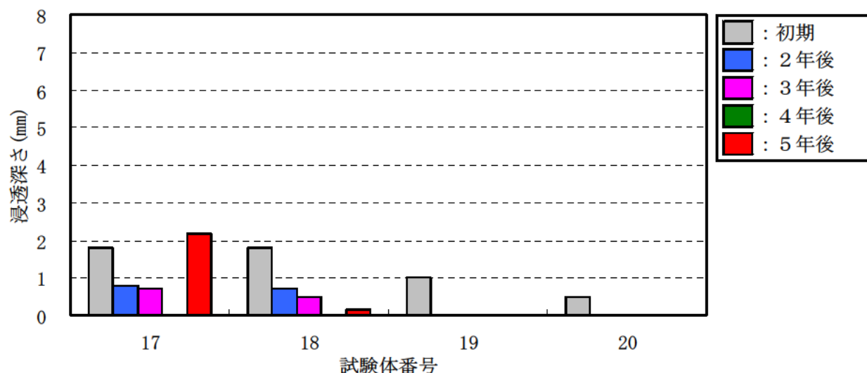
図-Ⅲ.1.71 その他の類の浸透深さ
