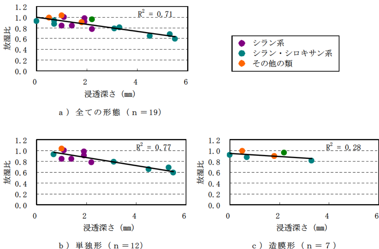
図－Ⅲ.1.24 放湿比と浸透深さ
