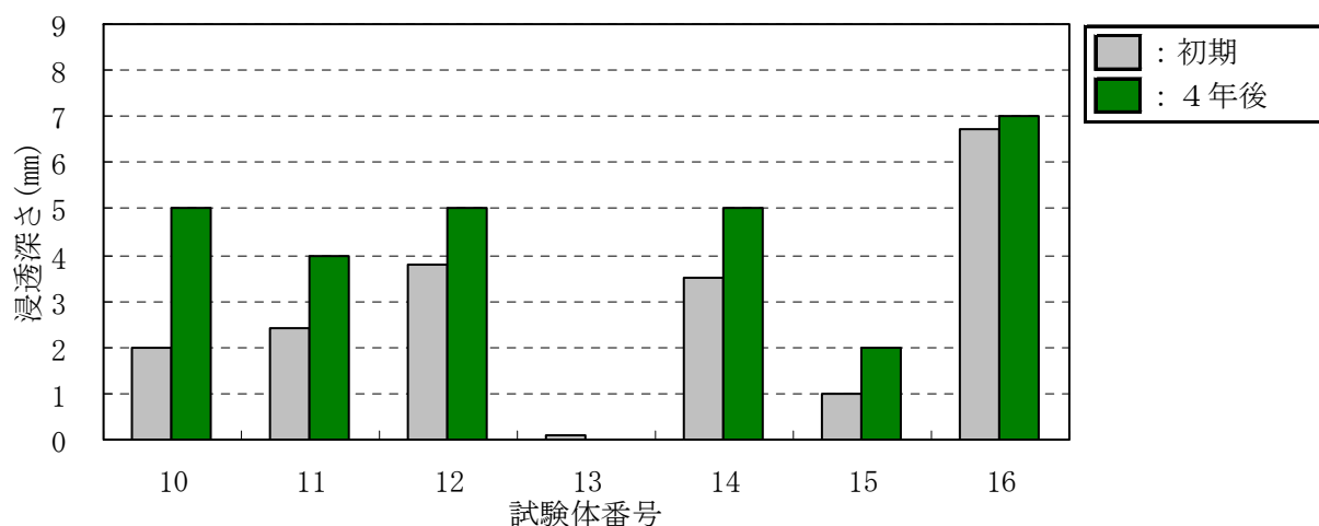
図－Ⅲ.2.49 シラン・シロキサン系の浸透深さ
