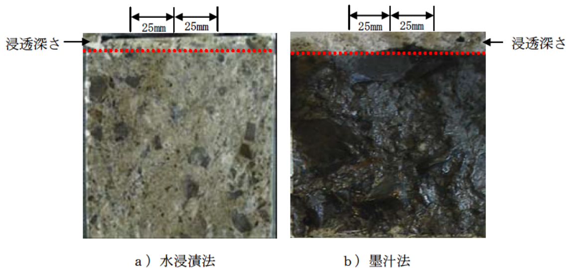
写真－Ⅲ. 1. 10 水浸漬法と墨汁法による浸透深さ
