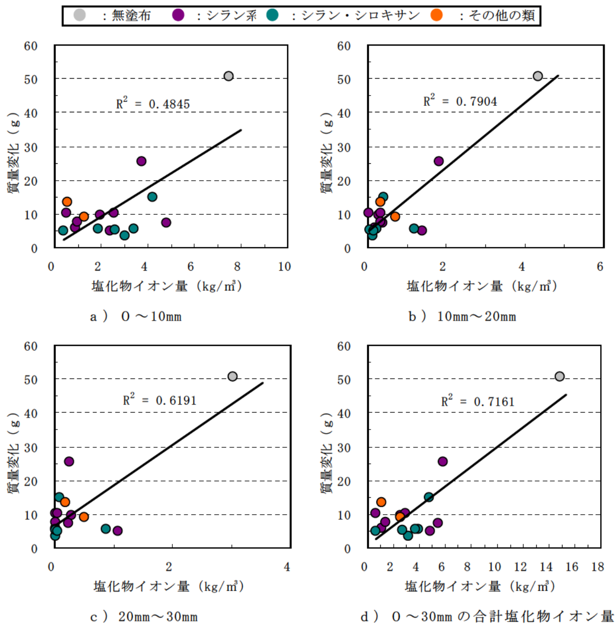
図一Ⅲ.2.76 暴露1年の塩化物イオン量と質量変化 (g) との関係 (n=17)
