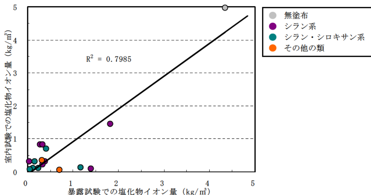
図-V.2.1 暴露試験での塩化物イオン量と室内試験での塩化物イオン量との関係 ( n = 16 )
