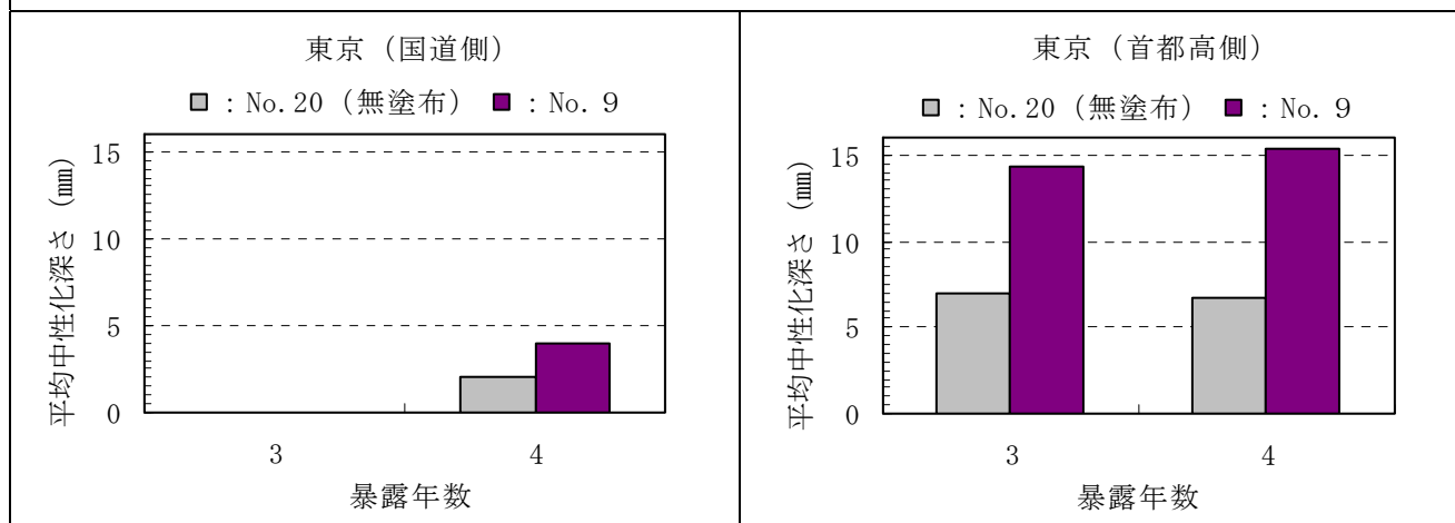
付録図－4.4.1(4) 中性化深さ測定結果（シラン系）
