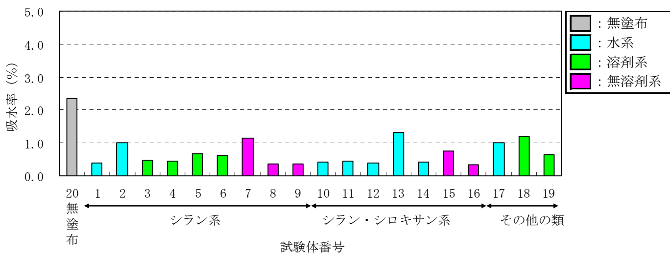
図－Ⅲ．2.23 100 mm×100 mm×60 mm（2面塗布）の吸水率
