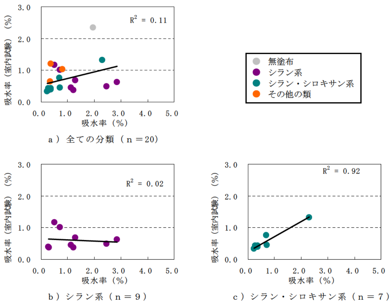
図－Ⅲ.2.57 吸水率（7日後）と吸水率（室内試験）
