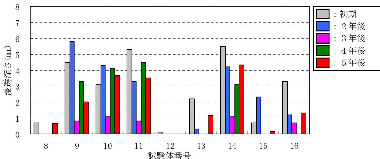
図－Ⅲ．1．63 シラン・シロキサン系の浸透深さ(首都高側)
