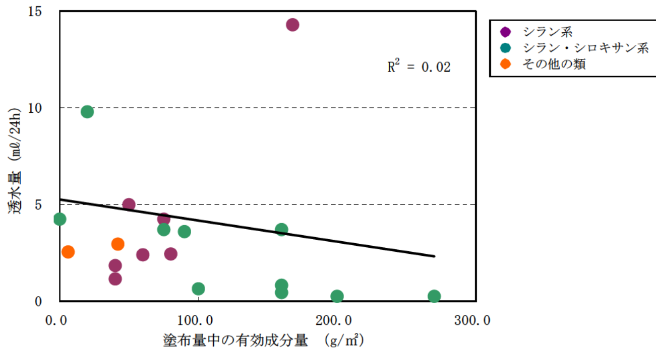
図－Ⅲ．1.85 暴露３年後の透水量と有効成分との関係（ n = 20 ）
