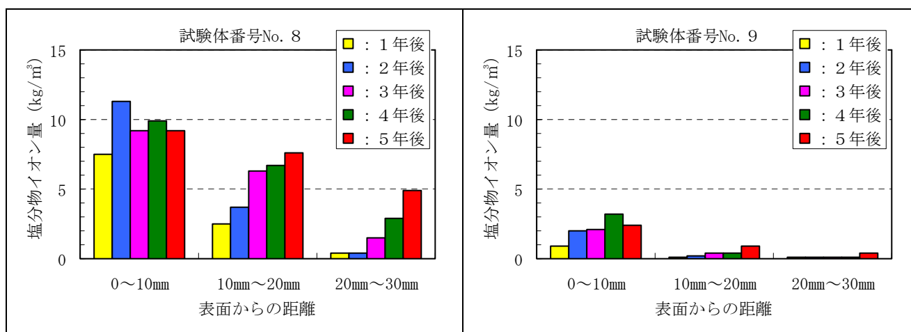
付録図－2.6.7(1) 塩化物イオン量測定結果（シラン・シロキサン系）
