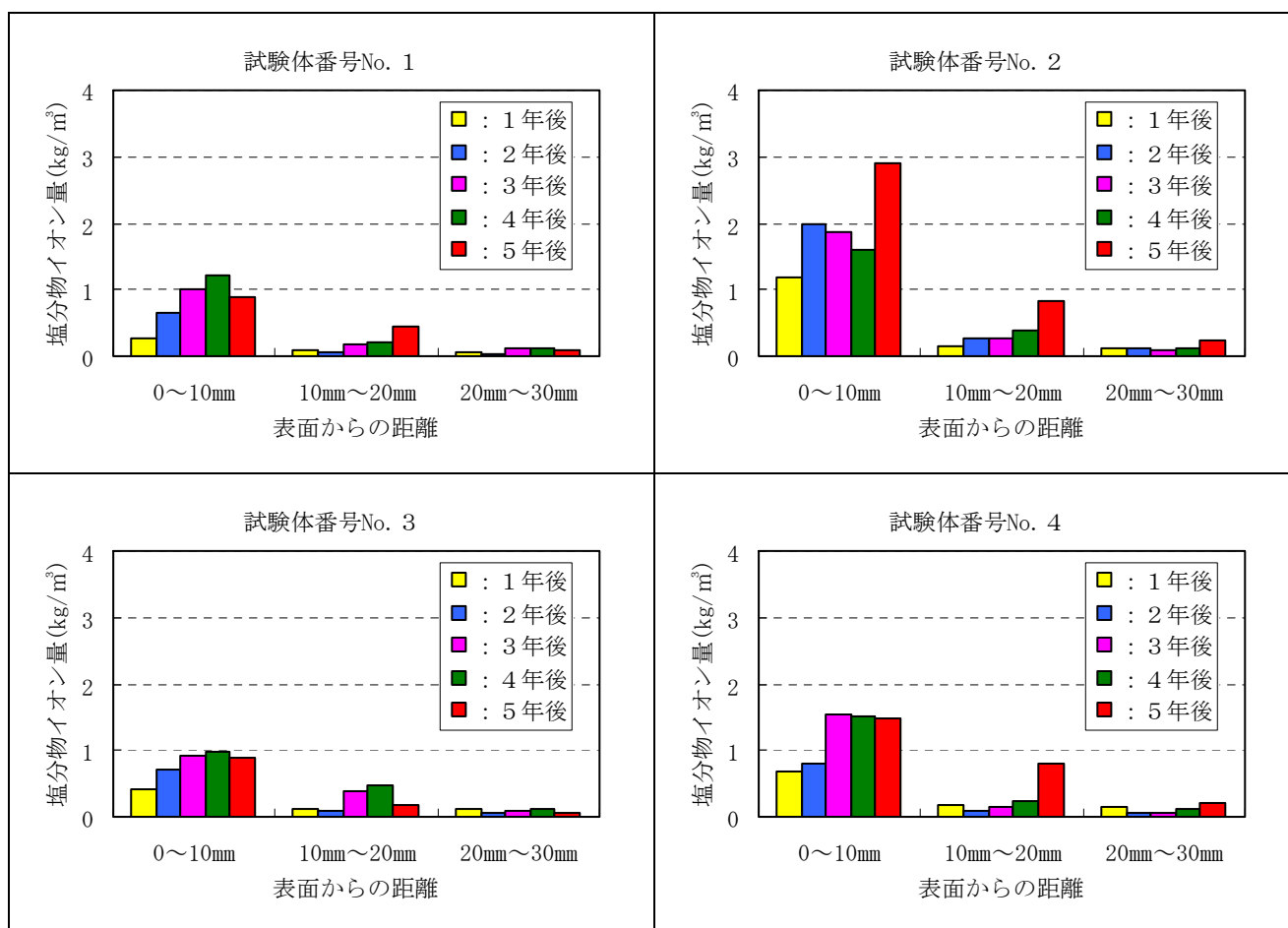
付録図－2.6.2(1) 塩化物イオン量測定結果 (シラン系)
