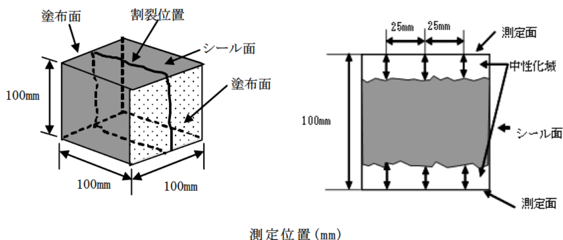
測定位置 (mm) 付属図－9.2 中性化の測定方法
