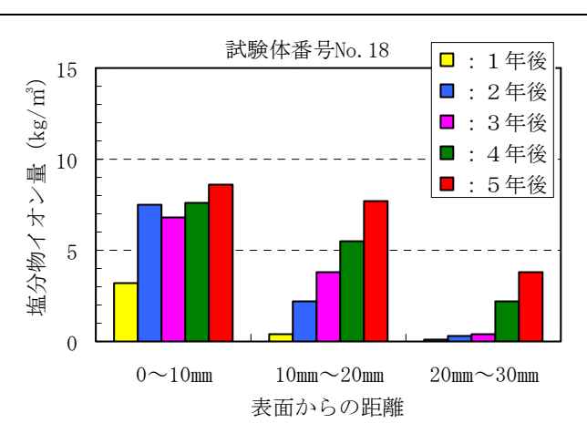
付録図－2.6.7(3) 塩化物イオン量測定結果（シラン・シロキサン系）
