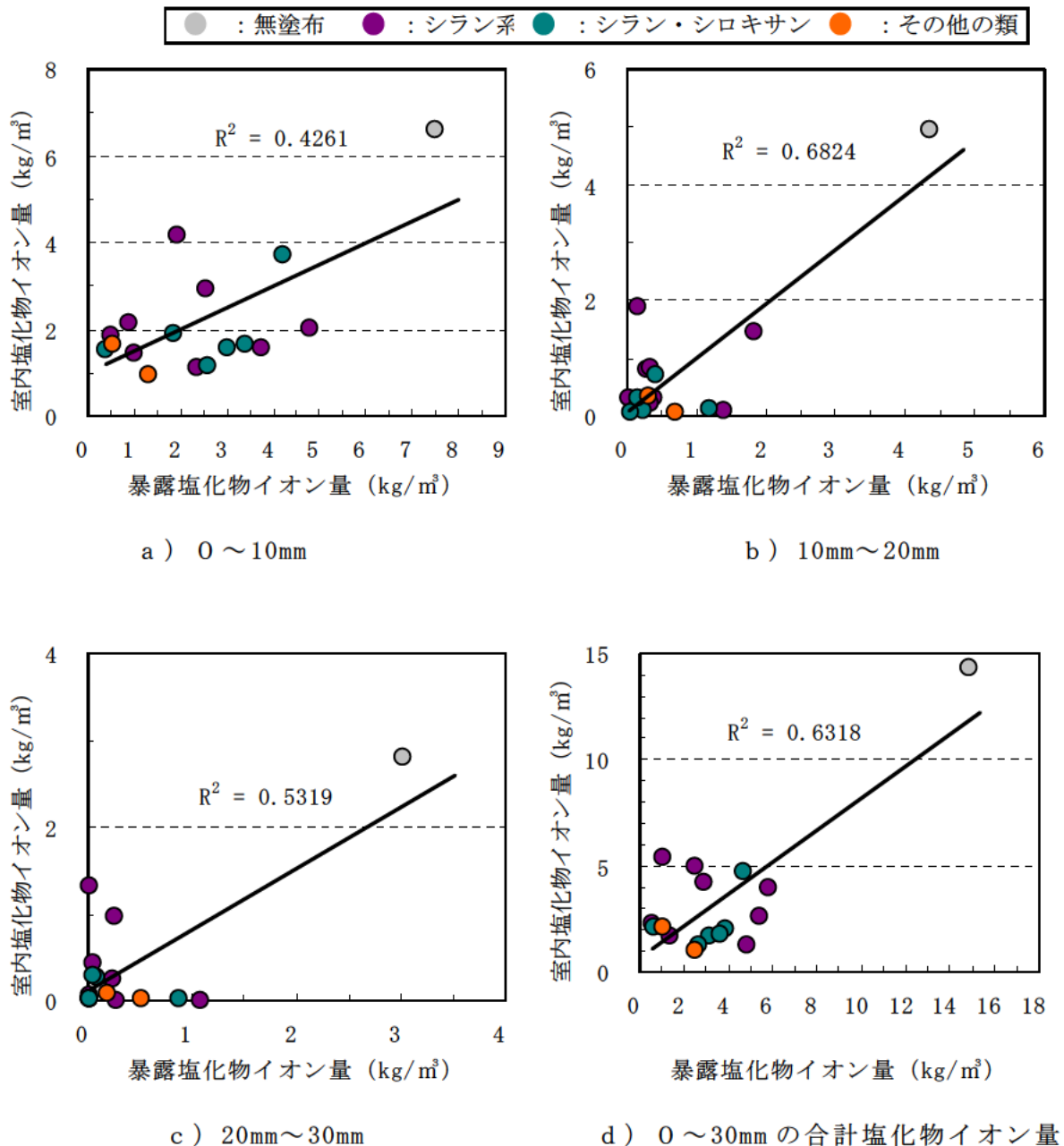
図－Ⅲ. 2. 73 暴露 3 年と室内塩化物イオン量との関係 ( n = 17 )
