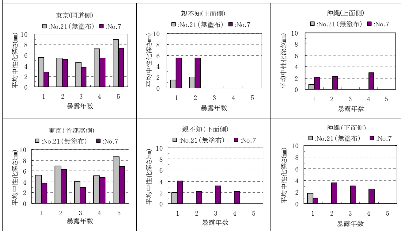
付録図－2.7.1(4) 中性化深さ測定結果（シラン系）
