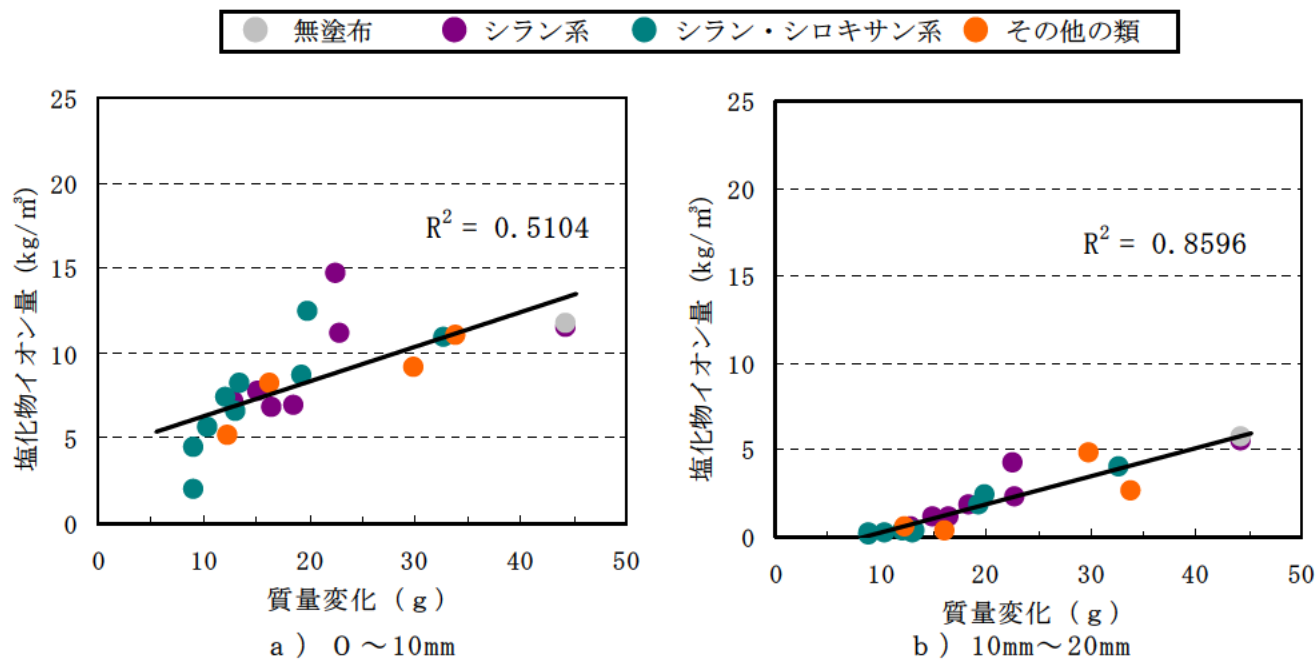
図－Ⅲ.1.43(1) 質量変化と深さ方向の塩化物イオン量との関係 (1) ( n = 21 )
