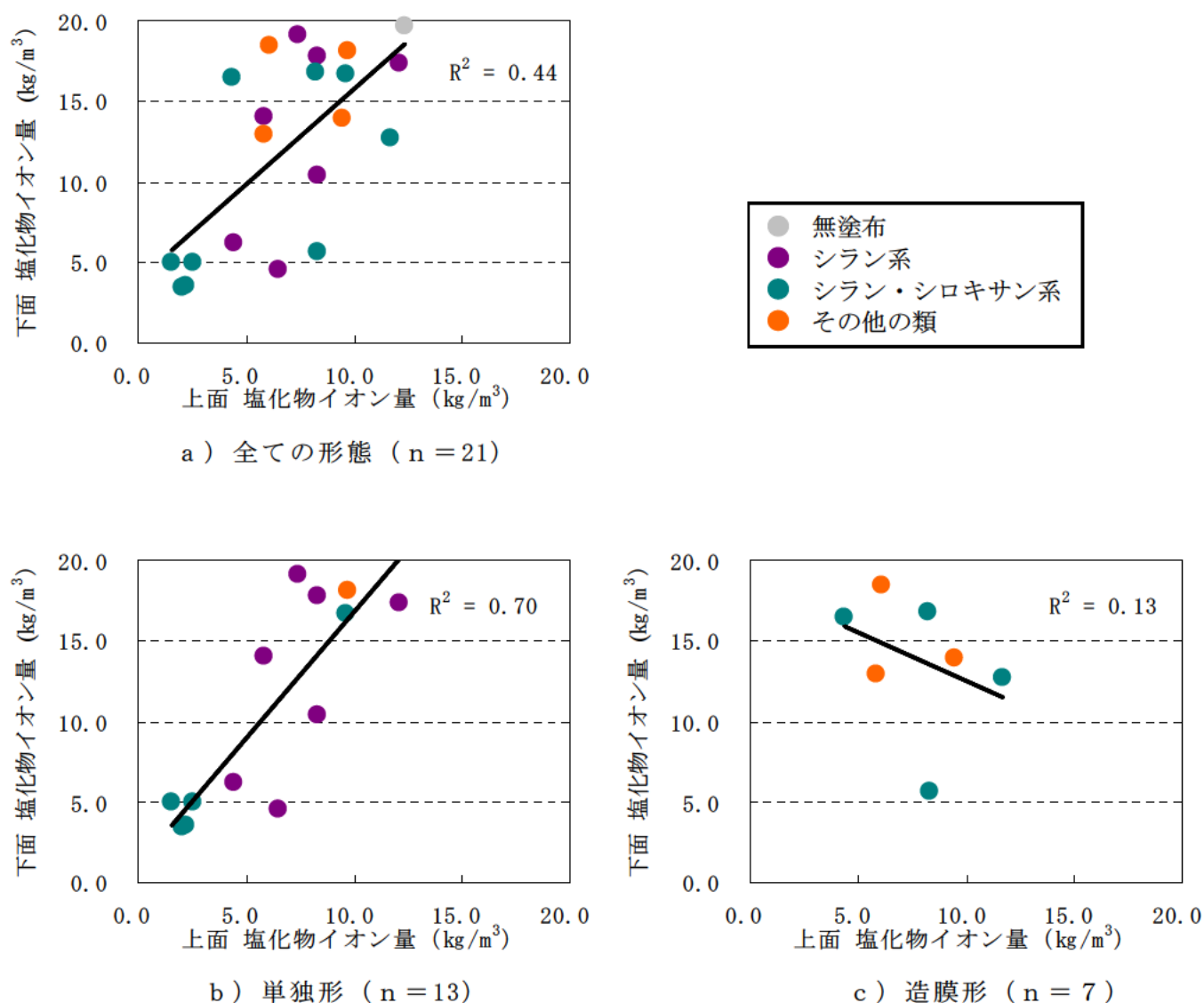
図－Ⅲ.1.140 上面の塩化物イオン量と下面の塩化物イオン量
