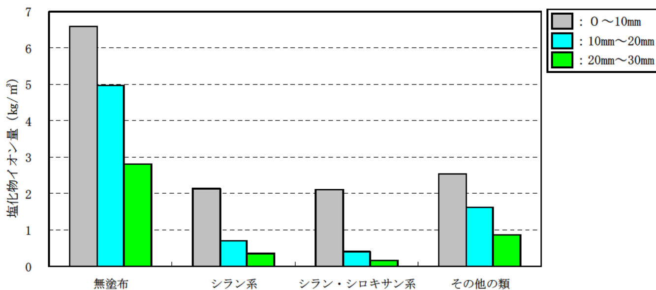
図－Ⅲ. 2. 37 分類別平均塩化物イオン量
