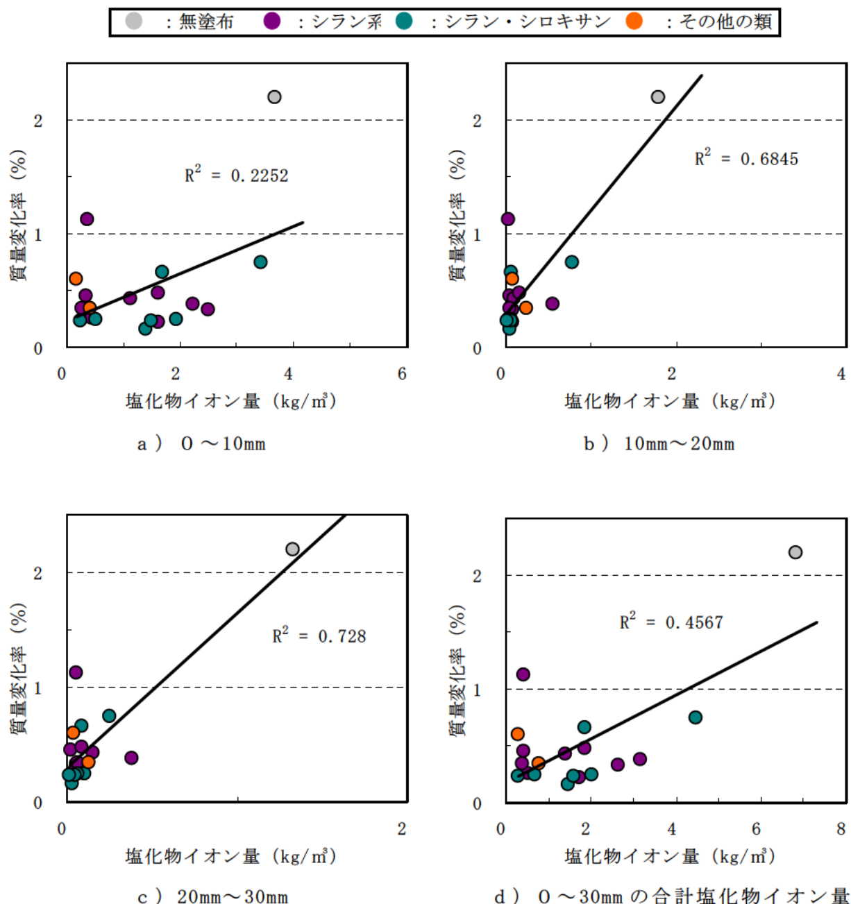
図－Ⅲ. 2. 75 暴露 1 年の塩化物イオン量と質量変化率 (%) との関係 (n = 19)
