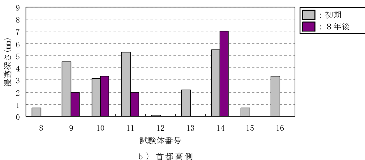
図－Ⅲ.1.135 シラン・シロキサン系の浸透深さ
