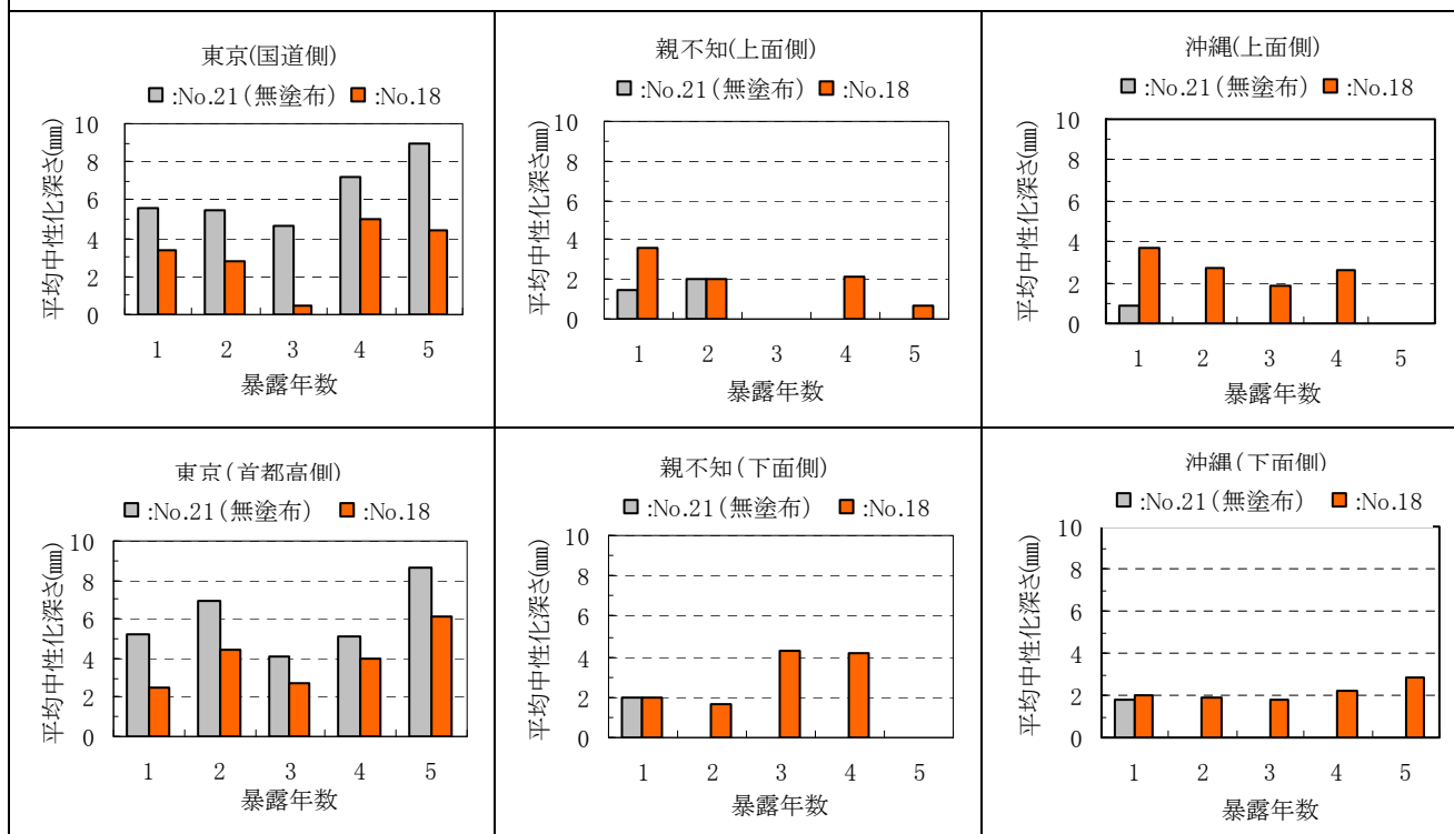
付録図－2.7.3(1) 中性化深さ測定結果（その他の類）
