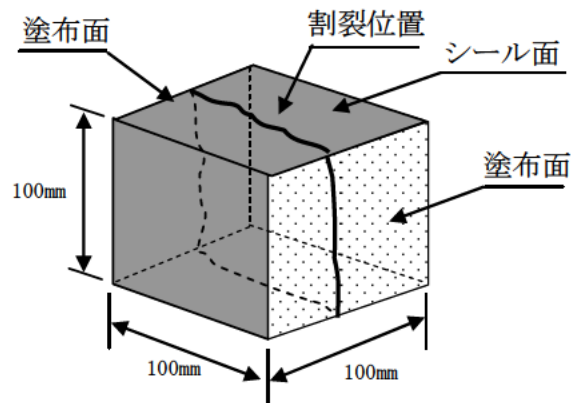
図－Ⅲ.1.9 割裂位置
