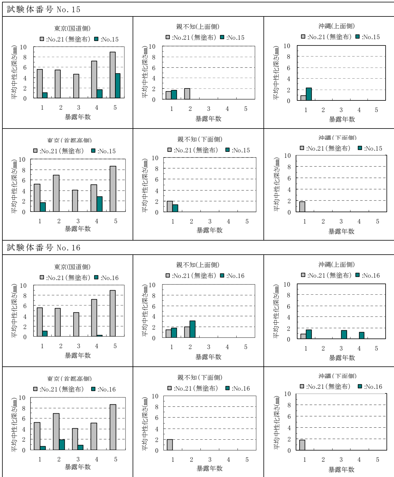
付録図－2.7.2(5) 中性化深さ測定結果（シラン・シロキサン系）
