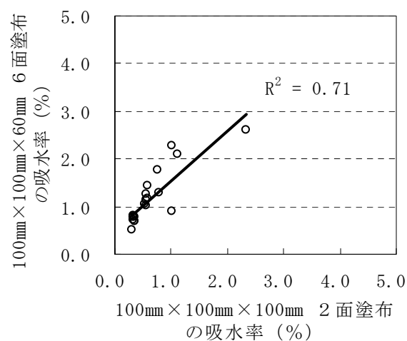
c) 試験体の大きさと塗布面数が異なる場合
