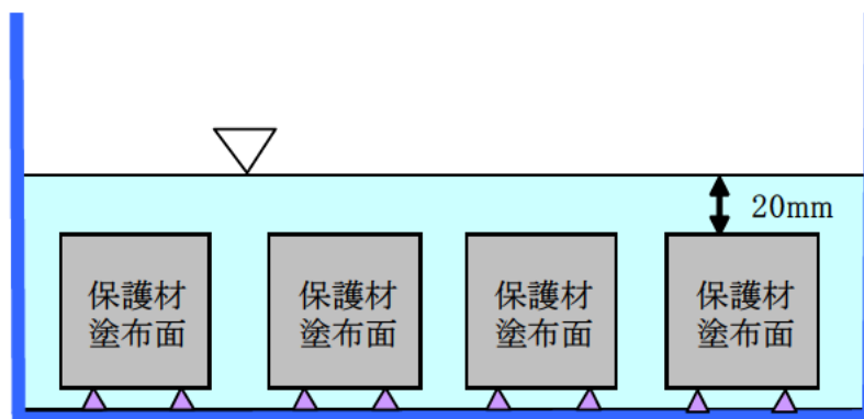
図-Ⅲ.2.44 塩化物イオン浸透性試験方法
