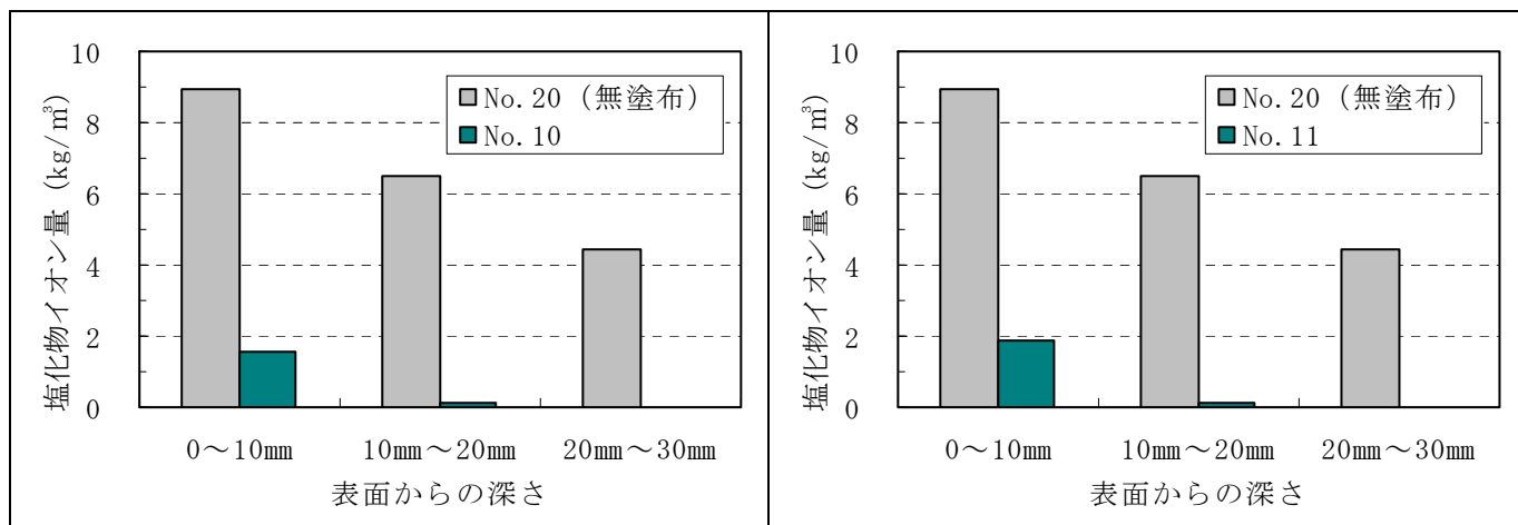
付録図－3.4.2(1) 塩化物イオン量（シラン・シロキサン系）
