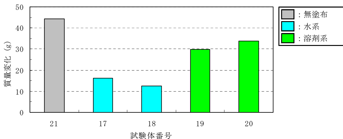
図－Ⅲ.1.30 その他の類の質量変化（浸漬 90 日）
