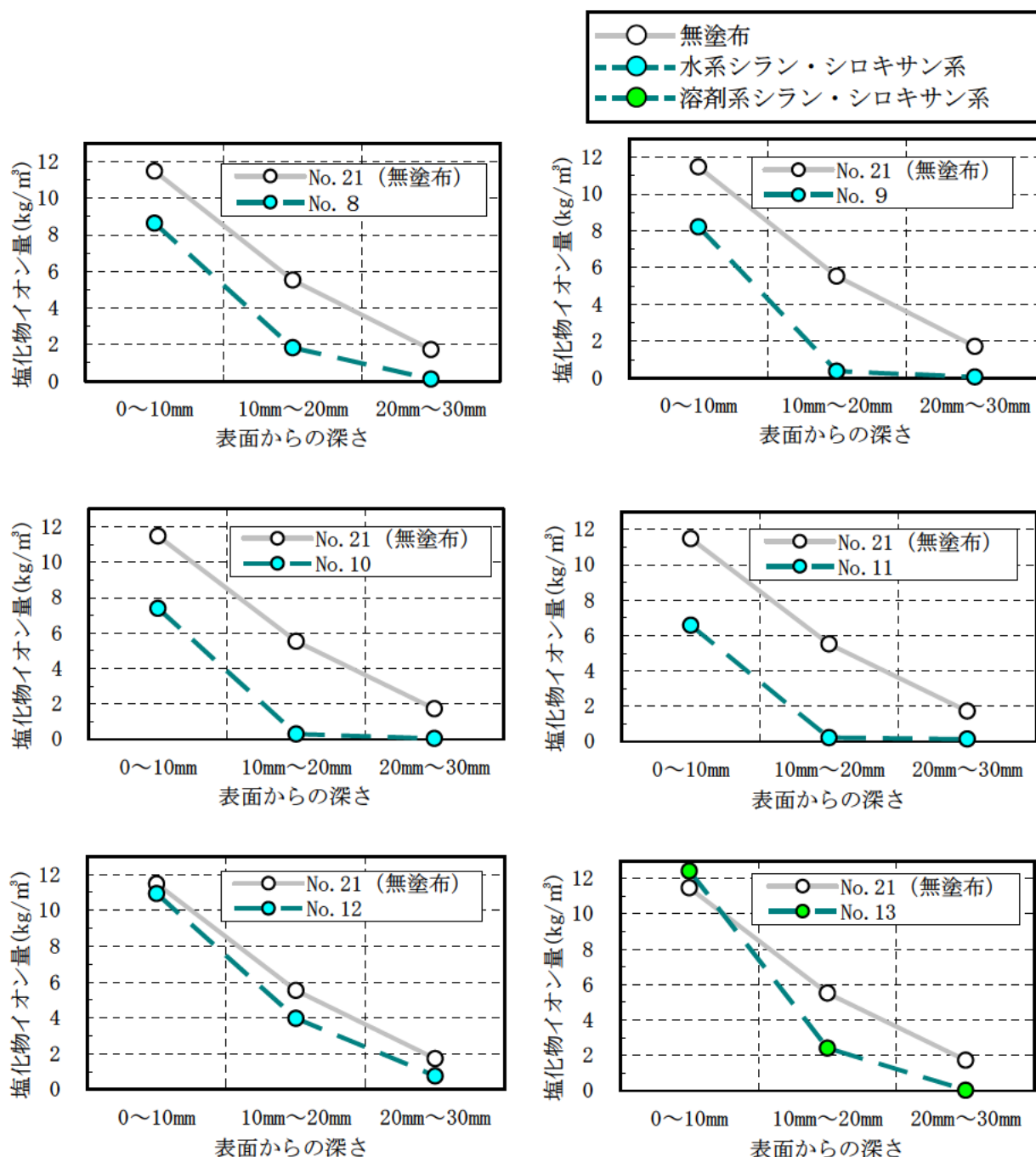
図－Ⅲ.1.39(1) シラン・シロキサン系（水系および溶剤系）の塩化物イオン量
