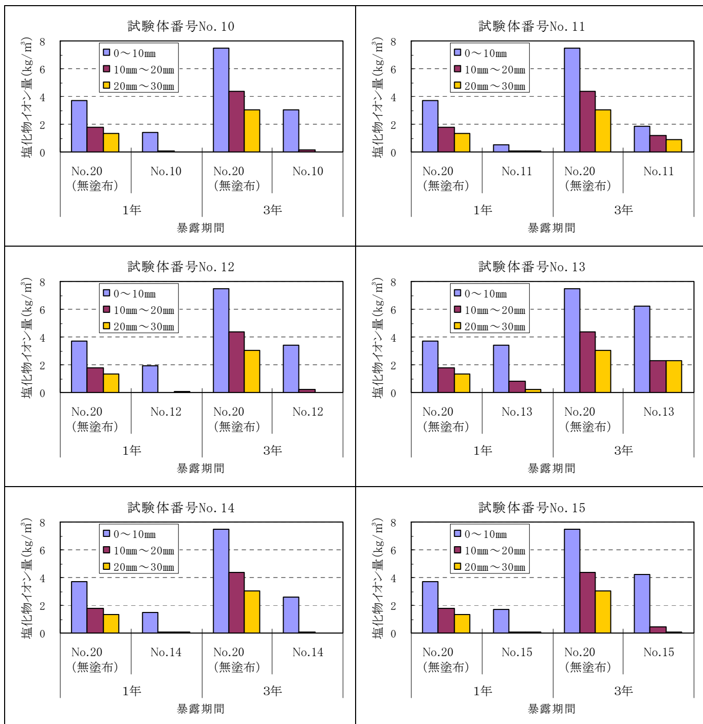
付録図－4.3.2(1) 塩化物イオン量（シラン・シロキサン系）
