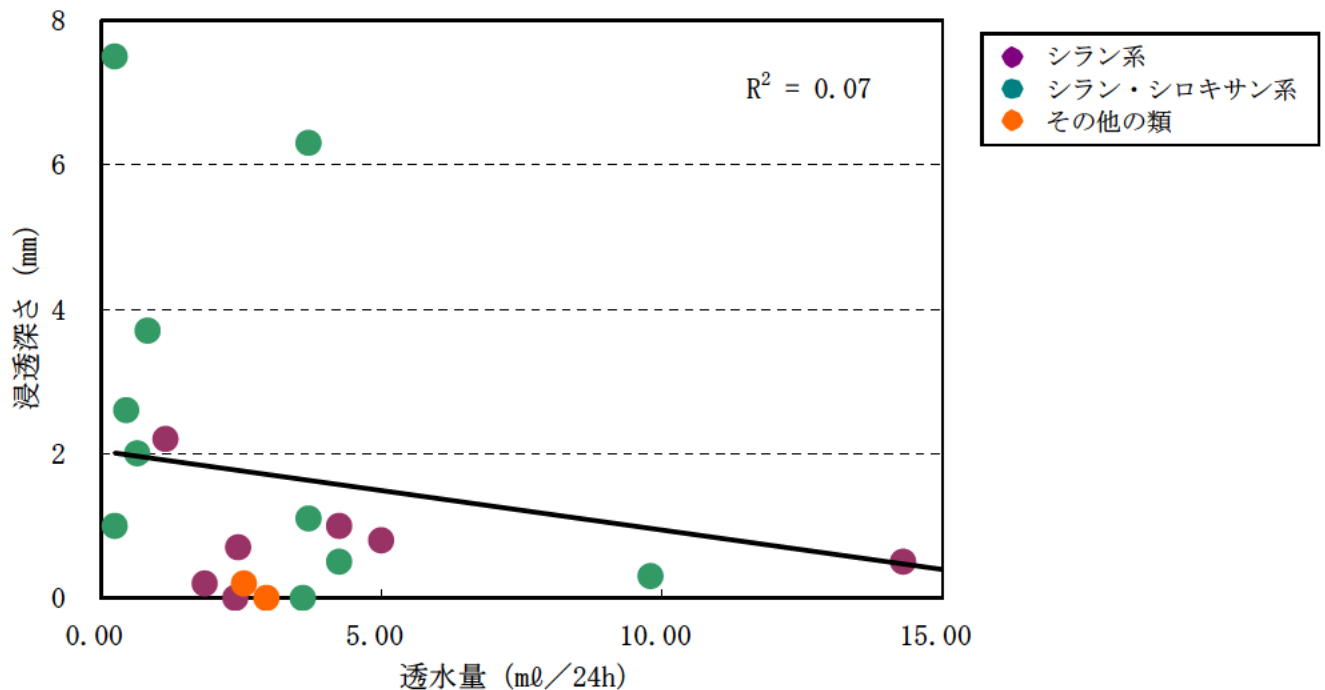
図－Ⅲ.1.88 暴露2年後の透水量と浸透深さとの関係（ n = 20 ）
