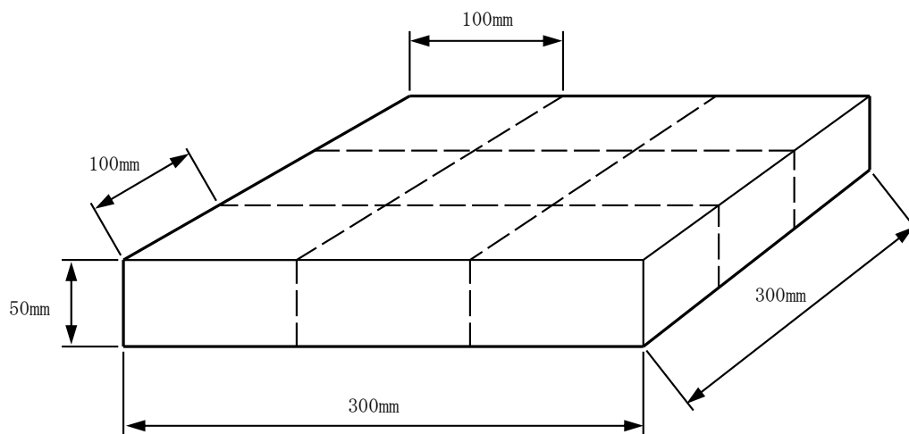
図－Ⅲ.2.2 コンクリートの切断寸法
