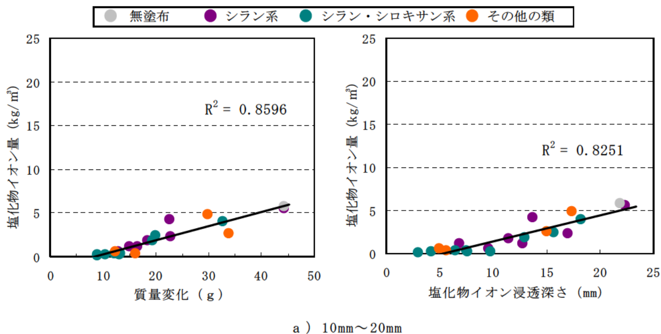
図－V.1.6 質量変化、塩化物イオンの浸透深さと塩化物イオン量との関係（n＝21）
