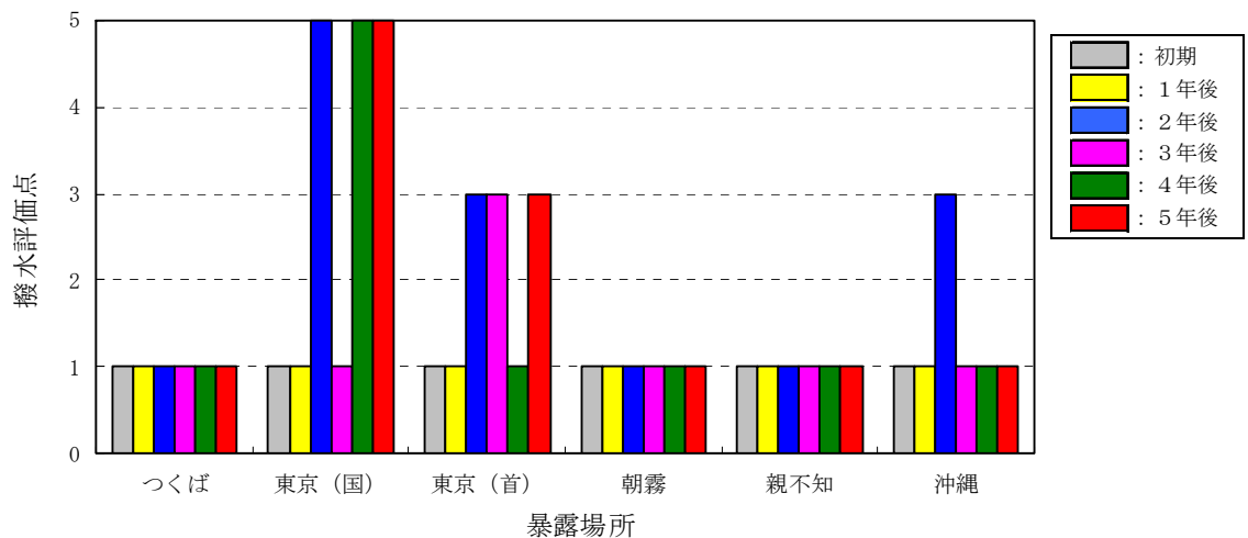
図－Ⅲ.1.59(1) 暴露場所による無塗布コンクリートの撥水評価点
