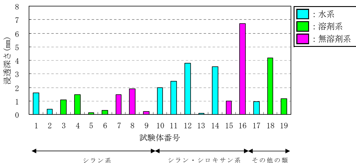
図－Ⅲ. 2. 9 全ての系の浸透深さ
