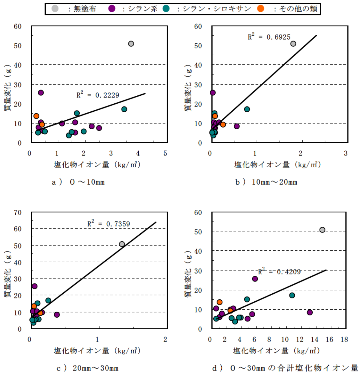
図一Ⅲ2.74 暴露1年の塩化物イオン量と質量変化 (g) との関係 (n=19)
