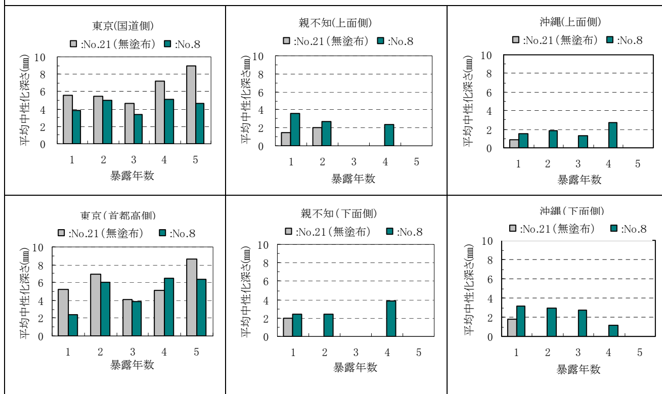
付録図－2.7.2(1) 中性化深さ測定結果（シラン・シロキサン系）
