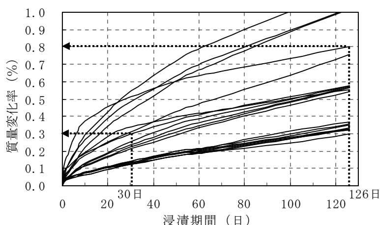
付属図解－1 浸漬期間と質量変化率の関係
