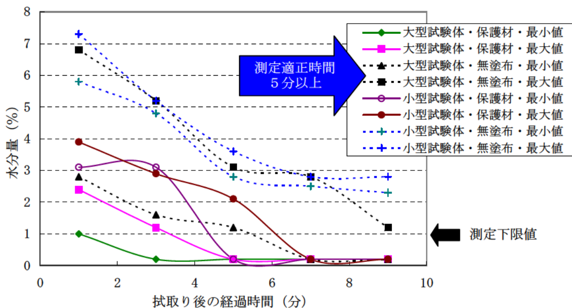
図－IV. 2. 22 適正な測定時間
