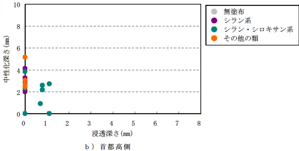
図－Ⅲ. 1. 77 浸透深さと中性化深さ (n = 21)
