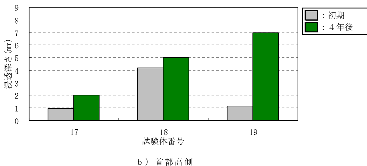
図-III.2.47 その他の類の浸透深さ
