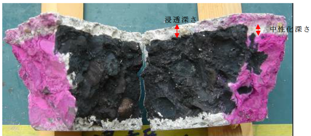
フェノールフタレイン法と墨汁法での確認
