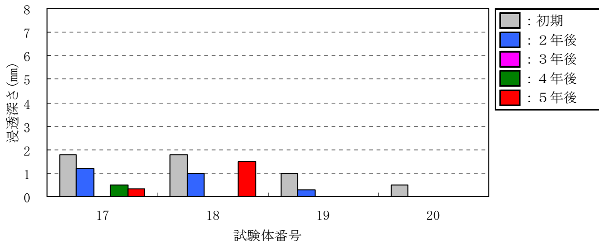
図－Ⅲ．１．６５ その他の類の浸透深さ（首都高側）
