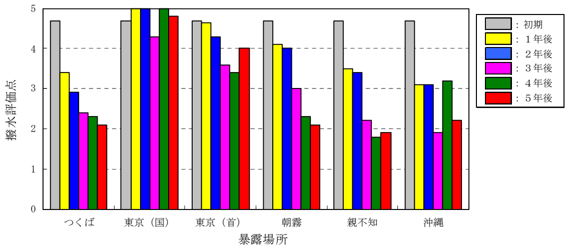
図－Ⅲ.1.59(2) 暴露場所による全試験体の撥水評価点
