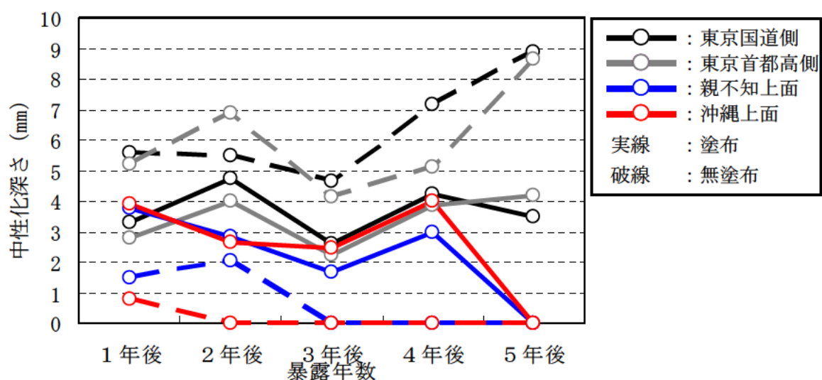
図－Ⅲ.1.130 シラン・シロキサン系 単独形の平均中性化
