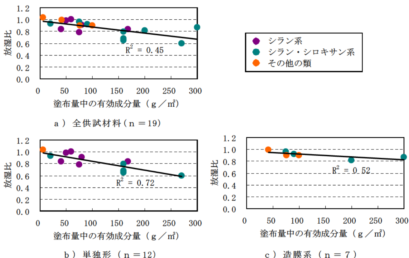
図－V.1.3 塗布量中の有効成分量と透湿性（放湿比）の関係
