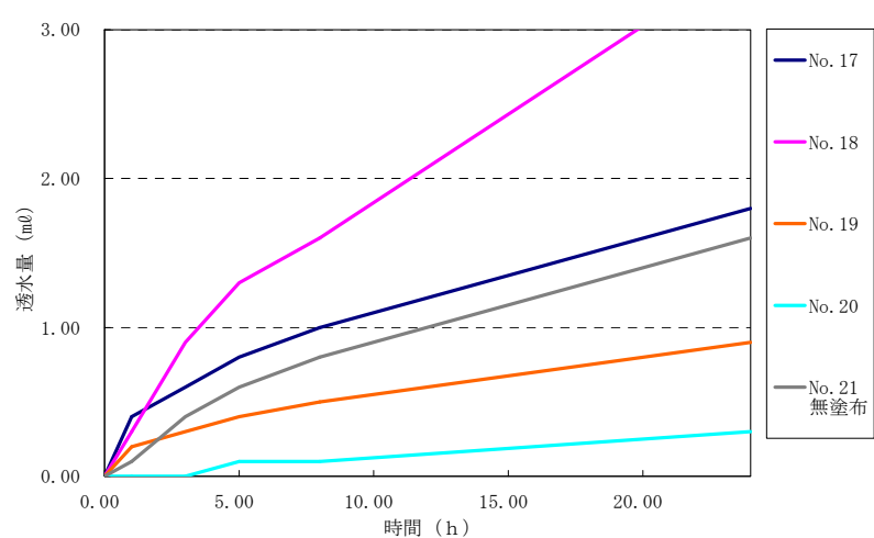
付録図－2.4.4 暴露4年後の透水量測定結果
