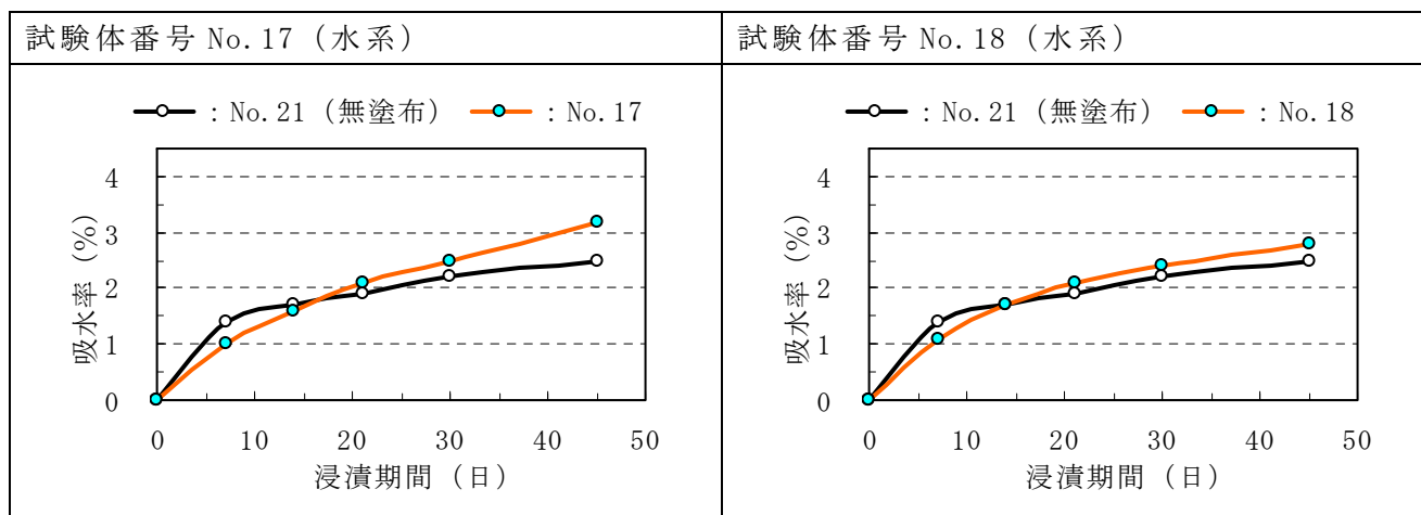
付録図－2.8.3(1) 吸水率測定結果 (その他の類)
