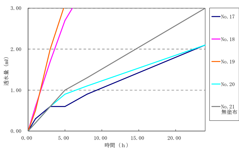
付録図－2.4.5 暴露5年後の透水量測定結果
