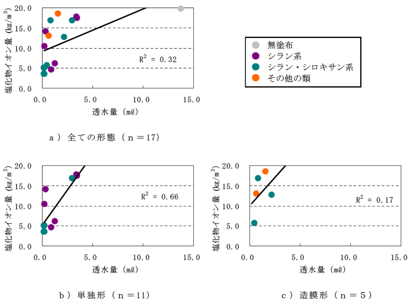
図－Ⅲ.1.146 下面の塩化物イオン量と透水量（室内試験）
