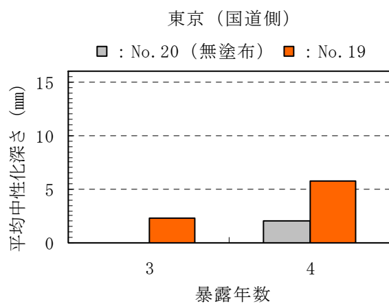
付録図－4.4.3(2) 中性化深さ測定結果 (その他の類)
