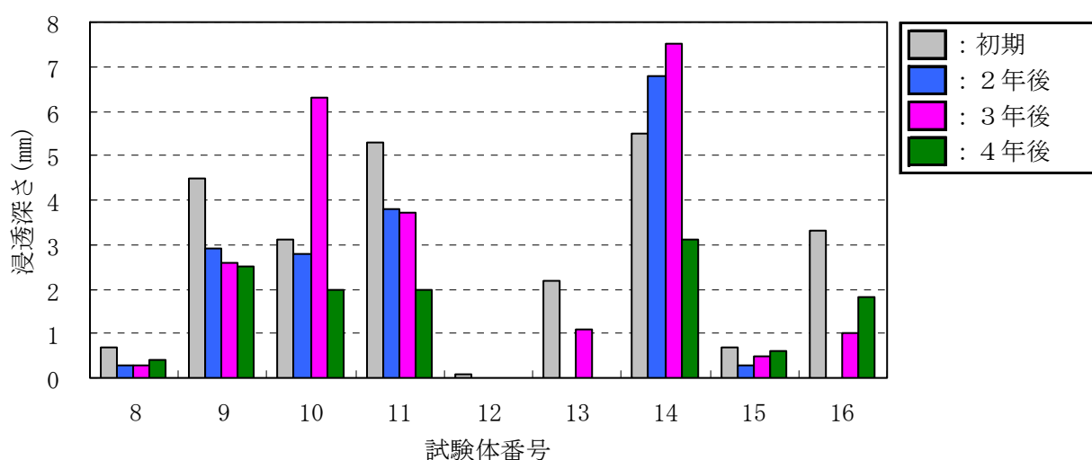
図－Ⅲ. 1. 67 シラン・シロキサン系の浸透深さ
