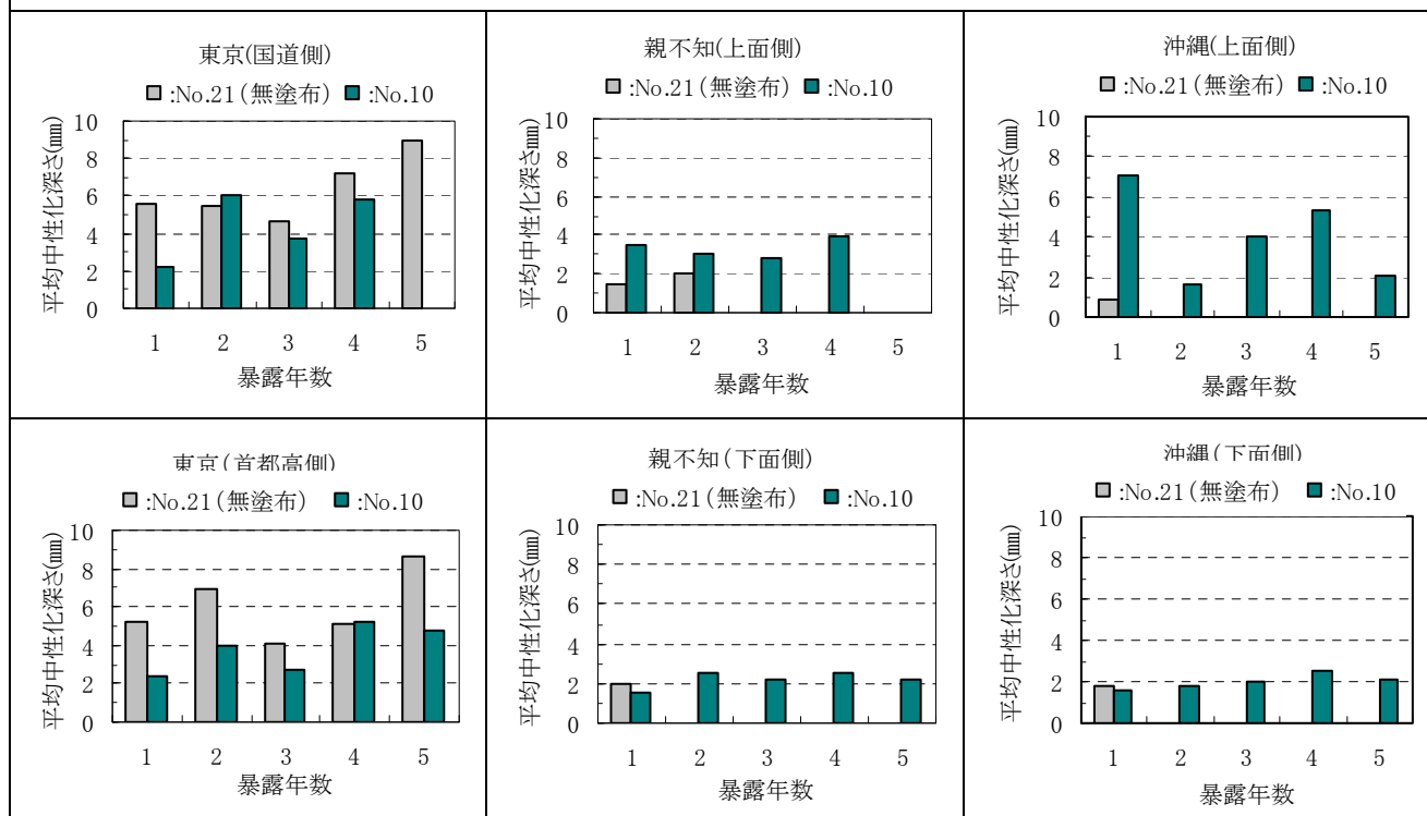
付録図-2.7.2(2) 中性化深さ測定結果 (シラン・シロキサン系)
