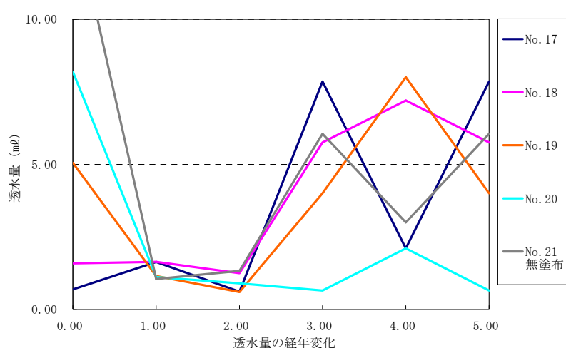
付録図－2.4.5 つくば暴露年数による24時間後の透水量変化
