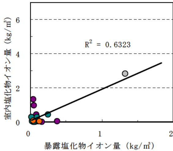
図-V.1.14 暴露1年と室内塩化物イオン量との関係 ( n=19 )
