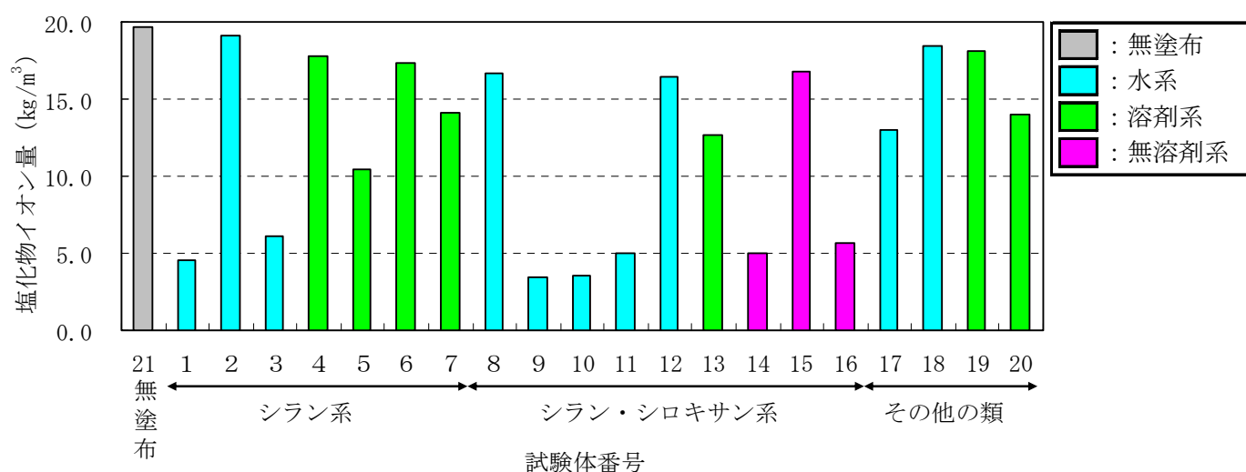
b) 下面の塩化物イオン量
