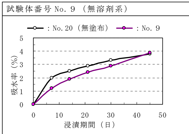
付録図－4.2.1(3) 吸水率測定結果 (シラン系)
