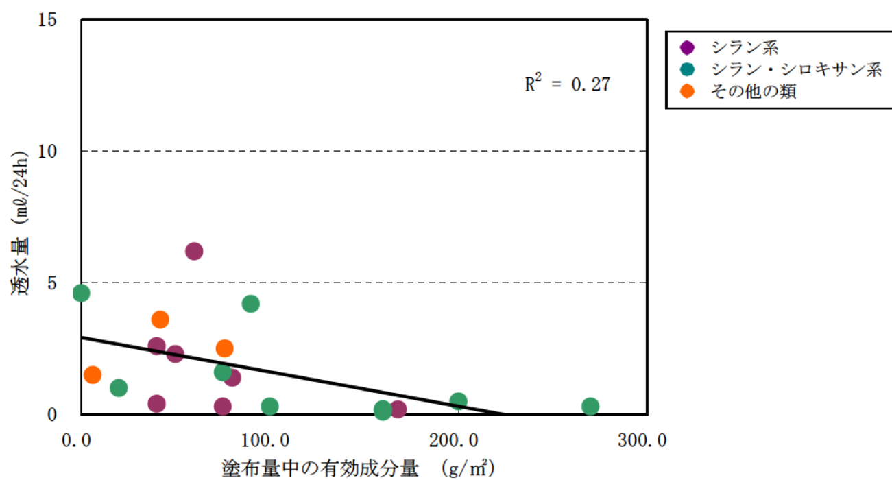
図－Ⅲ．1.86 暴露4年後の透水量と有効成分との関係（n＝20）
