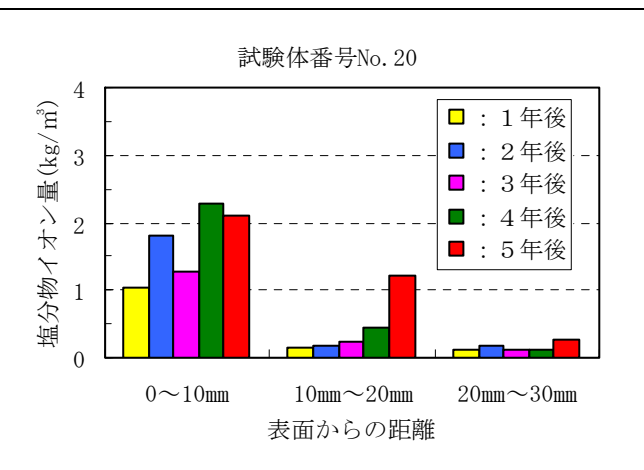
付録図－2.6.4 塩化物イオン量測定結果（その他の類）
