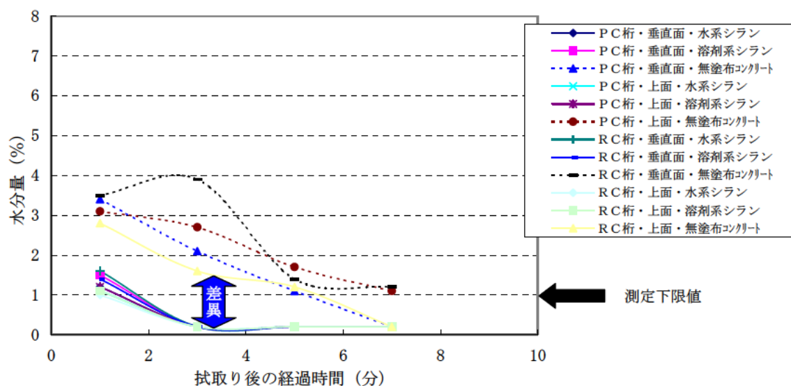
図－Ⅳ. 2. 21 コンクリート桁の部位と保護材種類による水分量の経時変化
