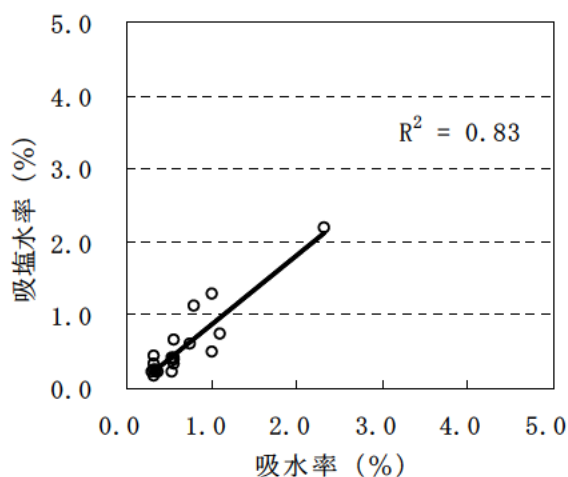
図－V.1.13 吸塩水率と吸水率の関係（ n = 19 ）
