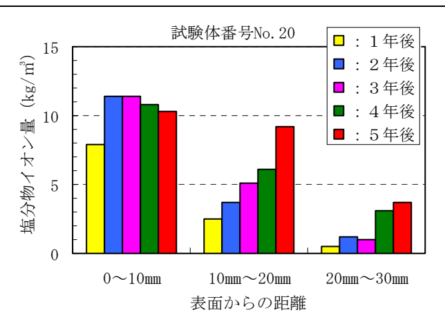
付録図－2.6.8 塩化物イオン量測定結果（その他の類）
