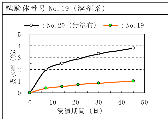
付録図－4. 2. 3 (2) 吸水率測定結果 (その他の類)
