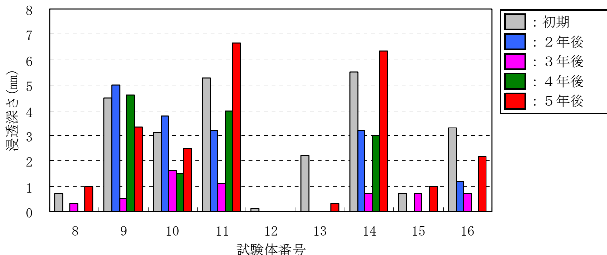
図－Ⅲ．1．62 シラン・シロキサン系の浸透深さ(国道側)
