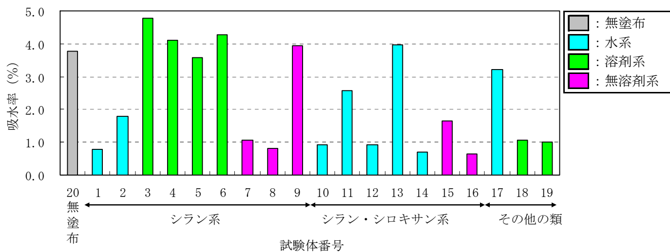
図－Ⅲ.2.54 吸水率
