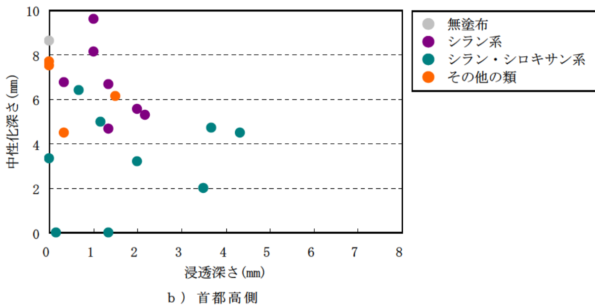
図-III.1.79 浸透深さと中性化深さ（n=21）
