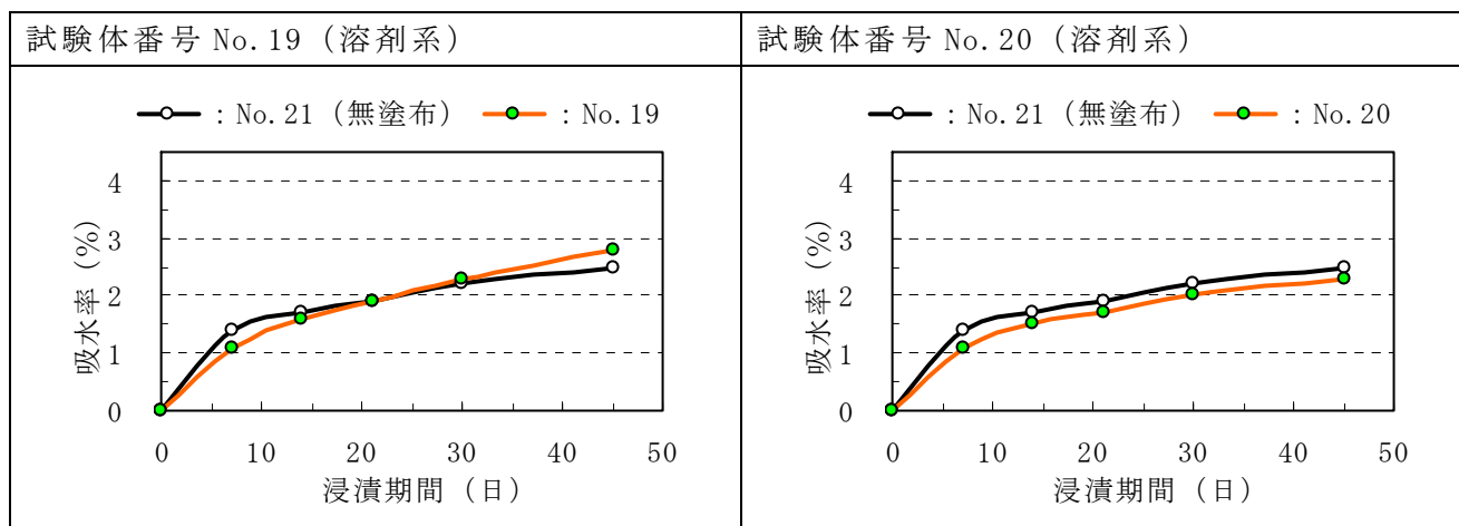
付録図－2.8.3(2) 吸水率測定結果 (その他の類)
