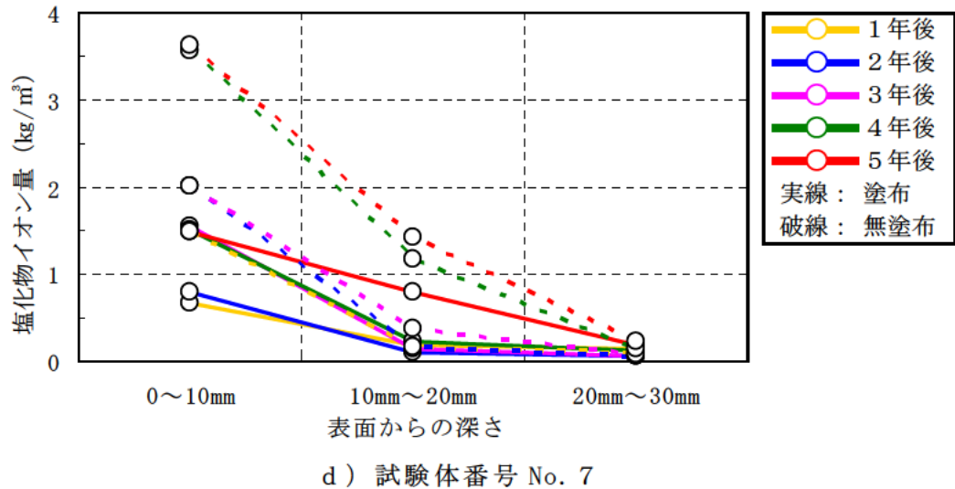
図－Ⅲ. 1. 99(2) シラン系（溶剤系）の塩化物イオン量測定結果
