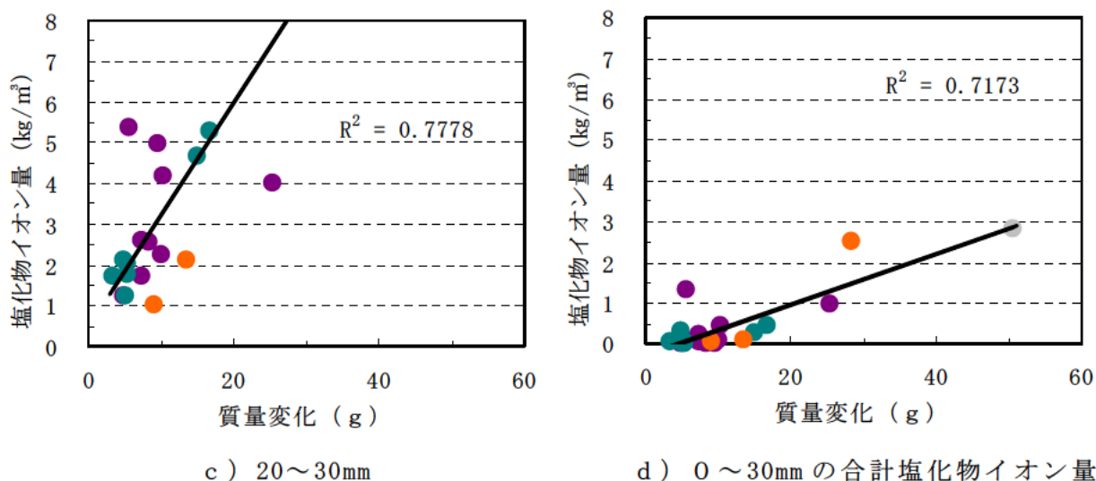
図－V.1.12 質量変化と深さ方向の塩化物イオン量との関係（ n = 20 ）
