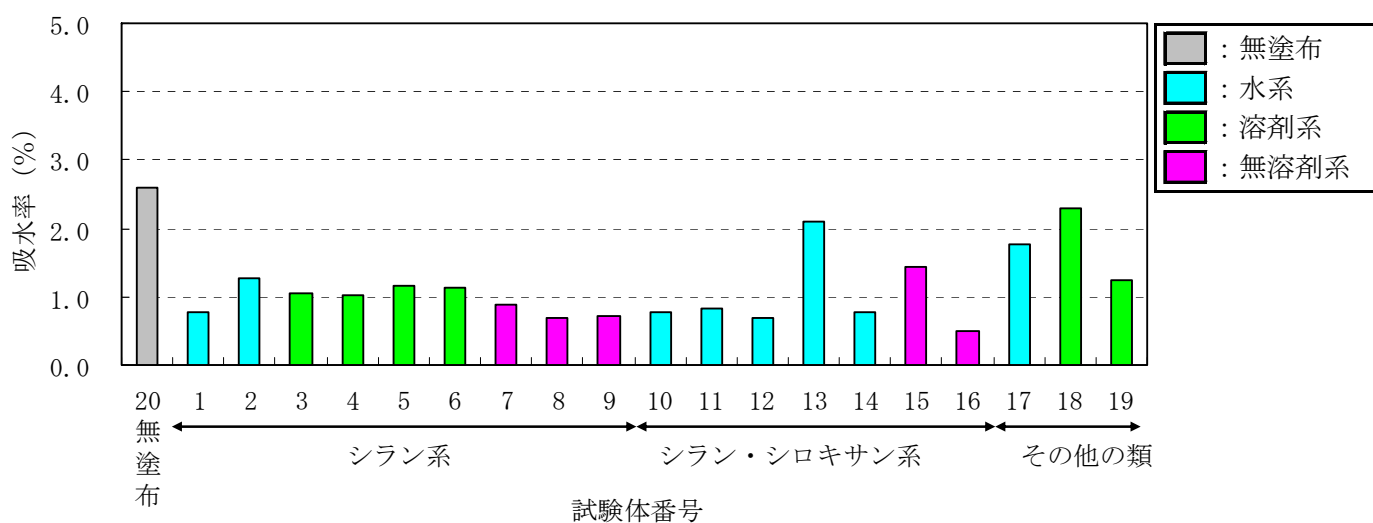
図一Ⅲ.2.24 100 mm × 100 mm × 60 mm (6面塗布) の吸水率
