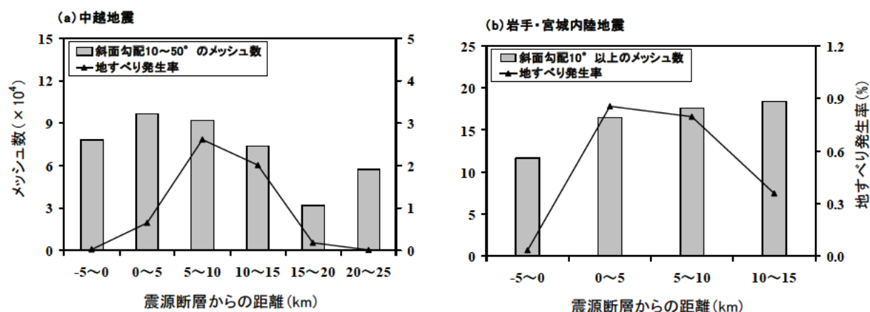
図-16 震源断層から 5 km 範囲毎の斜面勾配と地すべり発生率との関係
