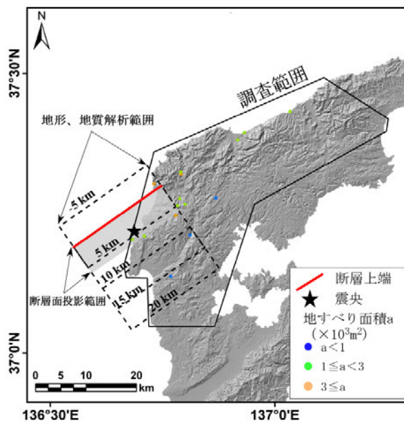
図-4 能登半島地震で発生した地すべりの分布
