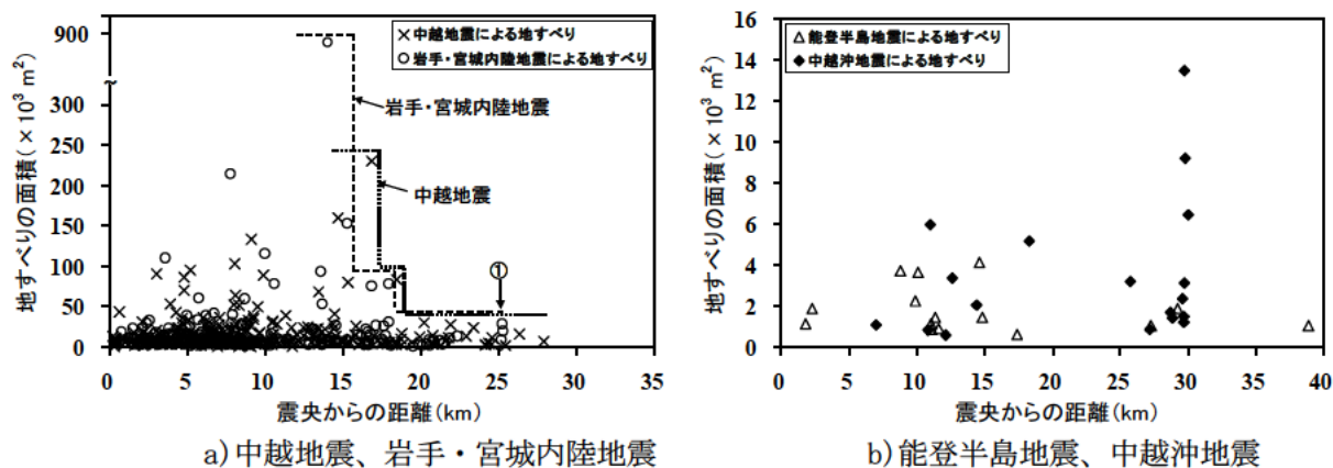
図-12 震央からの距離と地すべりの面積との関係
