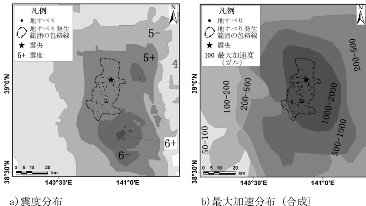
図-11 岩手・宮城内陸地震における震度、最大加速度分布と地すべりが発生した範囲
