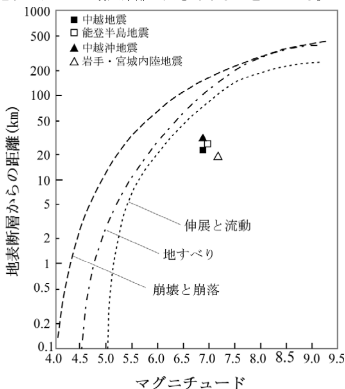
図-20 地震のマグニチュードと地すべりの最大距離 Keefer (1984)の図に加筆。マグニチュードは7.5までがMs, \geq 7.5 はMw。
