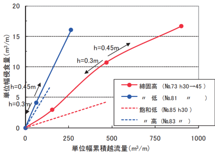
図-1.5 堤体状態及び越水深の影響
