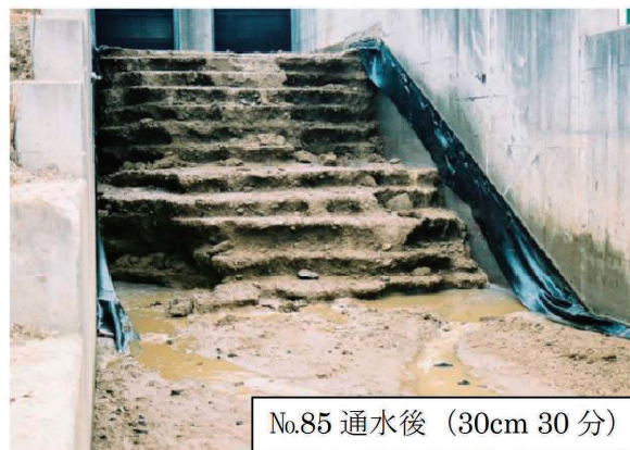
写真-2.7 湛水無し、裸提の実験 (ケース85)
