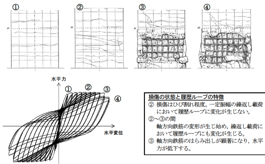
図-5.1 柱基部で曲げ破壊するタイプの鉄筋コンクリート橋脚の水平力-水平変位関係と損傷の進展
