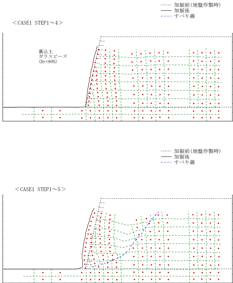
図 4-48 変形状況のスケッチ
