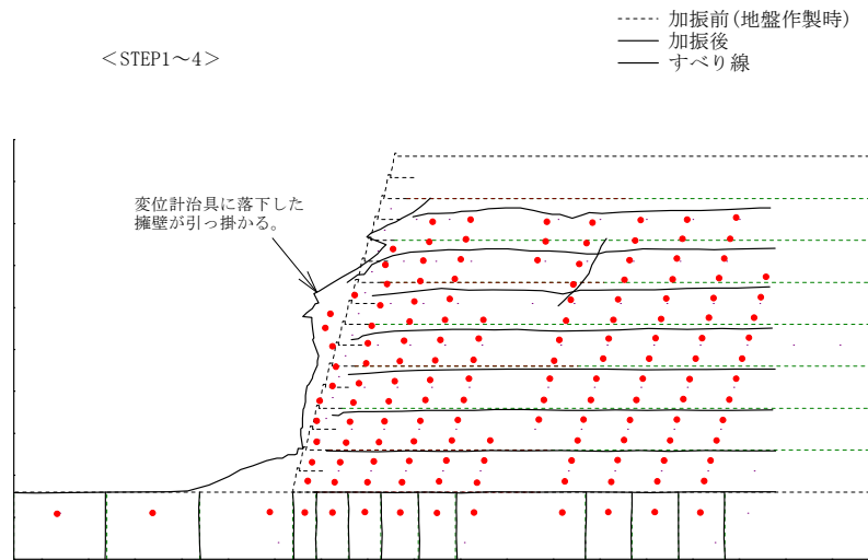
図 4-10 変形状況のスケッチ
