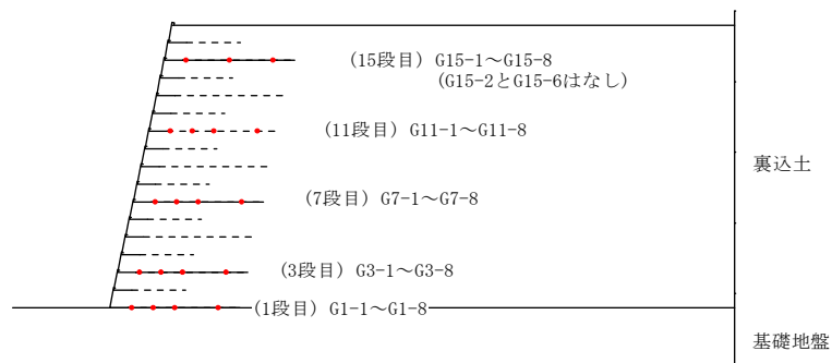
図 3-48 ひずみゲージの貼り付け位置 (GW26)
