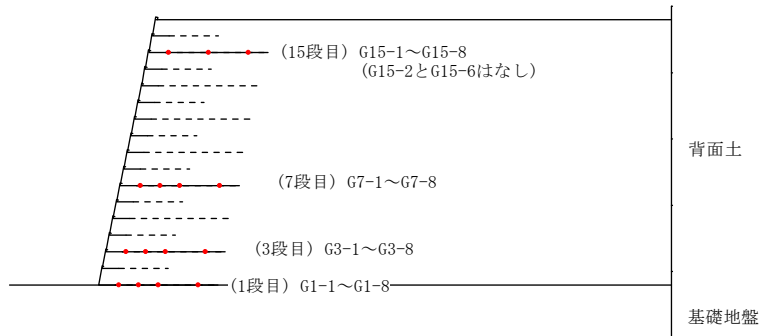
図 3-42 ひずみゲージの貼り付け位置 (GW23)
