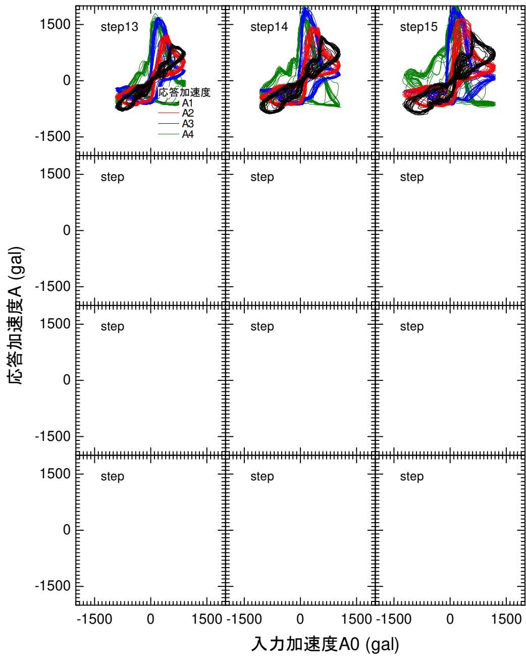
図 4-127 入力加速度と応答加速度の関係 GW33r その2
