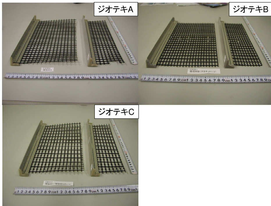
図 2-4 補強材および壁面工模型
