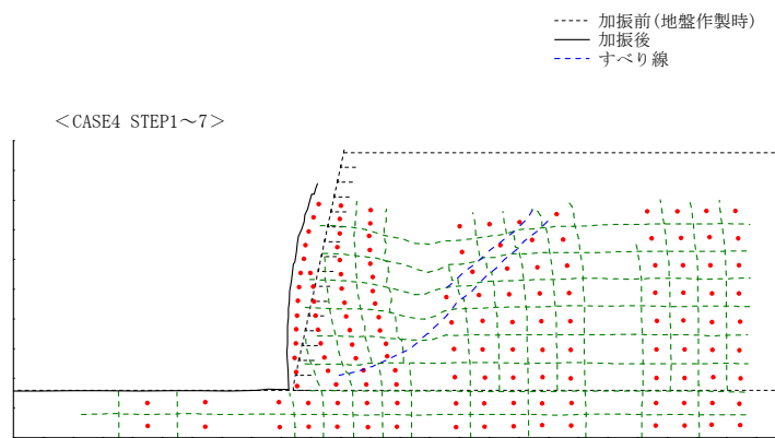
図 4-54 変形状況のスケッチ
