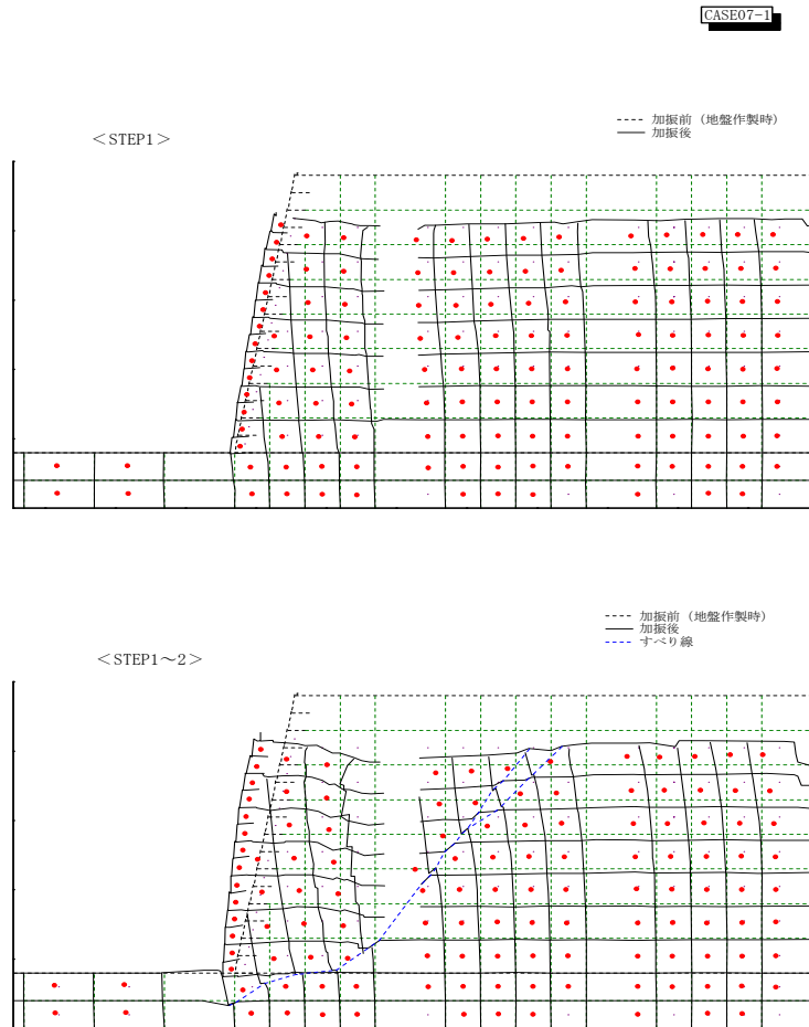
図 4-30 変形状況のスケッチ
