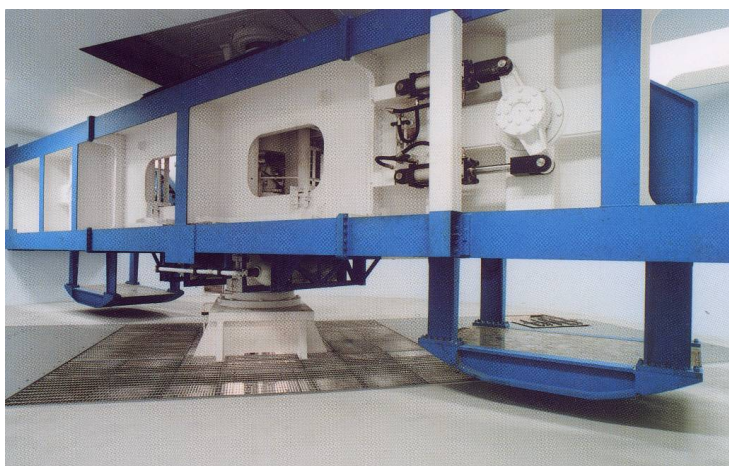
図 2-1 大型遠心力載荷試験装置
