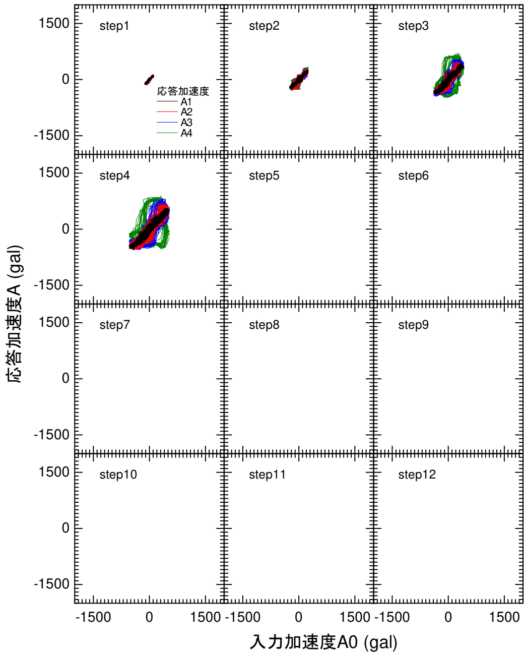
図 4-104 入力加速度と応答加速度の関係 GW05
