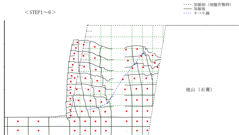
図 4-26 変形状況のスケッチ
