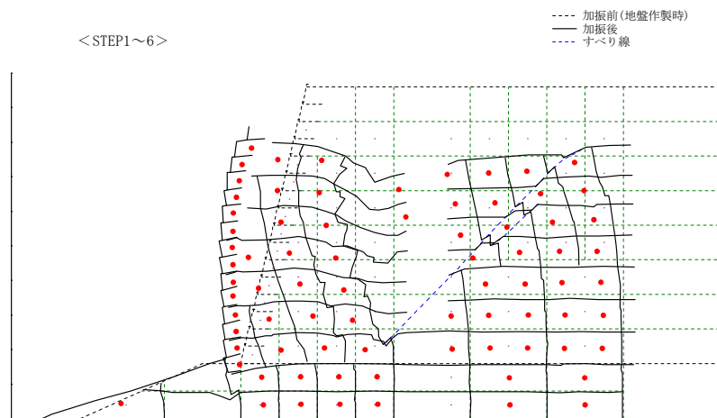
図 4-16 変形状況のスケッチ
