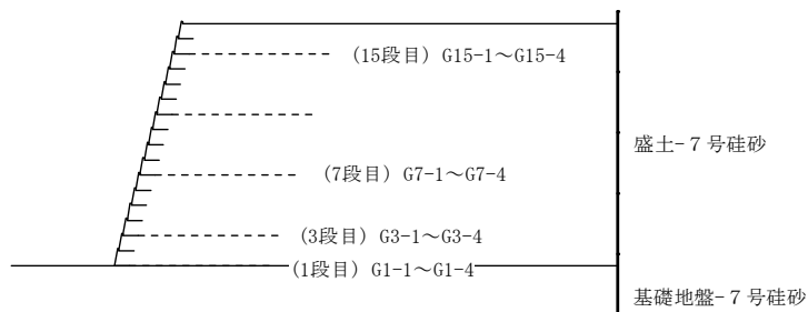
図 3-28 ひずみゲージの貼り付け位置 (GW16)
