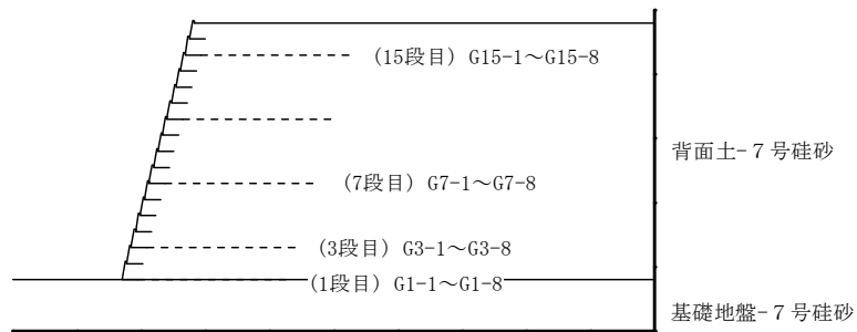
図 3-18 ひずみゲージの貼り付け位置 (GW11)
