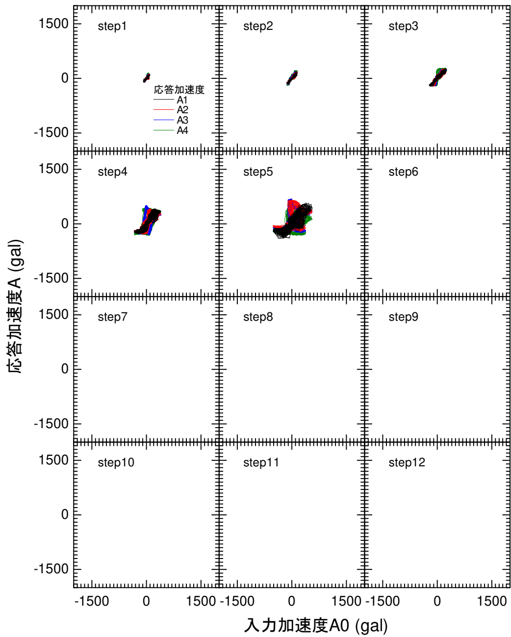
図 4-116 入力加速度と応答加速度の関係 GW24
