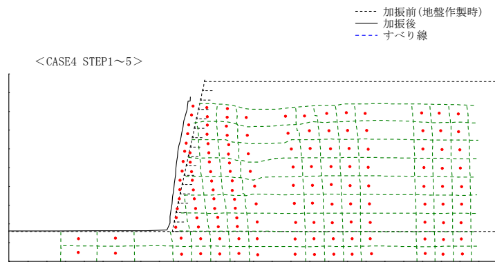
図 4-44 変形状況のスケッチ
