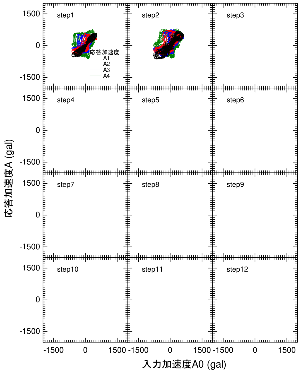
図 4-118 入力加速度と応答加速度の関係 GW26
