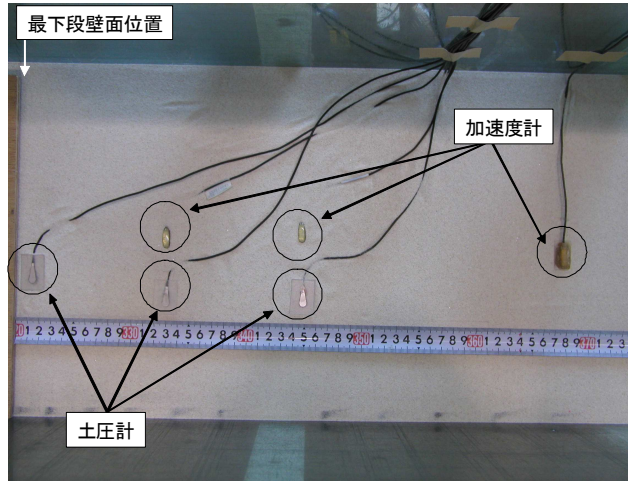
図 2-29 土圧計・加速度計の設置（補強領域底面）
