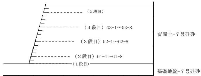
図 3-14 ひずみゲージの貼り付け位置 (GW09)
