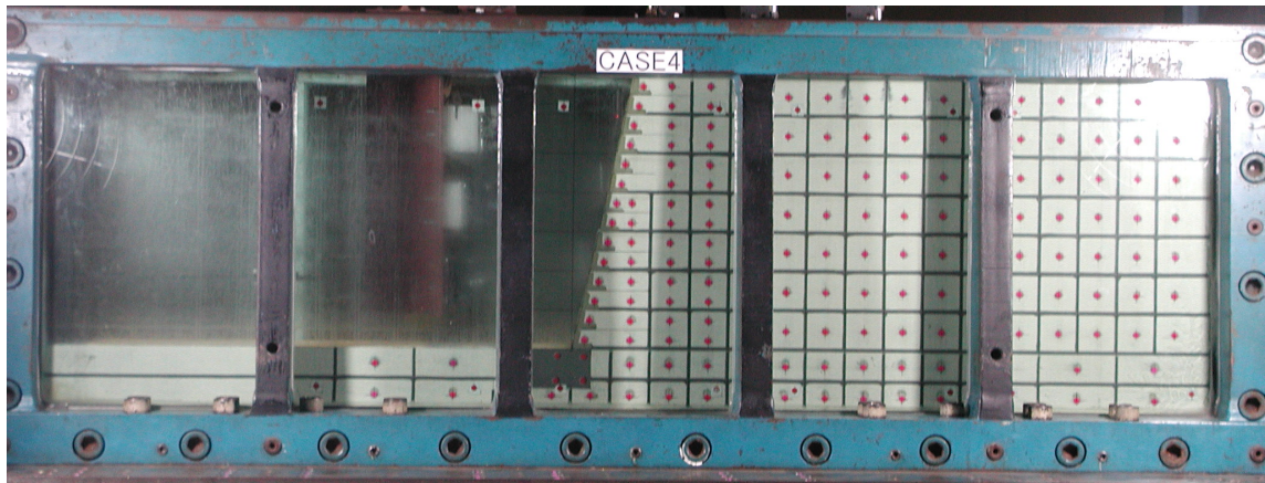
図 2-10 基礎地盤に浅部改良体を設けた GW32
