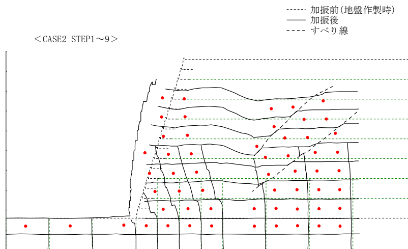
図 4-4 変形状況のスケッチ
