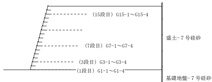
図 3-30 ひずみゲージの貼り付け位置 (GW17)
