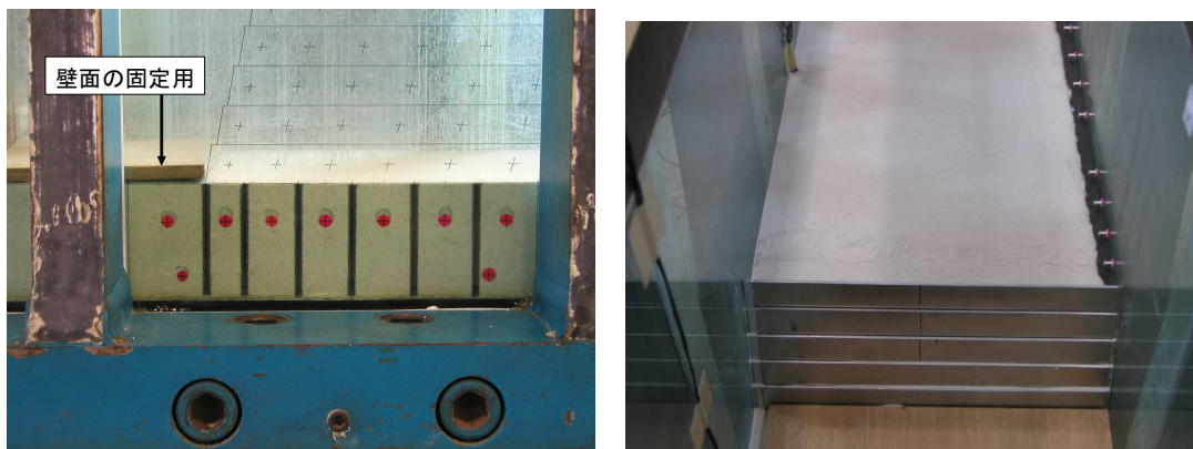
図 2-30 壁面の設置および背後地盤の作製
