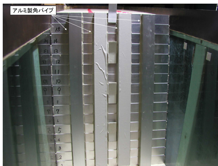
図 2-8 壁面工の一体化
