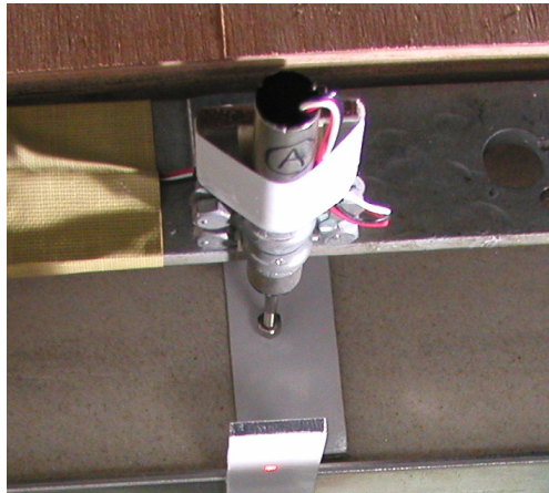
図 2-39 天端沈下計測用ポテンショメータ
