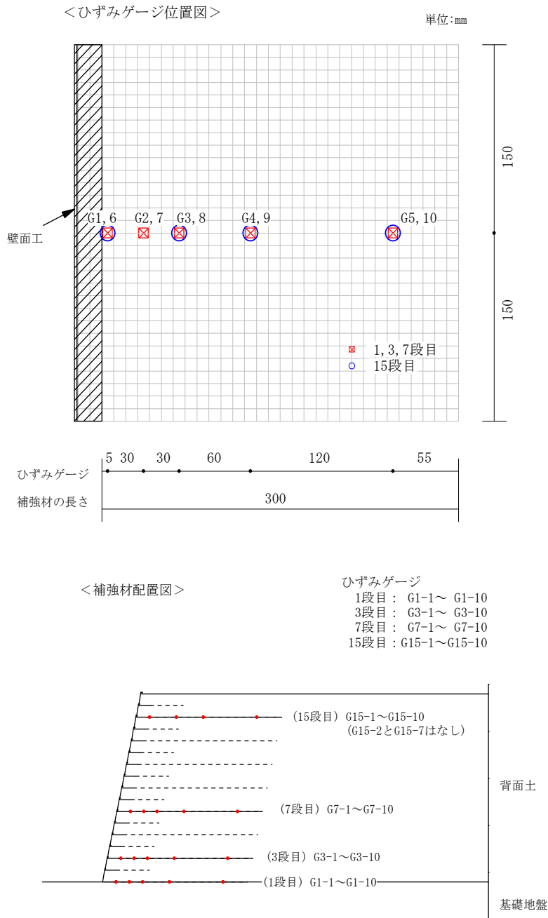
図 3-36 ひずみゲージの貼り付け位置 (GW20)
