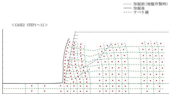
図 4-60 変形状況のスケッチ
