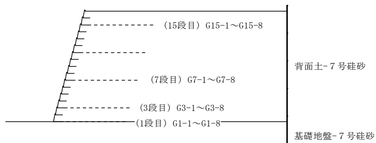
図 3-22 ひずみゲージの貼り付け位置 (GW13)
