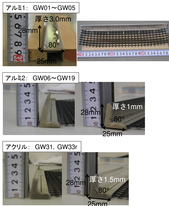
図 2-3 壁面工（模型スケール）
