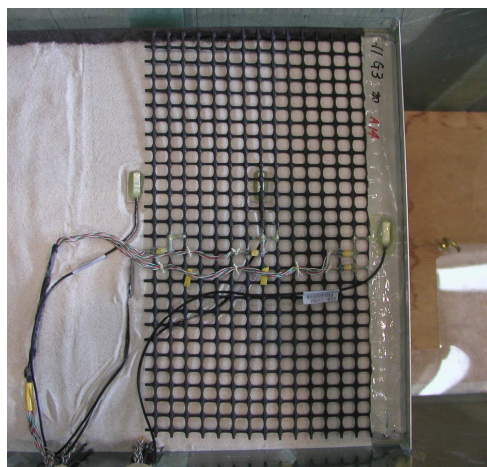
図 2-41 ひずみゲージと補強材
