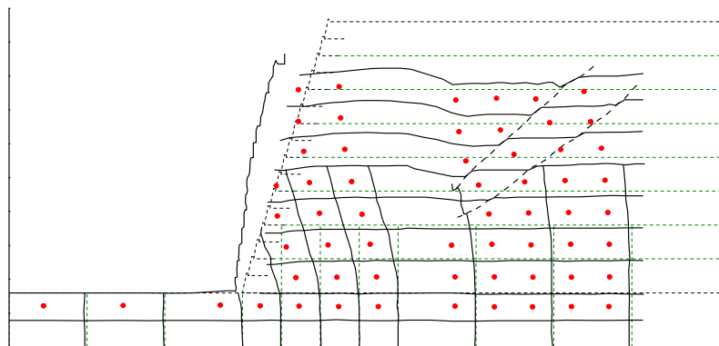
図 4-6 変形状況のスケッチ
