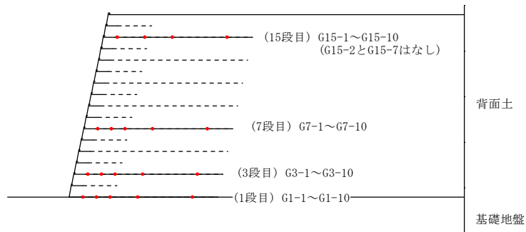
図 3-52 ひずみゲージの貼り付け位置 (GW28)
