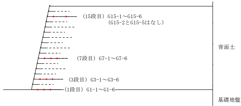
図 3-38 ひずみゲージの貼り付け位置 (GW21)
