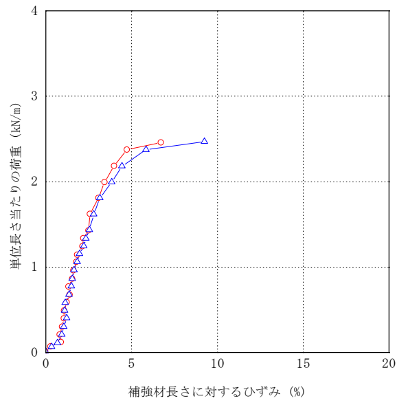
図 2-22 ジオテキ B の引張試験結果 (レーザー変位計に基づくひずみ, 模型スケール)
