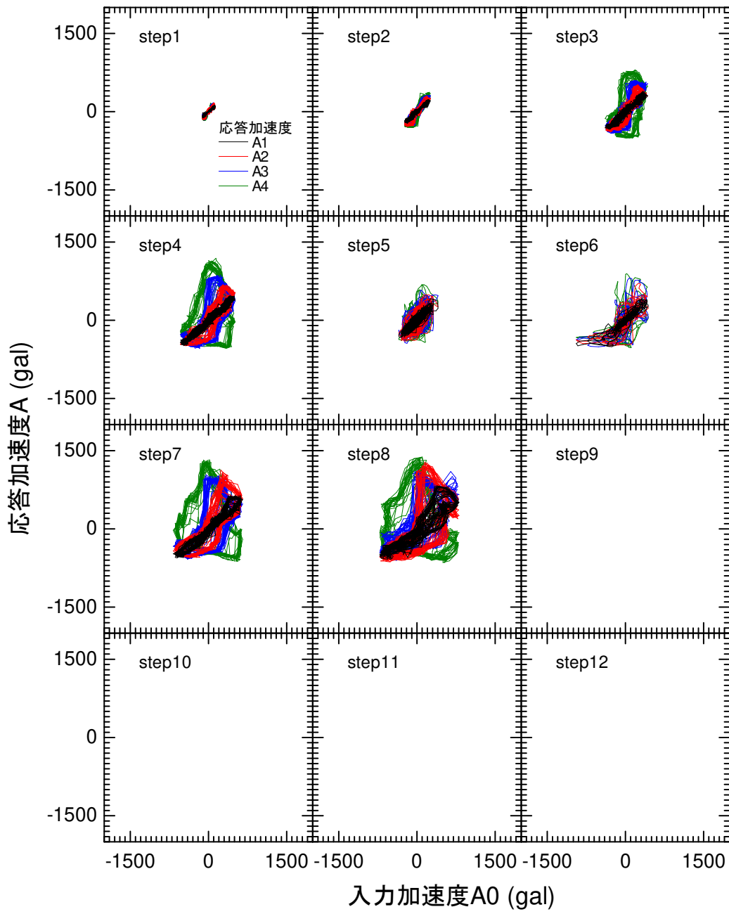
図 4-105 入力加速度と応答加速度の関係 GW06
