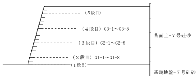
図 3-8 ひずみゲージの貼り付け位置 (GW06)
