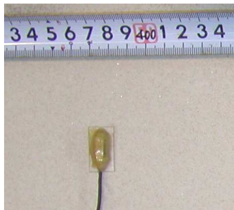
図 2-37 地盤中に設置する場合の加速度計と台座
