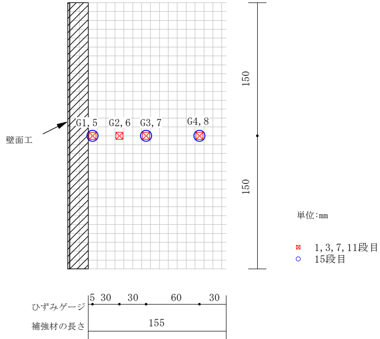
《ひずみゲージ位置図》
