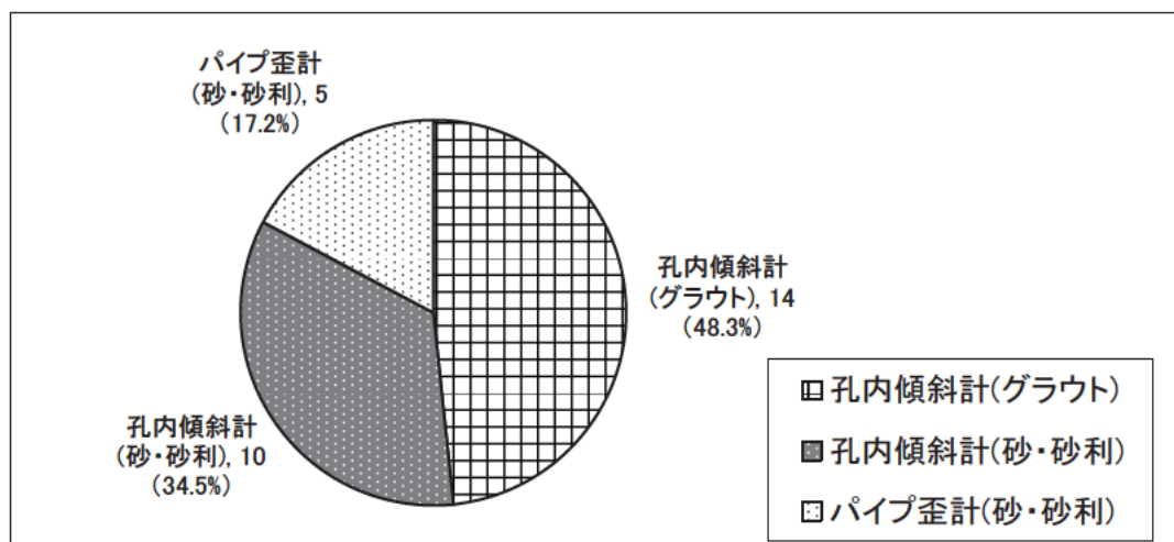
図-3-1-1-1 浮き上がりと充填材の関係
