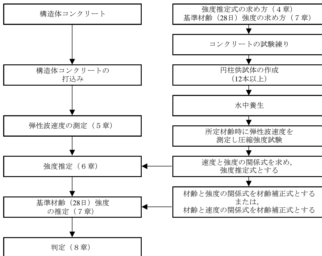
図2 強度推定フロー
