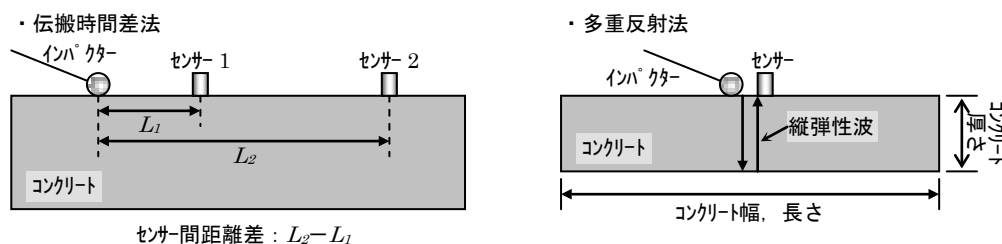
図1 本法での弾性波速度の測定方法
