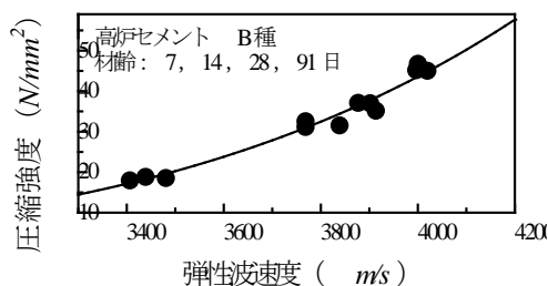
図4 回帰分析例
