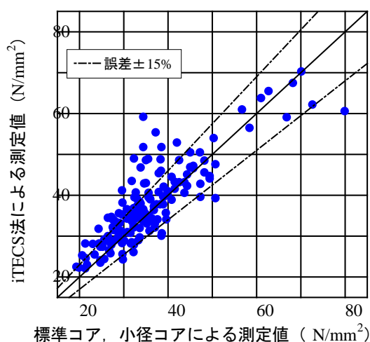
図5 iTECS法による推定強度とコア強度との関係
