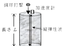
図2 円柱供試体での弾性波速度測定
