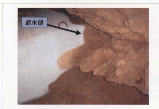
函体と遮水壁が密着している状況
