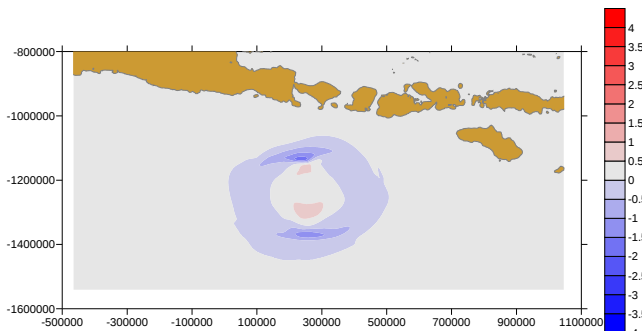
図-2 (2) バリ島南部の津波水位変化（発生 10 分後）
