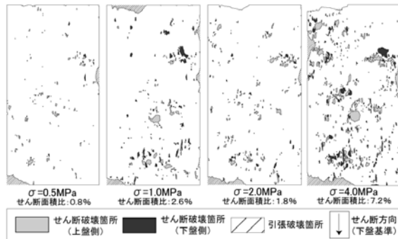
図4 形状A（硬）におけるせん断破壊域の分布
