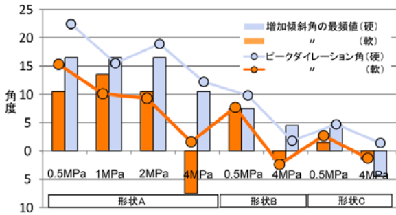
図-9 増加傾斜角の最頻値とピークダイレーション角
