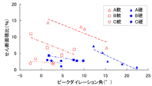
図-10 ピークダイレーション角とせん断面積比の関係 5.2 セン断強度予測式の検証
