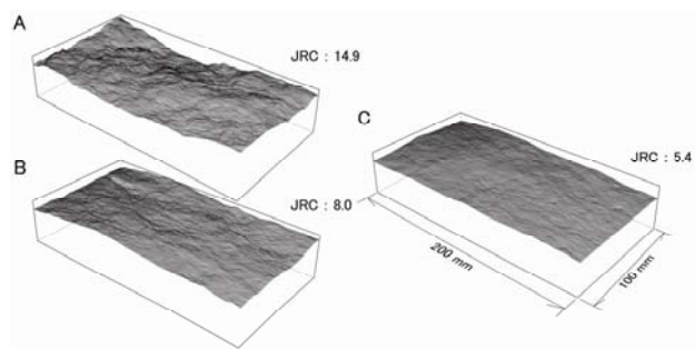
図-1 供試体の形状
