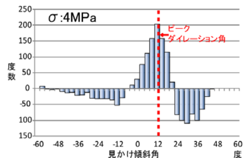
図8 形状A（硬）供試体における傾斜角の増減
