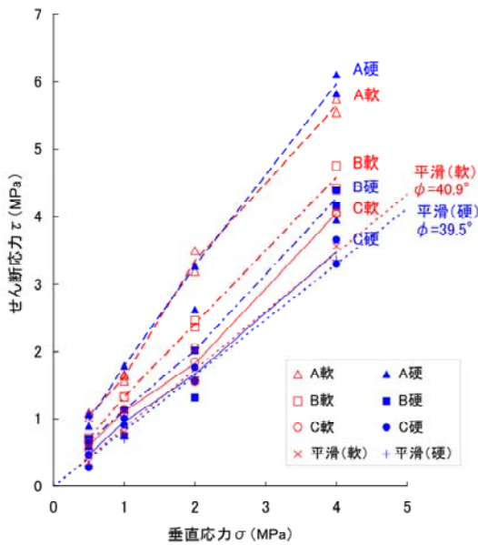
図-3 せん断試験結果
