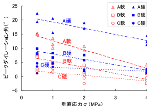
図6 各試験のピークダイレーション角
