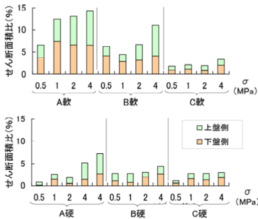
図5 ピークせん断応力直後の破壊面積
