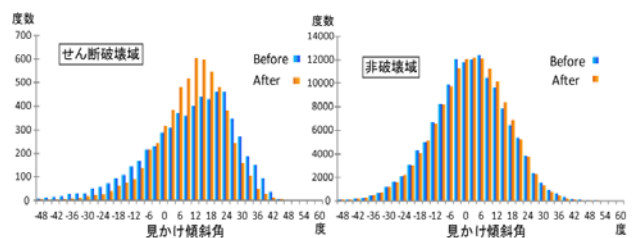
図7 せん断による供試体表面の傾斜変化
