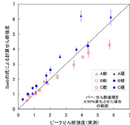
図-11 実測値と計算値の関係
