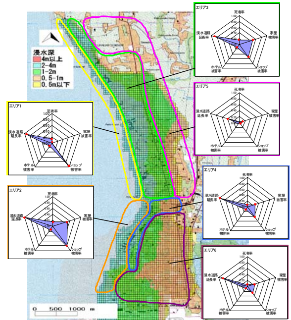
図-7 クタ地区における津波災害リスクマップ
