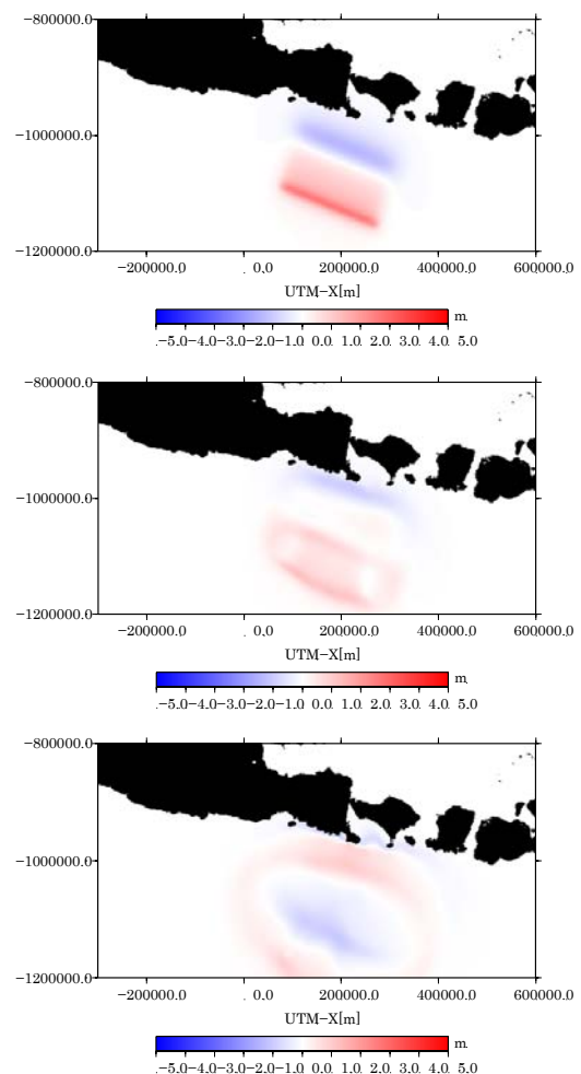
図-2 津波の水位変化
