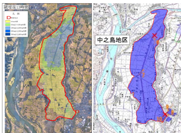
図-6 洪水氾濫域再現シミュレーション結果図（左：シミュレーション結果、右：洪水氾濫実績 6) ）
