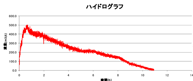
図-5 破堤流量のハイドログラフ
