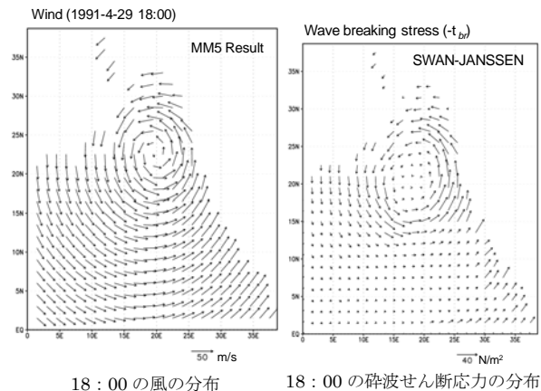
図-8 風速および碎波せん断応力分布
