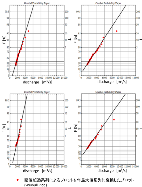
図 9 近未来気候実験における年最大値系列に変換された閾値超過系列資料
