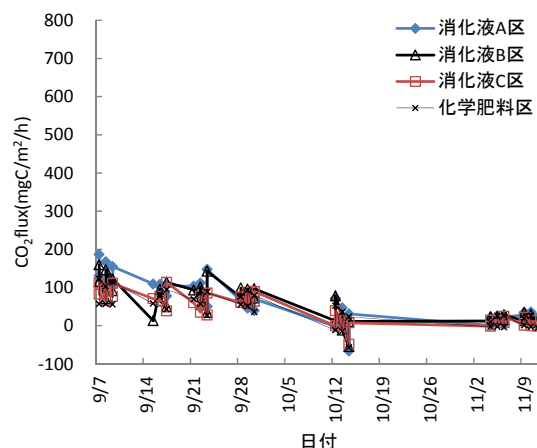
図 29 CO 2 フラックス（消化液区および化学肥料区）（二番草刈取後以降）
