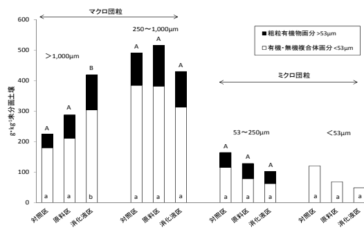
図 16 表層1層目の団粒のサイズ別重量分布
