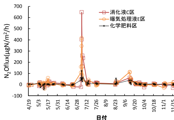
図 38 N 2 O フラックス
