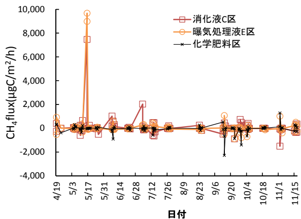
図 35 CH 4 フラックス
