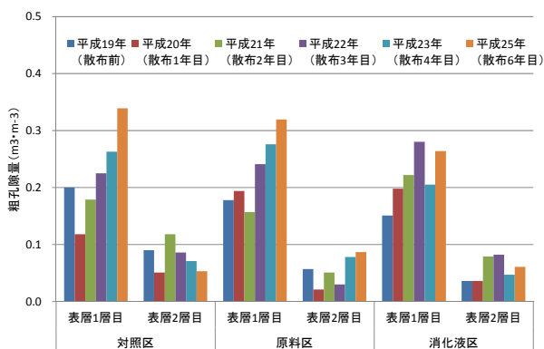
図22 各試験区における粗孔隙量の推移
