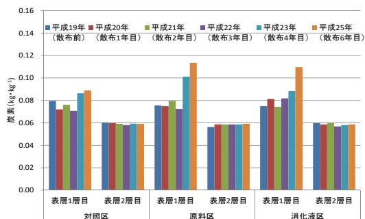
図 14 各試験区における炭素の推移
