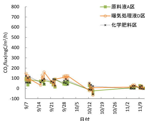
図 30 CO 2 フラックス（消化液区以外）（二番草刈取後以降）
