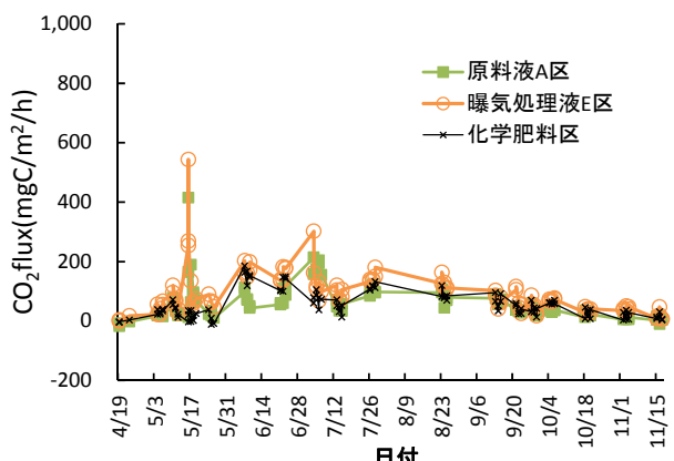
図 32 CO 2 フラックス (消化液区以外)
