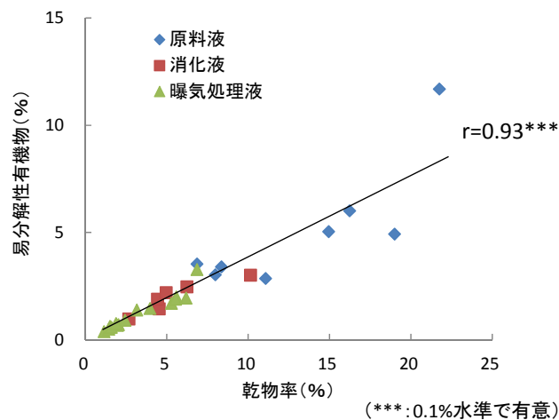
図 10 乾物率と易分解性有機物割合との関係(H25)
