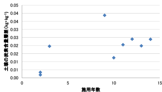
図 39 施用年数と土壌の炭素含量層差の関係
