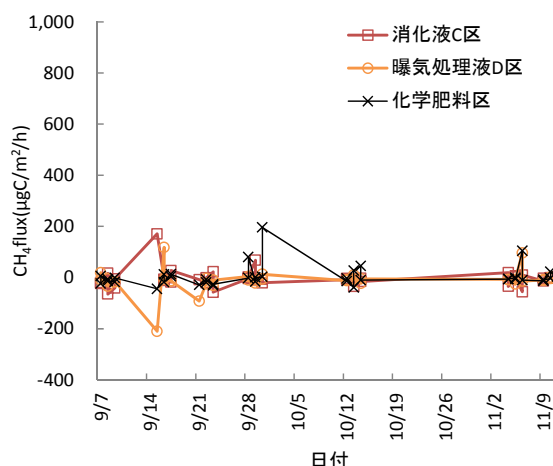
図 34 CH 4 フラックス (二番草刈取後以降)
