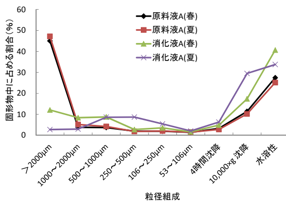
図 6 プラント A 試料中の粒径組成(H25)
