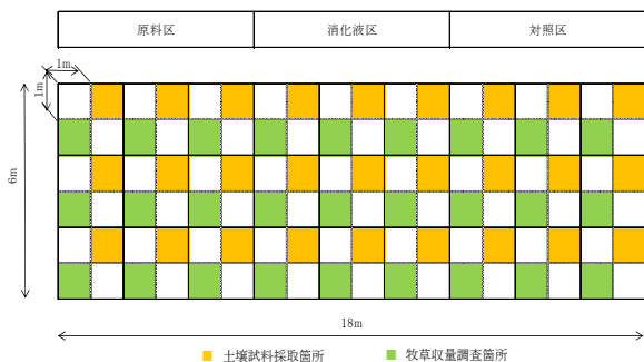
図1 試験区 A 配置図
