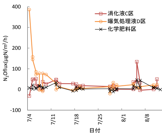
図 36 N 2 O フラックス (施肥直後～二番草刈取前)
