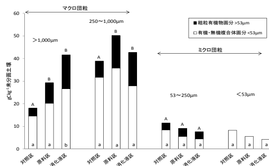
図 17 表層1層目の団粒のサイズ別炭素分布
