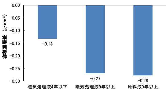
図41 施用年数別の容積重層差
