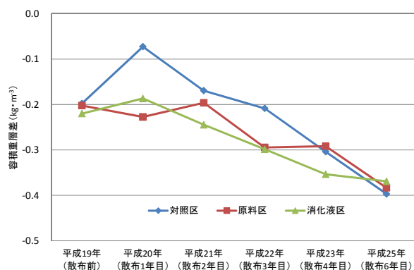
図 21 各試験区における容積重層差の推移
