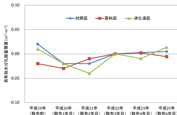
図25 各試験区における易有効水分孔隙量層差の推移
