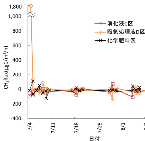
図 33 CH 4 フラックス (施肥直後～二番草刈取前)
