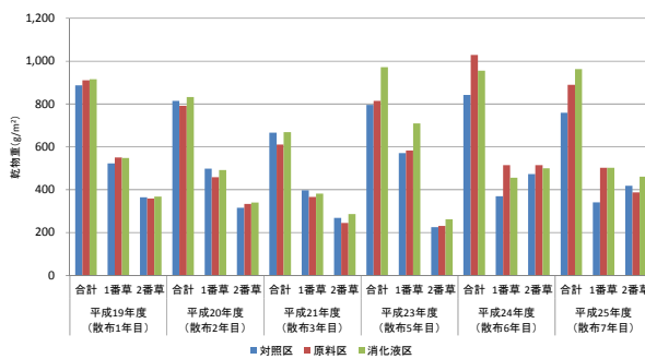
図26 各試験区の調査年度ごとの乾物重
