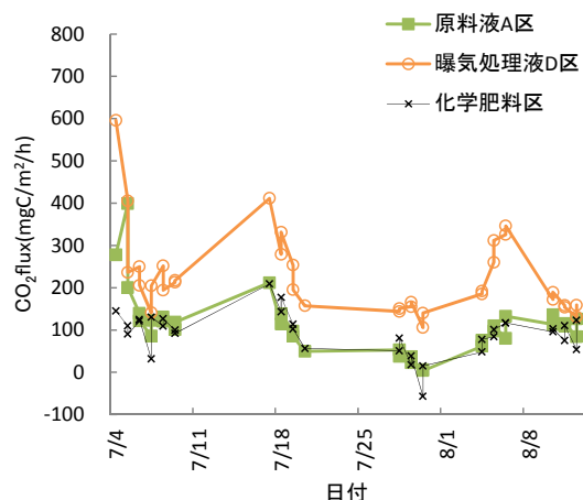
図 28 CO 2 フラックス（消化液区以外）（施肥直後～二番草刈取前）
