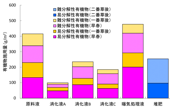
図 12 有機物施用量 (H24)
