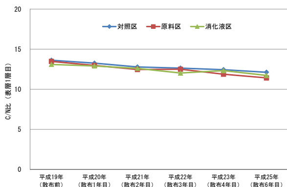
図 18 各試験区における表層 1 層目の C/N 比の推移
