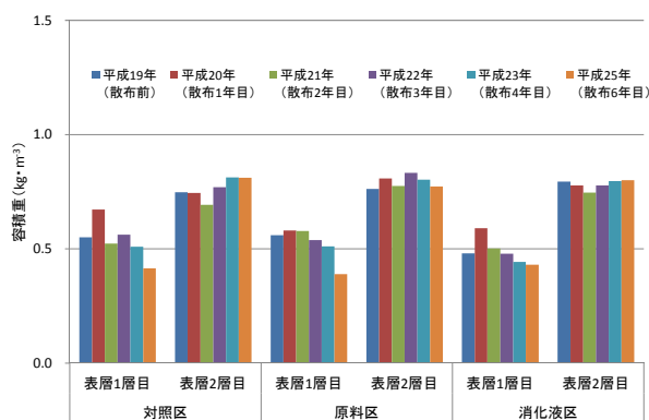
図 20 各試験区における容積重の推移
