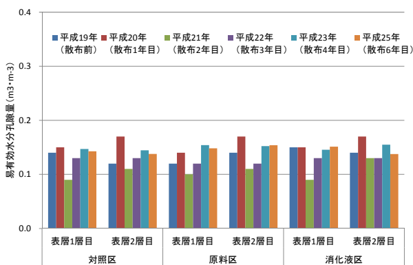
図23 各試験区における易有効水分孔隙量の推移
