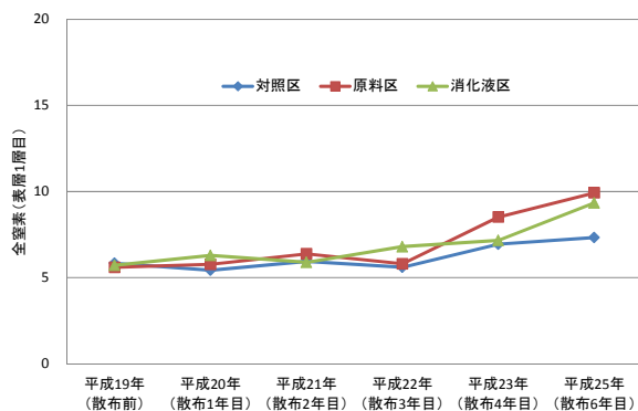
図 19 各試験区における表層 1 層目の全窒素
