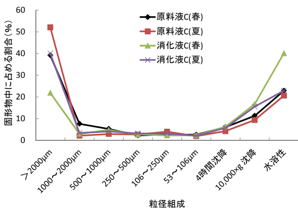
図8 プラント C 試料中の粒径組成(H25)
