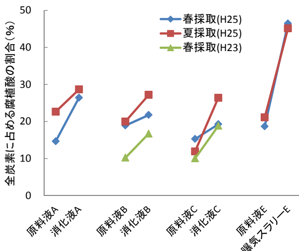
図 4 全炭素に占める腐植酸の割合
