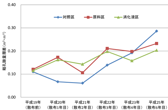
図24 各試験区における粗孔隙量層差の推移
