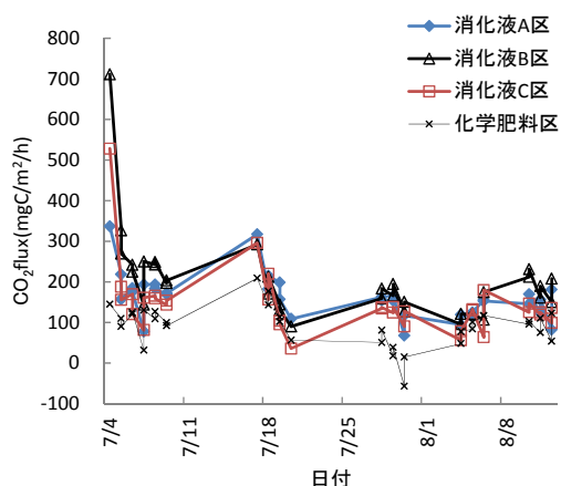
図 27 CO 2 フラックス（消化液区および化学肥料区）（施肥直後～二番草刈取前）
