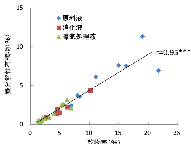
図 11 乾物率と難分解性有機物割合との関係(H25)
