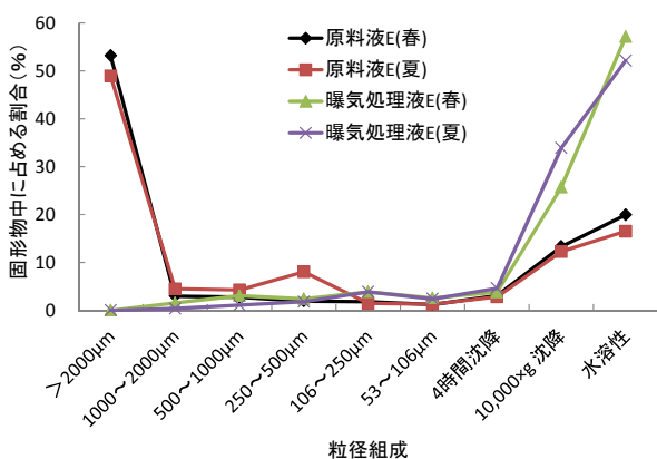
図9 肥培かんがい施設 E 試料中の粒径組成(H25)
