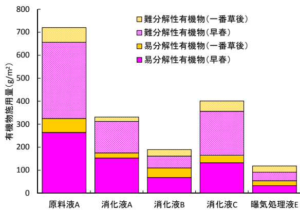
図 13 有機物施用量 (H25)
