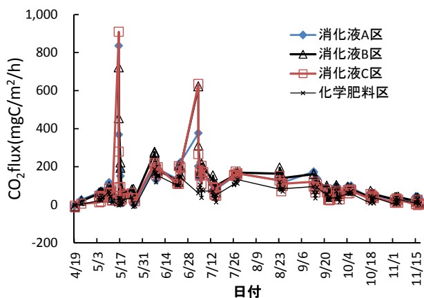
図 31 CO 2 フラックス (消化液区および化学肥料区)
