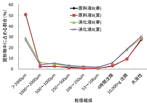
図 7 プラント B 試料中の粒径組成(H25)
