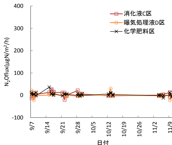
図 37 N 2 O フラックス (二番草刈取後以降)
