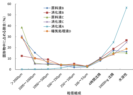
図 5 試料中に含まれる固形物の粒径組成(H23)
