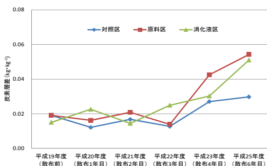
図 15 各試験区における炭素層差の推移
