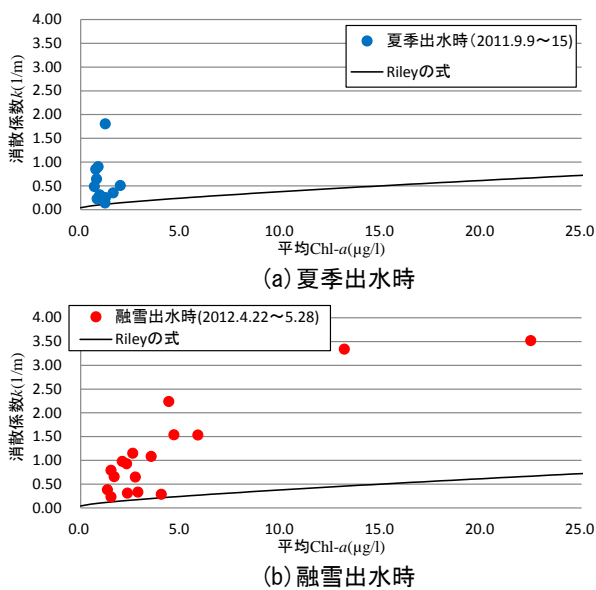
図-17 消散係数とクロロフィル a の関係
