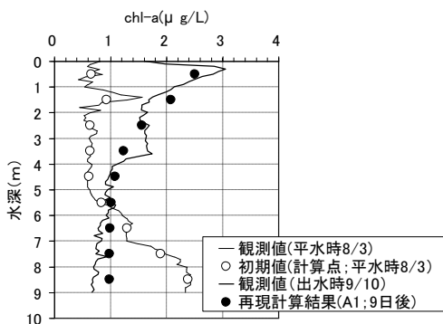
図-15 現況再現計算結果 St.2-3
