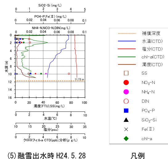
図-7 水温・塩分・Chl-a・栄養塩の鉛直分布 (St. 2-3)
