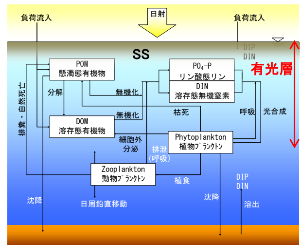
図-14 生態系モデルの概念図 7)
