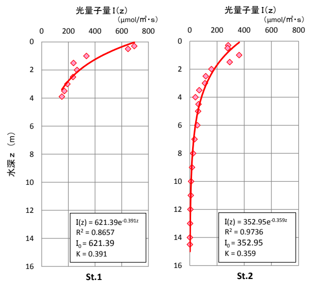
図-22 光量子量と消散係数の実測値
