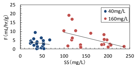
図-27 浮遊物質 SS と濾水速度 (6 時間計測)
