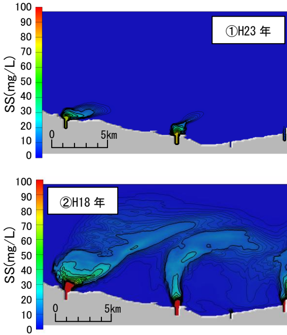
図-12 浮遊物質 SS の拡散状況
