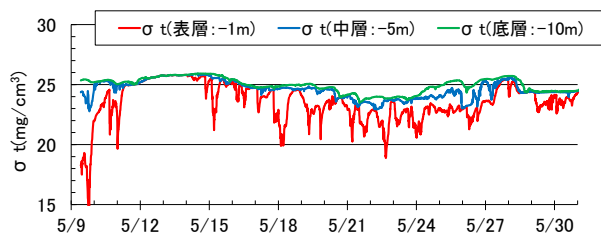
図-8 \sigma_t の時系列変化（融雪出水時、St. 2-3）
