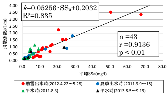
図-18 消散係数と SSa の関係
