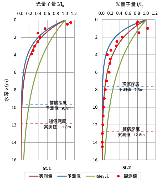
図-23 消散係数 k の比較
