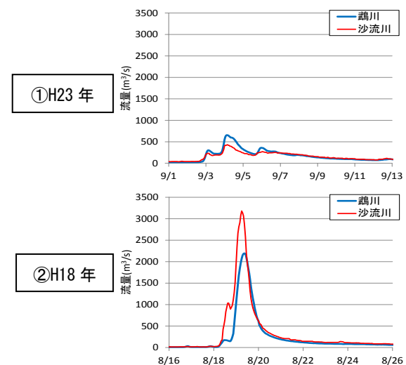
図-11 鵜川、沙流川の河川流量
