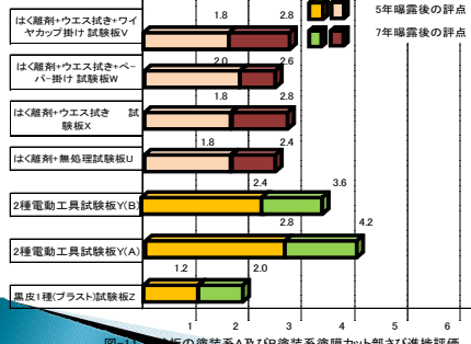
図-11 素地調整工法の塗装系A及びB塗装系塗膜カット部さび進捗評価
