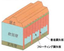
矢板工法 (PFS工法)
