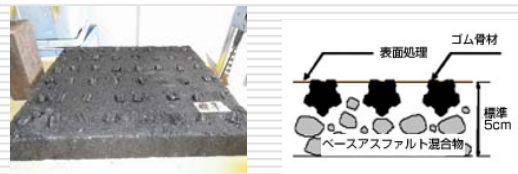
物理系凍結抑制舗装の一例（ゴム圧入型）
