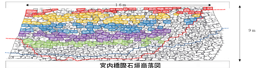
宮内橋際石垣崩落図 (赤破線: 熊本地震崩落 青破線: 平成15年度修復) *1面目のみ表示 透視値
