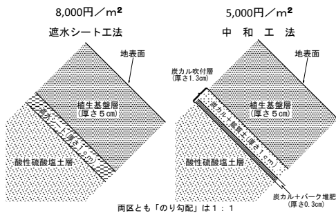
第1図 各試験施工区の施工断面
