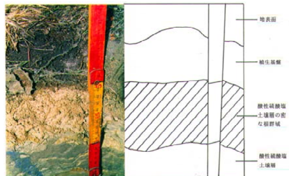
写真-4 中和工法区の酸性硫酸塩土層層における植生根の侵入状況 (施工3年後:1995年7月4日撮影)
