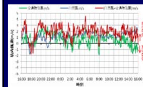
【風速成分(解析値)】
