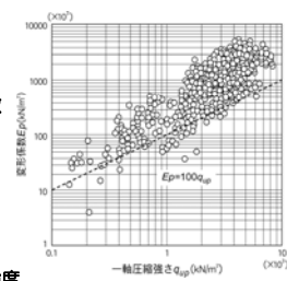
地盤改良強度と 変形係数の関係
