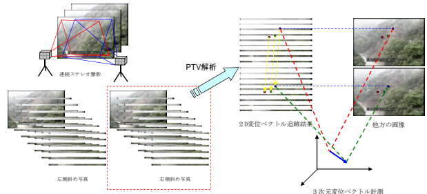
片方の時系列画像を用いたPTV・PIVベクトルから、3次元変位ベクトル算出
