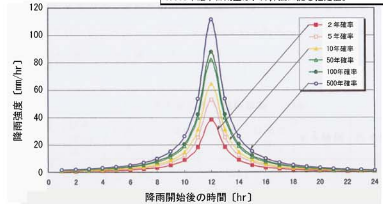
太宰府市における確率N年降雨の連続降雨曲線(ハイエトグラフ)
