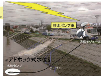
※アドホック式水位計 移動式アドホック型簡易水位計を利用した水位観測イメージ
