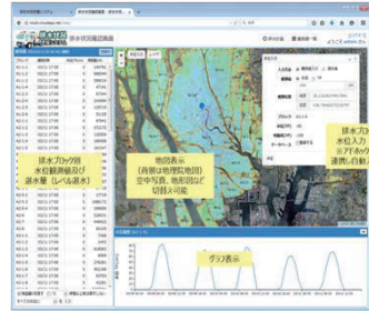
排水システム アウトプットのイメージ
