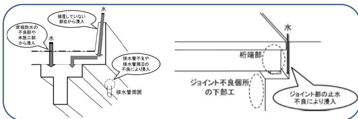
水分によって変状が生じやすい箇所例
