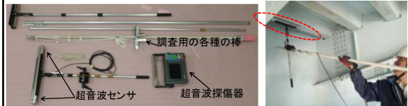
開発した超音波装置
