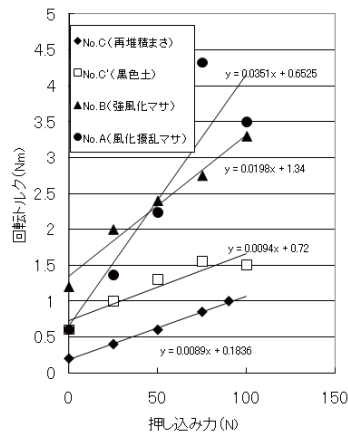
ベーンコーンせん断試験結果の例
