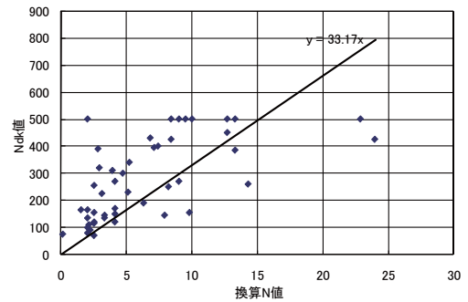
スウェーデン式サウンデイングによる換算N値と土検棒貫入強度の関係
