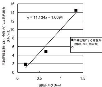
室内三軸圧縮試験による粘着力Cや内部摩擦角φの関係(相関式)の例
