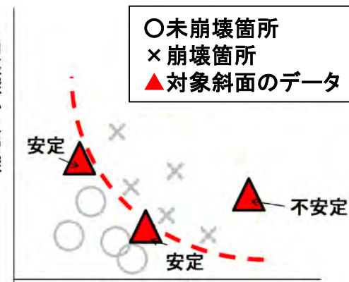
斜面勾配(°) 崩壊危険性評価図
