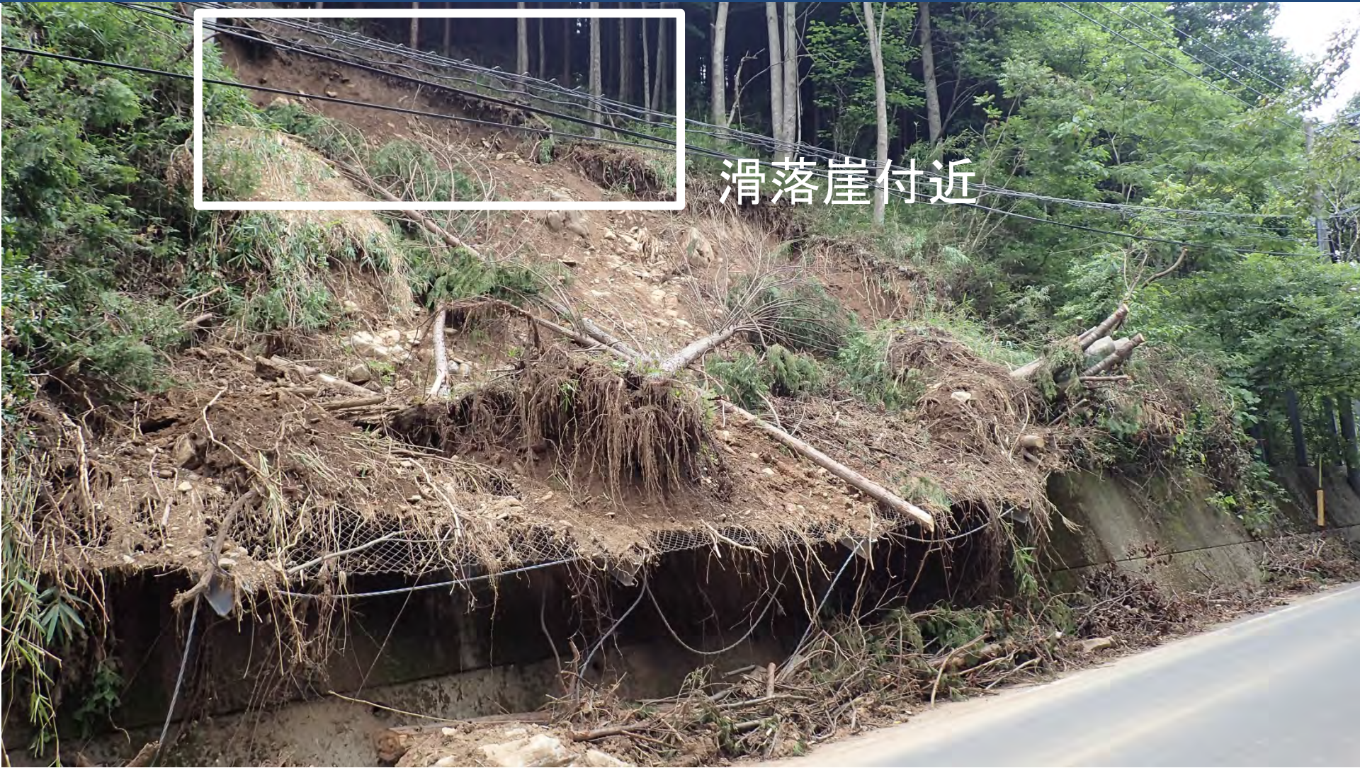
道路斜面で発生した表層崩壊の頭部（滑落崖）の状況
