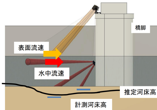
縦断面図
