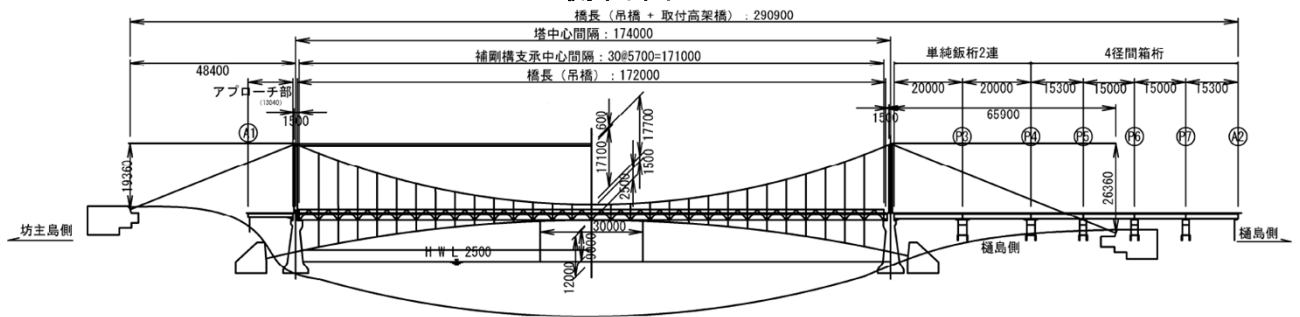
側面図
