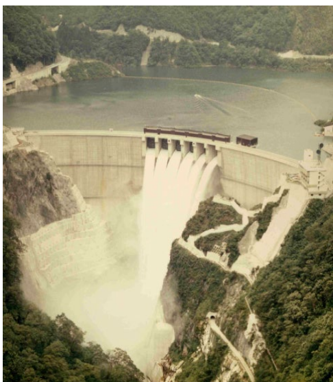
川治ダム
