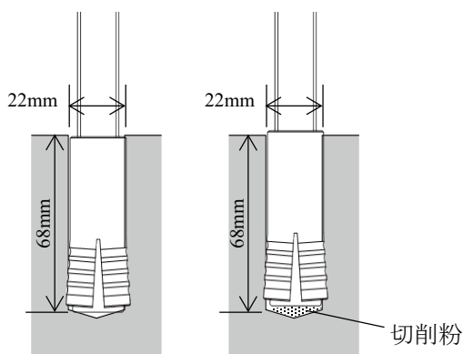
(a) 孔内清掃あり（適切） (b) 孔内清掃なし
