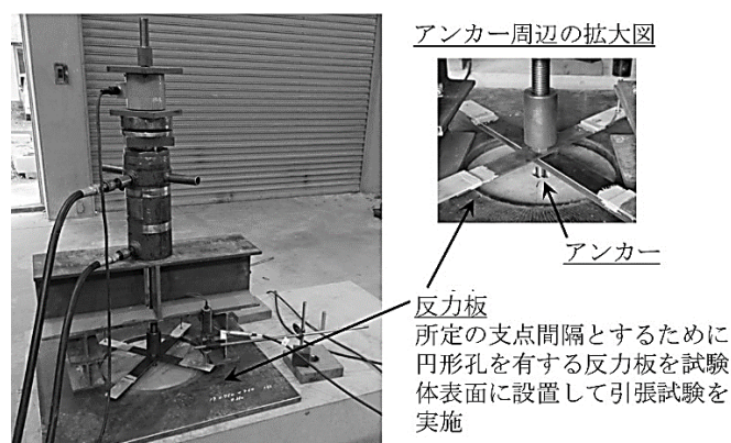
写真 4-1 引張試験の状況 (荷重の測定)
