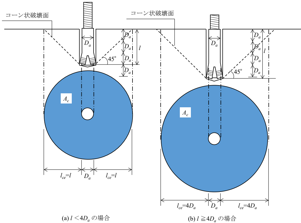
図 2-6 有効水平投影面積 A_c の求め方
