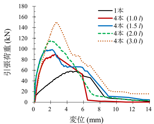
図 4-12 荷重-変位曲線の例
