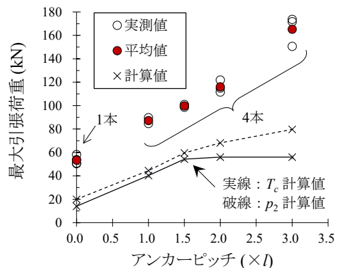
図 4-7 アンカーピッチと最大引張荷重
