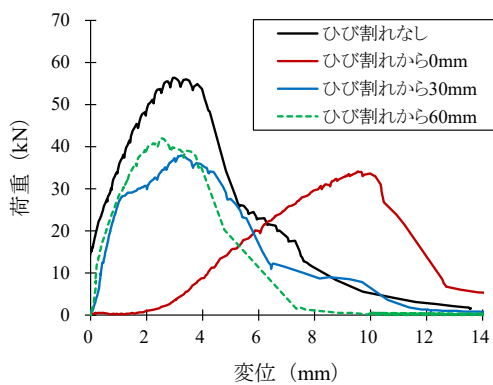
図 6-3 荷重－変位曲線
