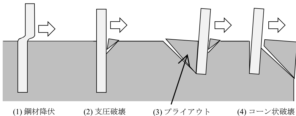
図 2-3 アンカーのせん断力に対する破壊モード
