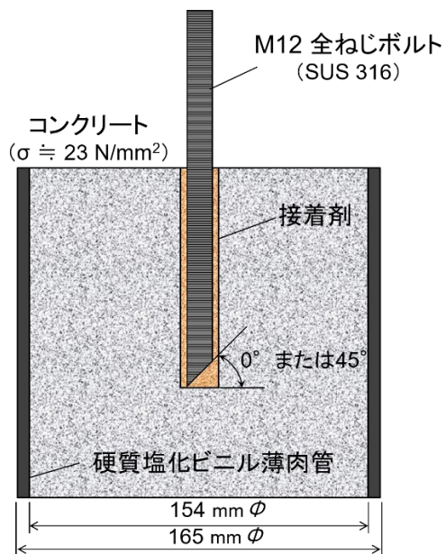
参考 図 1.2.3.3 試験体の概略図
