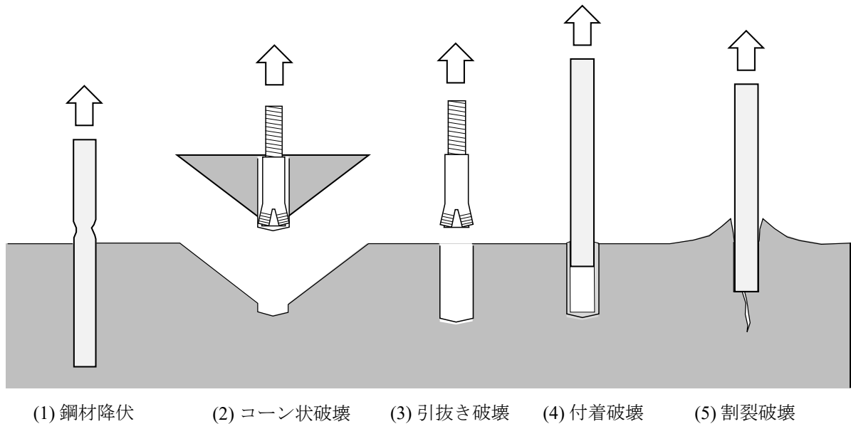
図 2-2 アンカーの引張力に対する破壊モード
