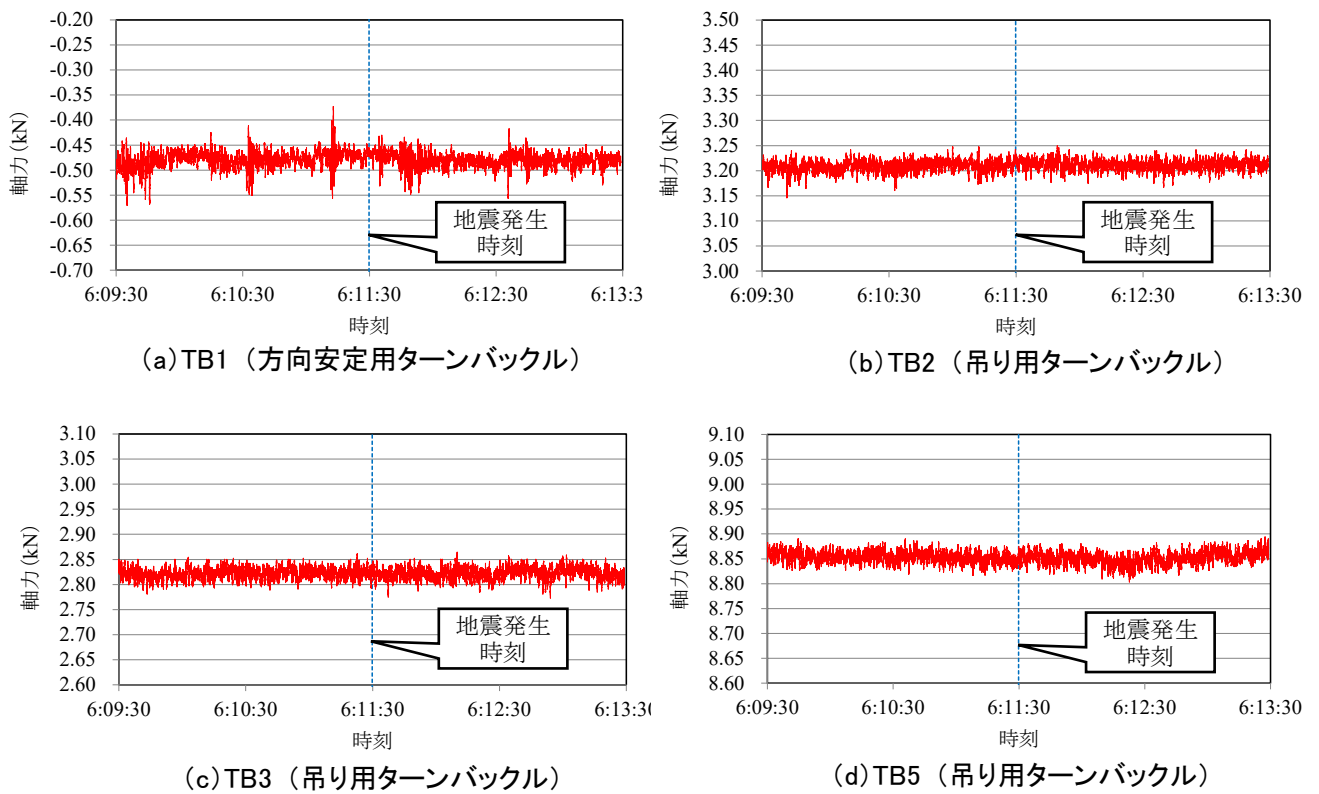
図 3-11 No. 7 地震発生時の各ターンバックルの軸力変動
