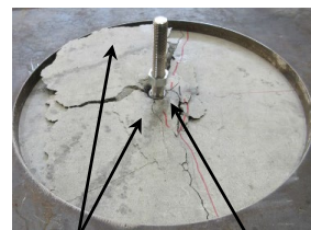
コーン状破壊 導入したひび割れ
