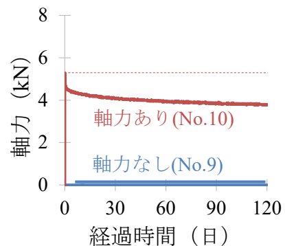
図 4-32 アンカーの軸力の経時変化
