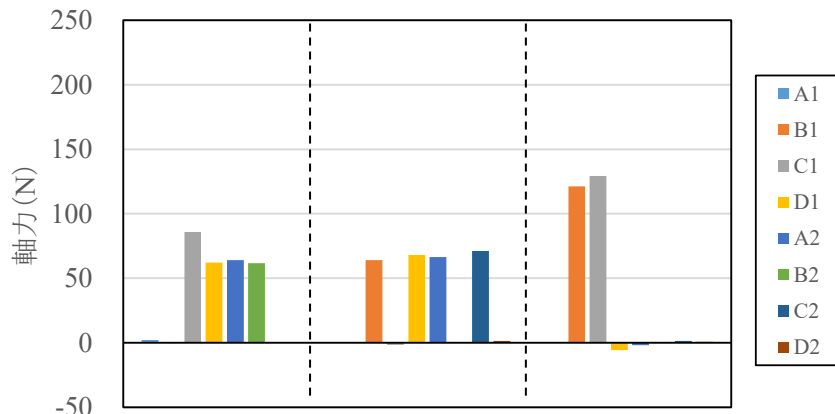
2 本目に切断したターンバックル (b) シリーズ 4 (たるみ: 有り)
