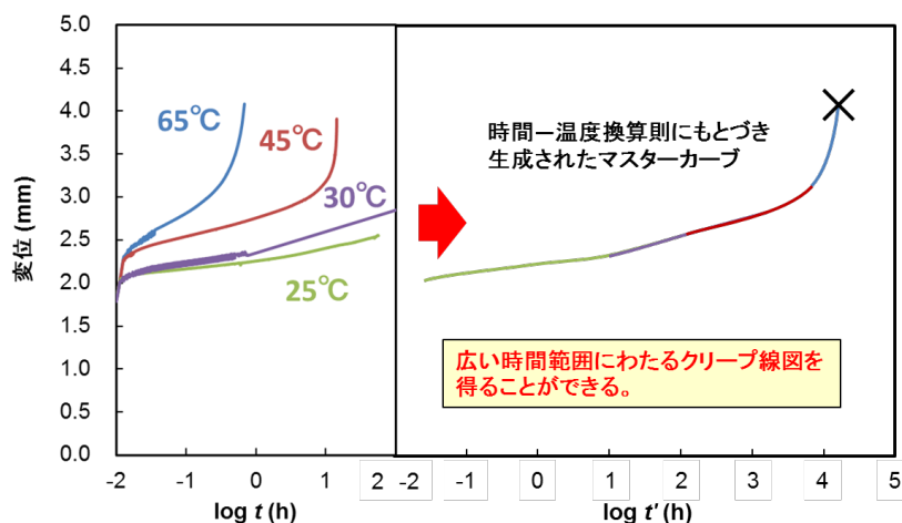
参考 図 1.2.2.5 クリープ変形曲線のマスターカーブ（最大引張荷重の 70%の負荷、基準温度 25°C）
