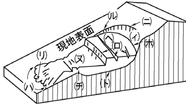
(イ) 滑落崖（主亀裂） (ロ) 二次亀裂 (ハ) 舌端部 (ニ) 冠頂部 (ホ) 頂天 (ヘ) 頭部 (ト) すべり面 (チ) 脚部 (リ) 尖端 (ヌ) 末端部 (ル) 側面
