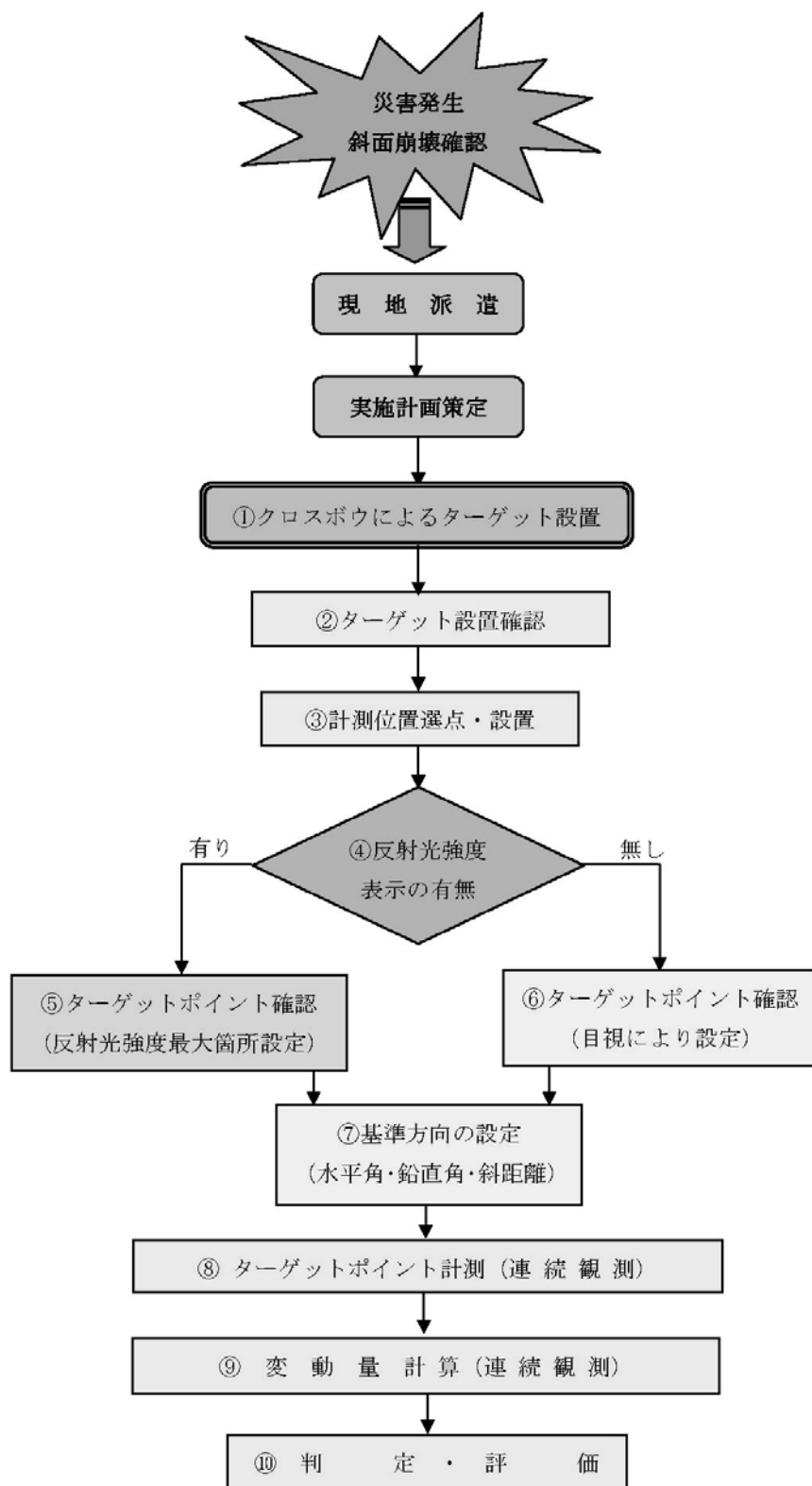
図参ー14 「RE・MO・TE2」計測フロー
