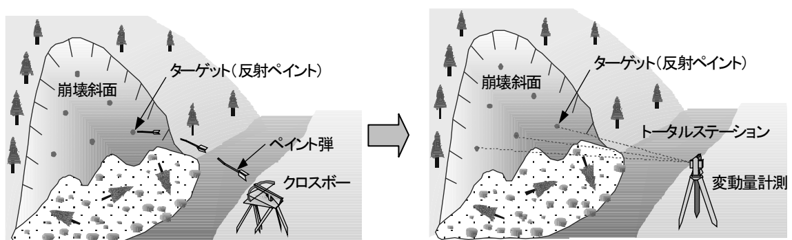
図参ー1 1 「RE・MO・TE 2 」の概要 1 2)
