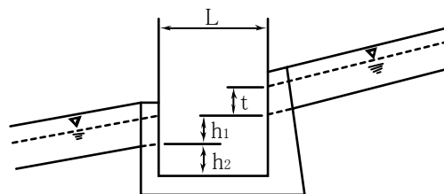
図 5 - 3 集水枳側面図
