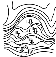
(d) 凹状多丘状地形
