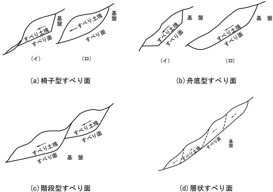
図参ー7 すべり面形状の模式図 6)
