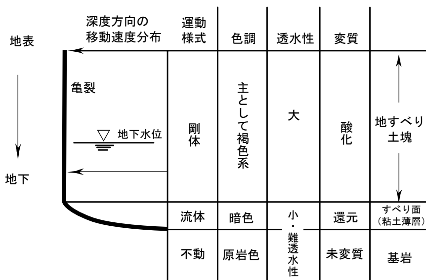
図2-7 地すべり斜面の構成 8) を一部修正
