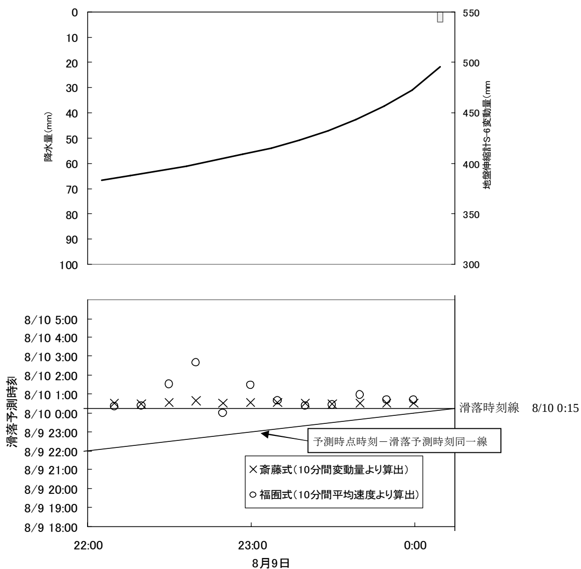
図 4 - 1 0 滑落2時間前における、斎藤式、福園式による滑落予測結果 (10分あたりの変動から予測)
