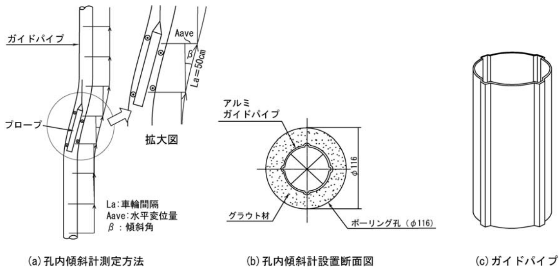
図2-10 挿入型孔内傾斜計の概要図 10) に加筆
