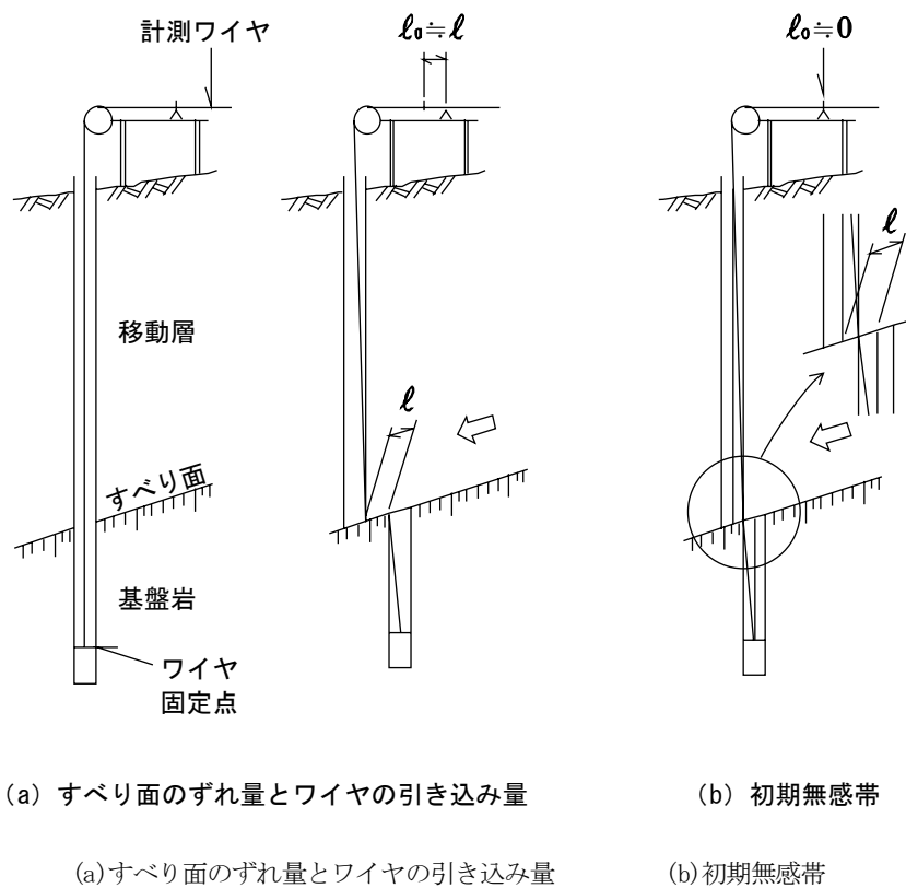
図 2-13 縦型伸縮計の概要図 10)
