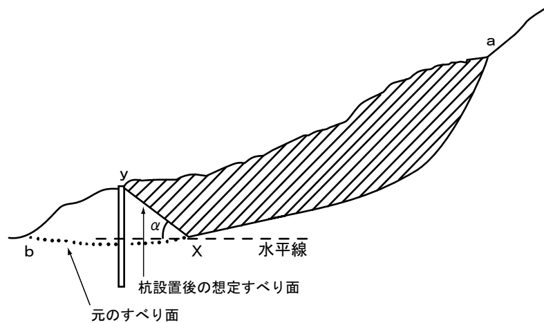
図 5-21 杭の上部の受動破壊 1)
