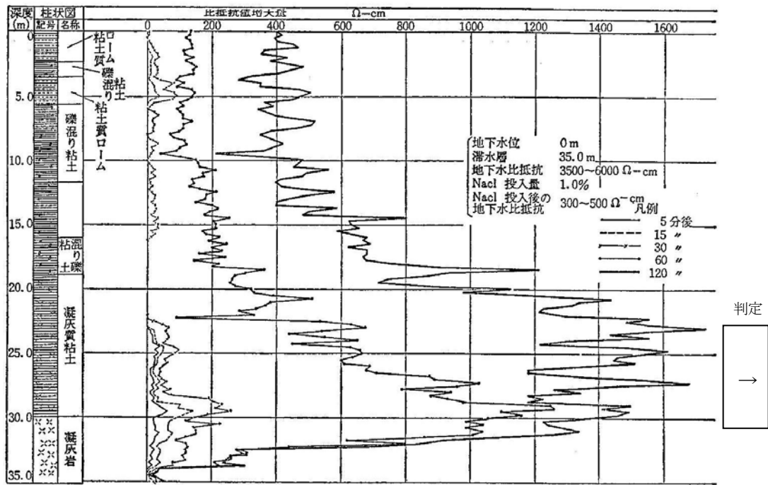
図 2-32 地下水検層測定結果 2)
