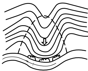
(a) 凸状尾根地形
