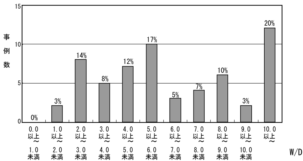
図参ー8 地すべり幅とすべり面深度との関係 8)
