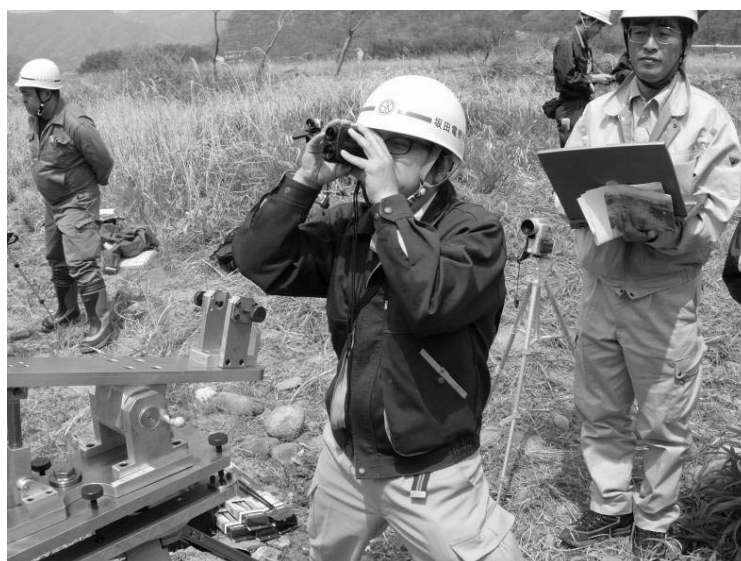
写真参－７ レーザー距離計による斜距離の計測
